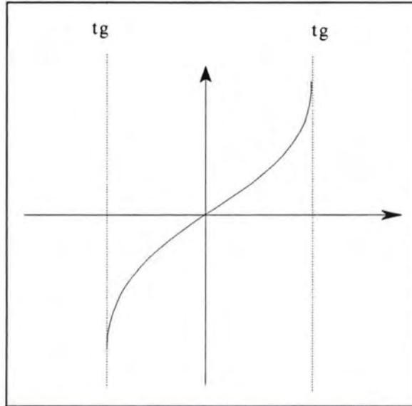
Figure C.7 : les tangentes verticales de la fonction \text{tg}
