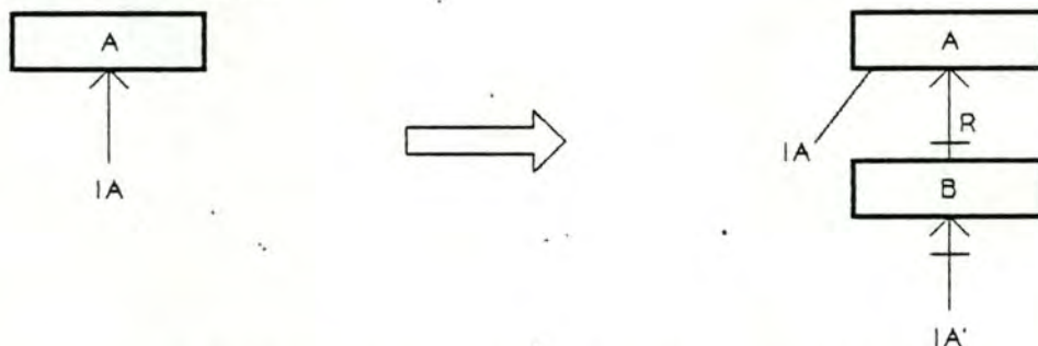
Figure 7.22: Transformation d'un accès par clé en un accès par type de chemins.
