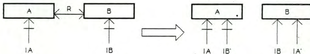
Figure 7.20: Duplication des identifiants de chaque membre de R.
