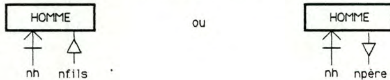
Figure 7.29: Elimination de la récursivité par duplication d'ITEMS.
