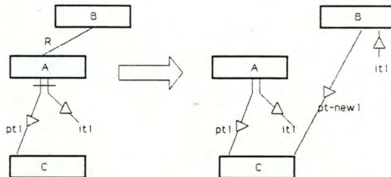
Figure 2.2: Remplacement d'un path-type par liaison de d'une de ses extrémités à l'identifiant de l'autre extrémité.
