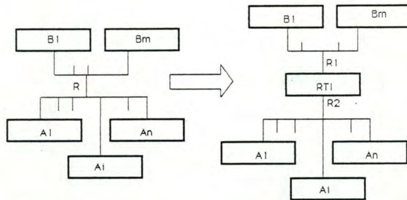
Figure 2.13: Transformation d'un path-type multitype en un record-type.
