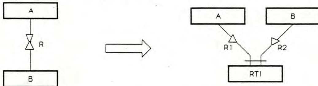
Figure 7.31: Transformation d'un type de chemins N-M en un type d'articles.
