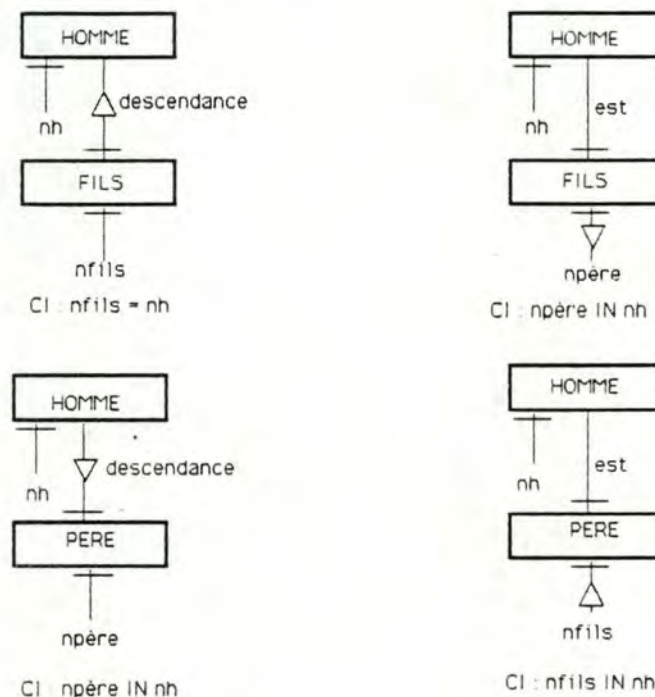
Figure 2.8: Exemple 2 de path-type récursif.
