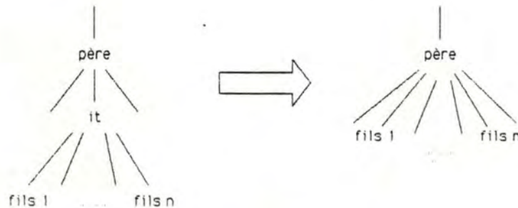
Figure 1.3: Suppression d'un niveau de décomposition d'ITEMS.
