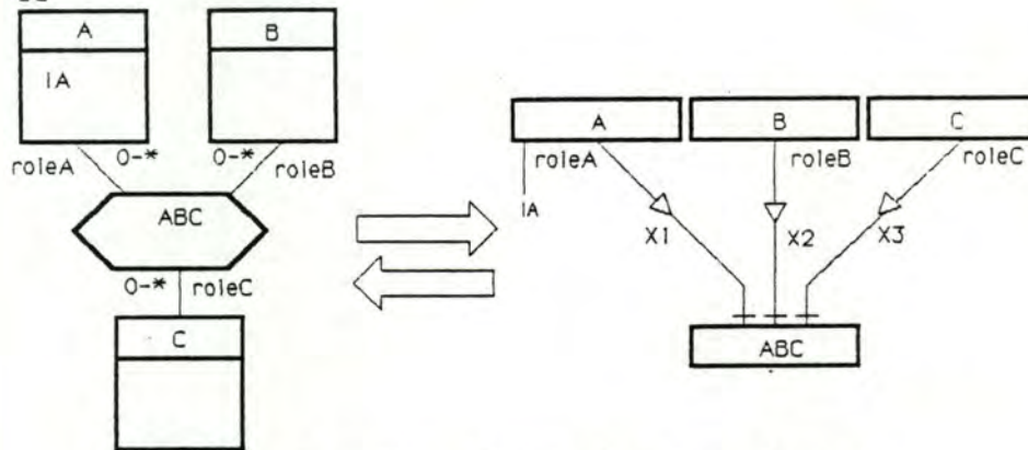
Figure 5.1: Identifiant d'un type d'entités.
