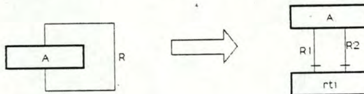
Figure 2.5: Transformation d'un PATH-TYPE récurrent en un RECORD-TYPE.
