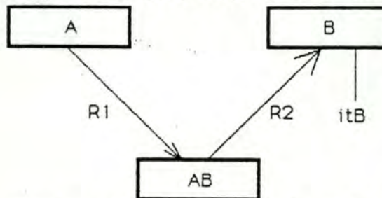
Figure 7.3: Clé d'accès dans un type de chemins transformé.
