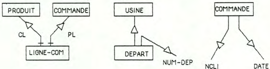
Figure 2.3: Exemple d'identifiants composés.
