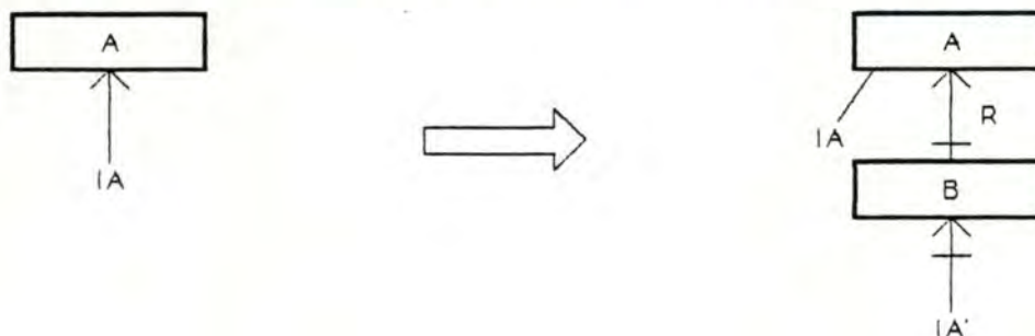
Figure 7.37: Transformation d'une clé d'accès en un type de chemins.
