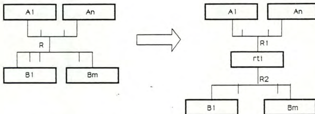
Figure 7.42: Type d'articles intermédiaire dans un multitype.
