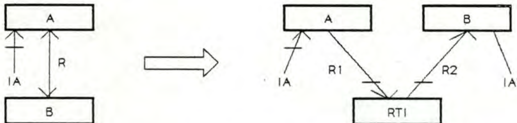
Figure 7.40: Exemple de transformation d'un type de chemins inverse.
