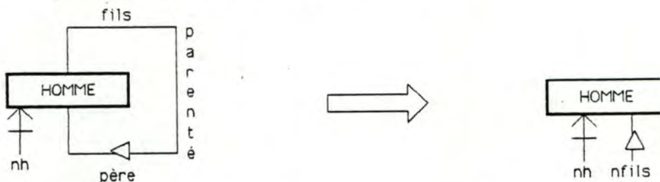
Figure 7.21: Cas d'un type de chemins récursif.
