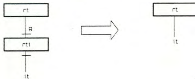
Figure 1.6: Transformation d'un RECORD-TYPE en un ITEM.
