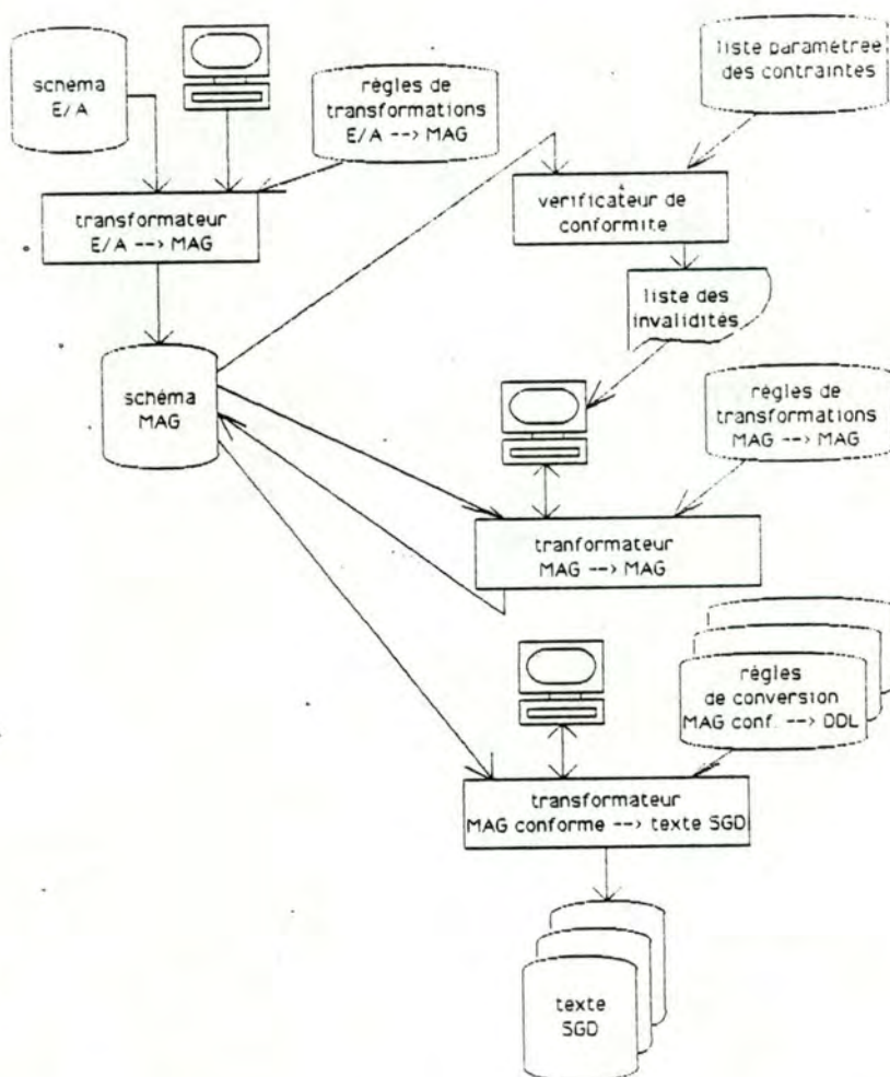
Figure : Scénario d'utilisation du transformateur de schémas.
