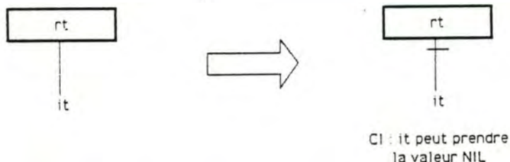
Figure 1.2: Transformations liées au caractère facultatif.
