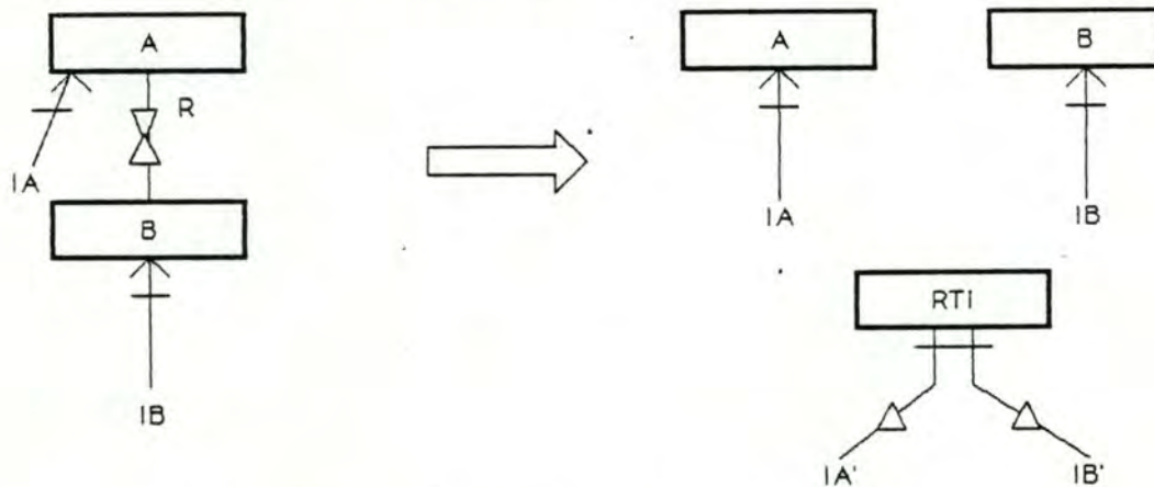
Figure 7.26: Macro-transformation : cas d'un type de chemins N-M.
