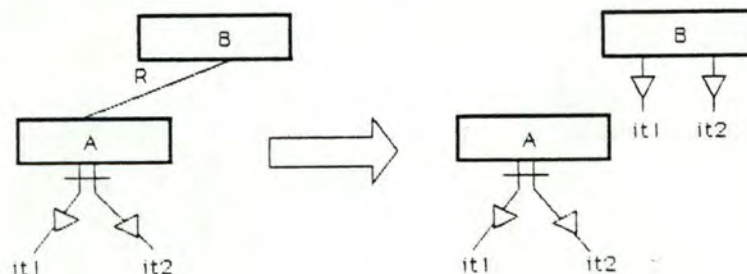
Figure 2.1: Elimination d'un path-type par duplication d'items.
