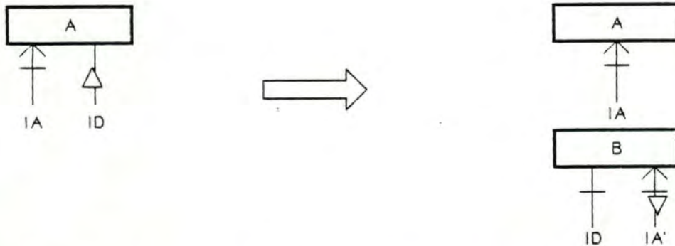
Figure 7.25: Elimination de la répétitivité sans créer un type de chemins.
