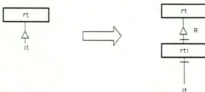
Figure 1.1: Elimination de la répétitivité par création d'un record-type intermédiaire.
