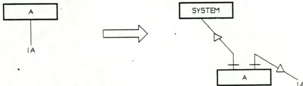
Figure 7.33: Le type d'articles SYSTEM comme support d'un identifiant.
