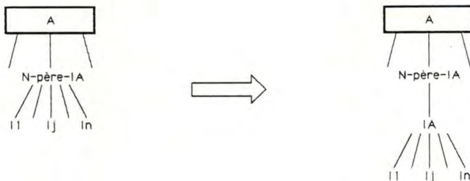
Figure 7.14: Regroupement d'ITEMS en un ITEM décomposable.
