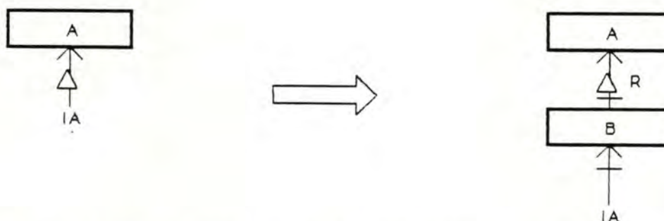
Figure 7.38: Remplacement d'une clé d'accès répétitive en types d'articles.
