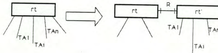
Figure 3.1: Eclatement d'un RECORD-TYPE en deux.
