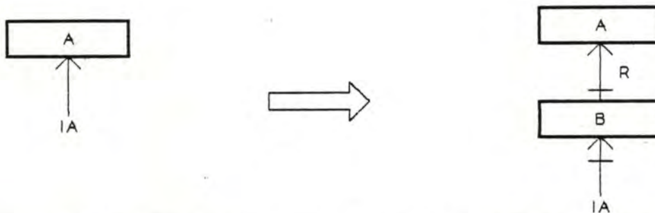
Figure 7.36: Transformation d'un ITEM clé d'accès en un type d'articles.
