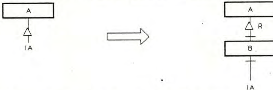
Figure 7.24: Transformation d'un ITEM répétitif en un type d'articles.
