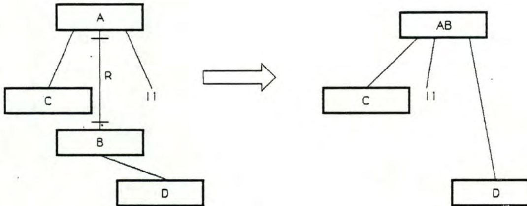
Figure 7.32: Fusion de deux types d'articles de même sémantique.
