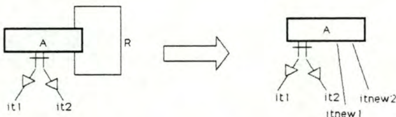
Figure 2.6: Elimination d'un PATH-TYPE récursif par duplication d'ITEMS.
