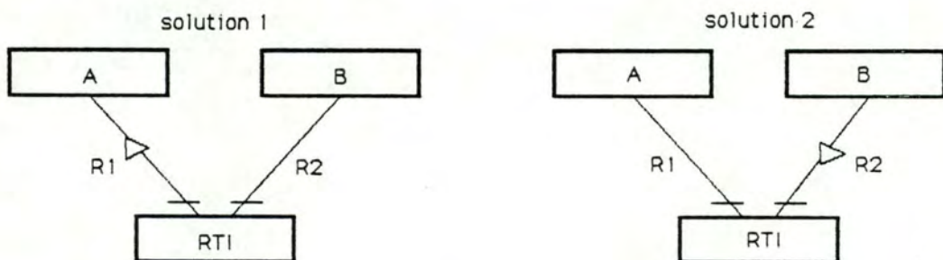
Figure 7.16: Cas d'un type de chemins 1-N.
