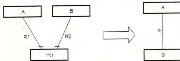
Figure 2.4: Transformation d'un record-type en un path-type.
