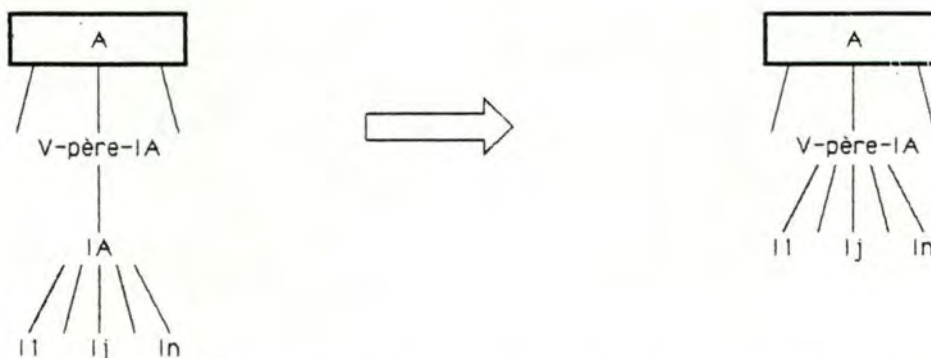
Figure 7.13: Aplatissement d'un ITEM décomposable.
