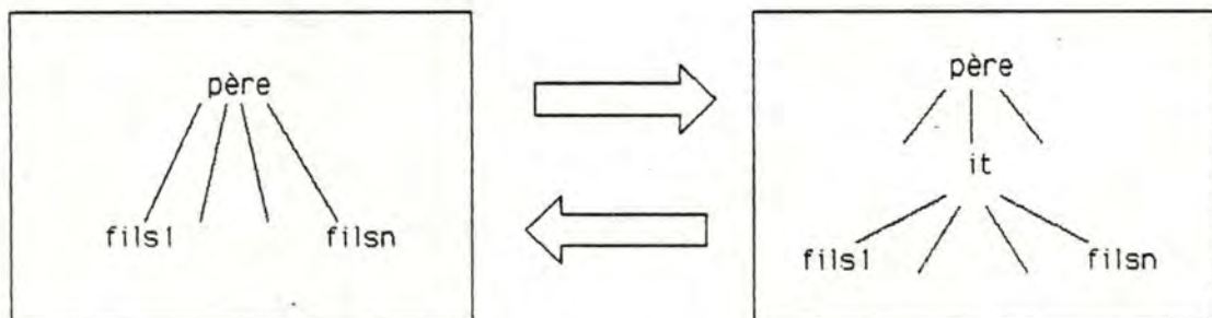
Figure 7.7: Regroupement/décomposition d'ITEMS.
