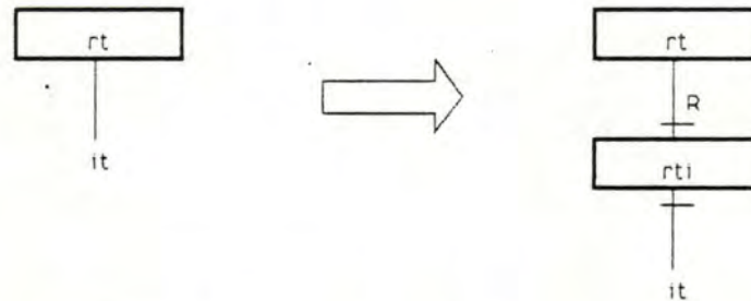
Figure 1.5: Transformation d'un item en un record-type.
