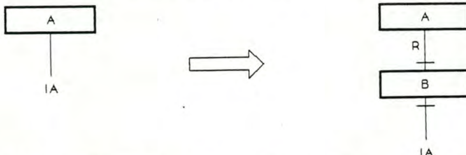
Figure 7.34: Transformation d'un ITEM identifiant en un type d'articles.
