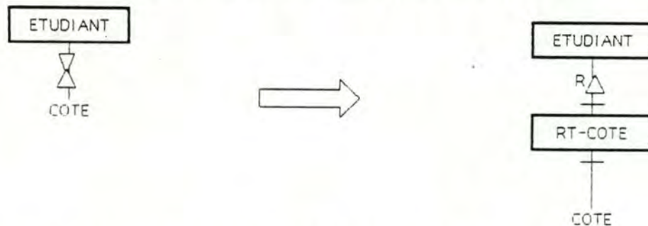
Figure 7.12: Cas d'un ITEM répétitif à valeurs éventuellement doubles
