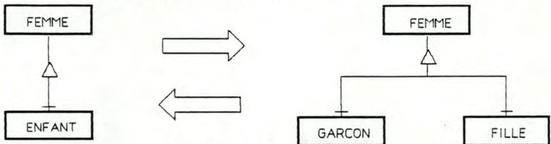
Figure 7.9: Exemple d'éclatement/fusion de types d'articles.
