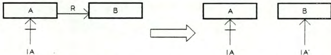
Figure 7.19: Cas où R ne sert d'accès que de A vers B.
