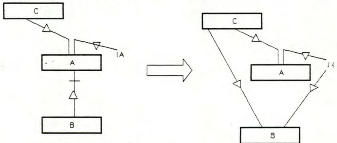
Figure 7.44: Liaison d'une extrémité à l'identifiant de l'autre.
