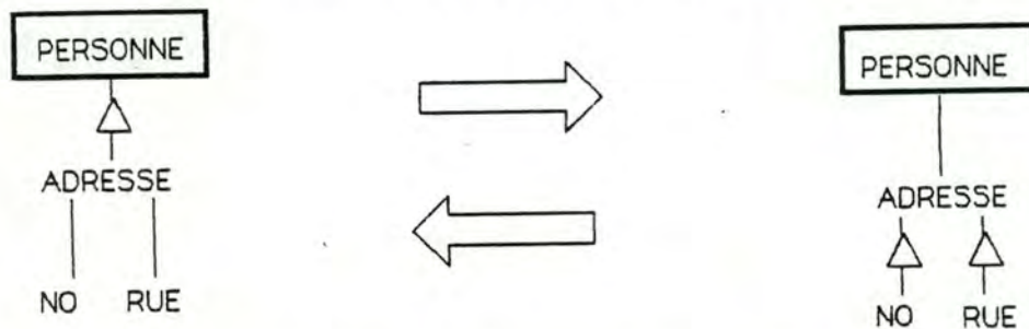
Figure 7.10: Exemple de report de répétitivité.
