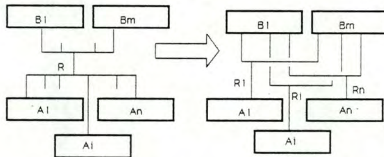
Figure 2.12: Elimination du multitype dans l'une des extrémités.
