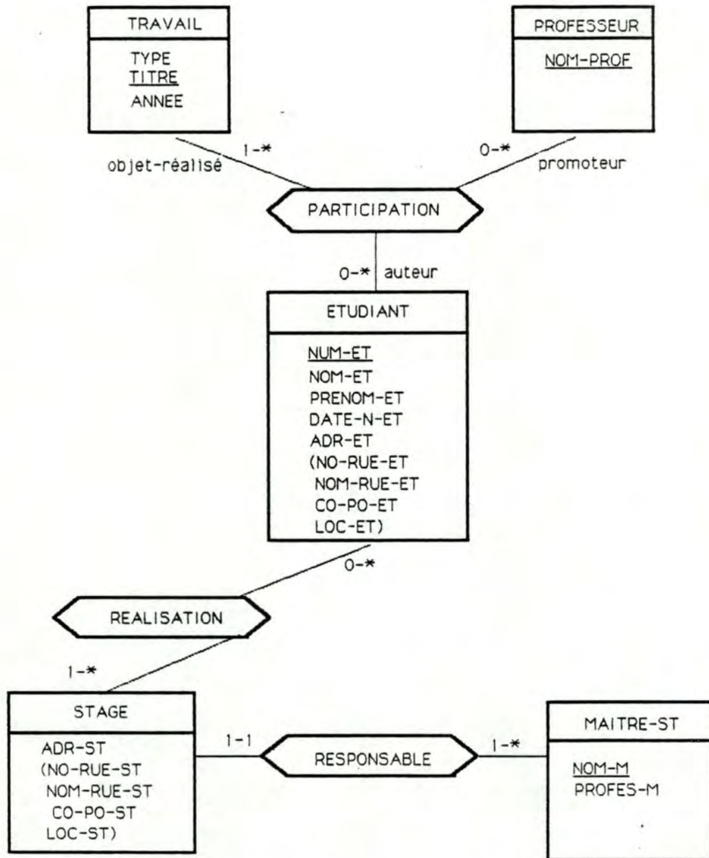
Figure 0.1: Schéma conceptuel des données.
