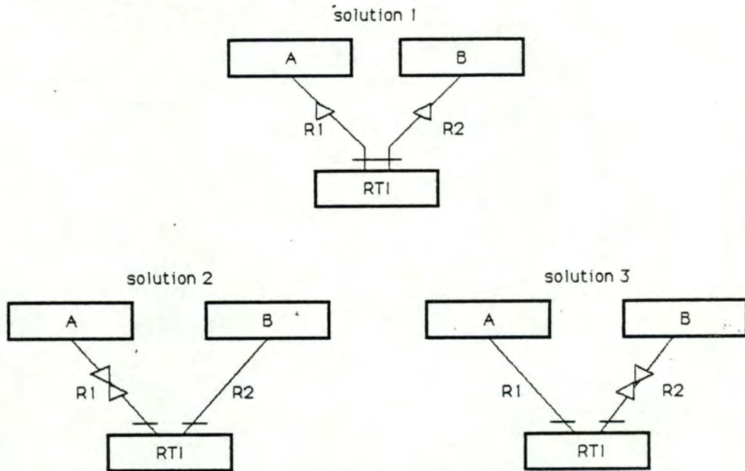
Figure 7.15: Cas d'un type de chemins N-M.
