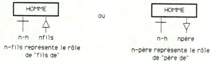
Figure 2.7: Exemple 1 de path-type récursif.
