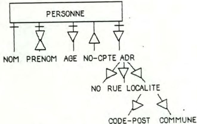
Figure 2.1: Exemple d'ITEMs.
