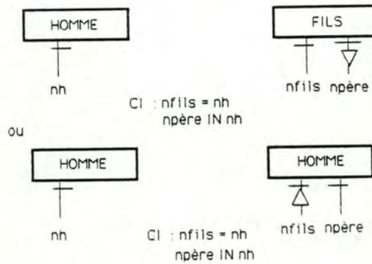
Figure 2.9: Exemple 3 de path-type récursif.
