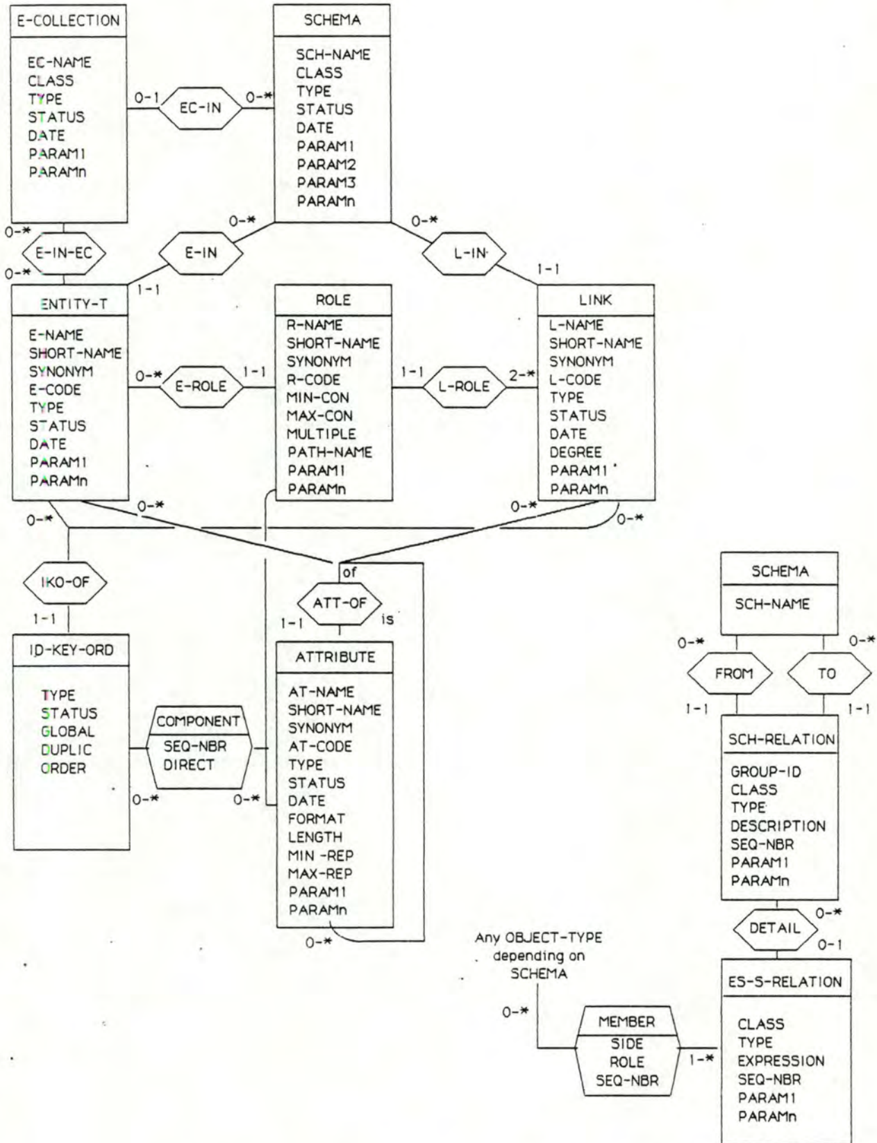
Figure 11.1: Sous-schéma de la BD des spécifications.
