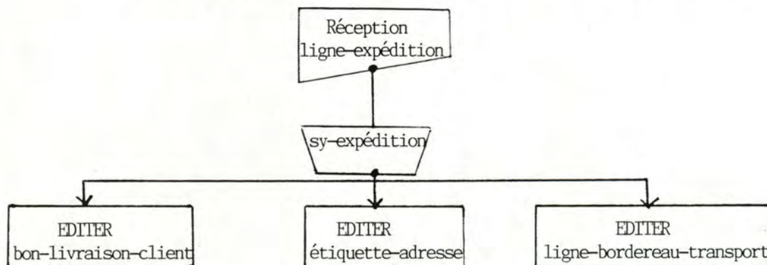
figure 3.11. Modèle dynamique de la phase FACTURATION.
