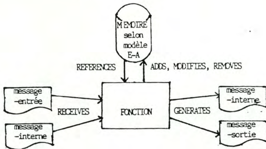
figure 3.17. Modèle statique d'une fonction.
