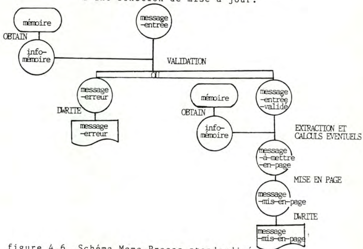
figure 4.5. Schéma Memo-Proges standardisé d'une fonction de mise à jour.
