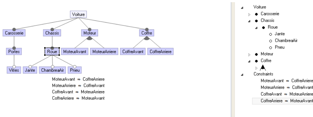
Figure A.1: Graphe généré par Feature IDE
