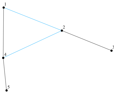
Figure 3.3: Parcours
