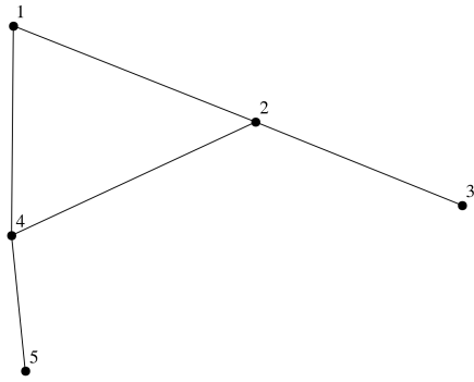
Figure 3.1: Graphe non-orienté
