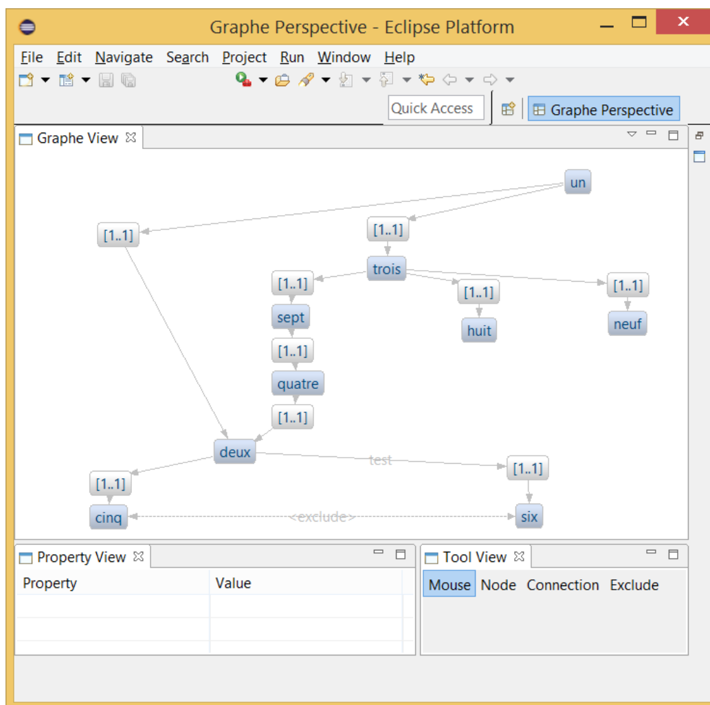
Figure 6.3: Capture d'écran du prototype
