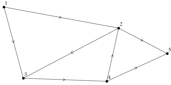
Figure 3.2: Graphe orienté
