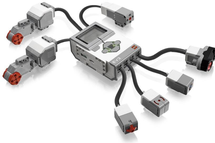
Figure 8 : Capteurs et actuateurs connectés à une brique Lego Mindstorms EV3
