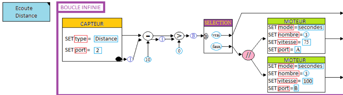
Figure 32 : Cas d'étude n°1 Exemple visuel (partie 3/3)
