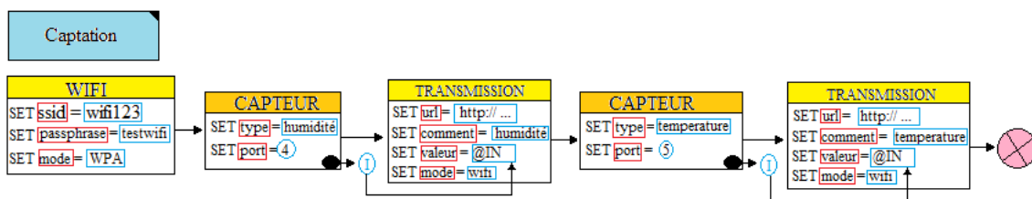
Figure 37 : Cas d'étude n°2 Exemple visuel (partie 4/4)
