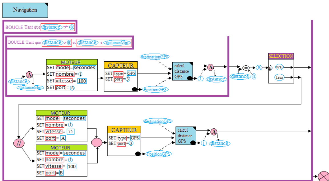
Figure 36 : Cas d'étude n°2 Exemple visuel (partie 3/4)
