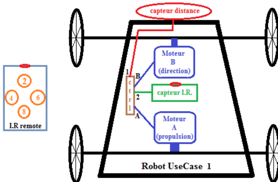
Figure 29 : Schéma du prototype de l'étude de cas n°1
