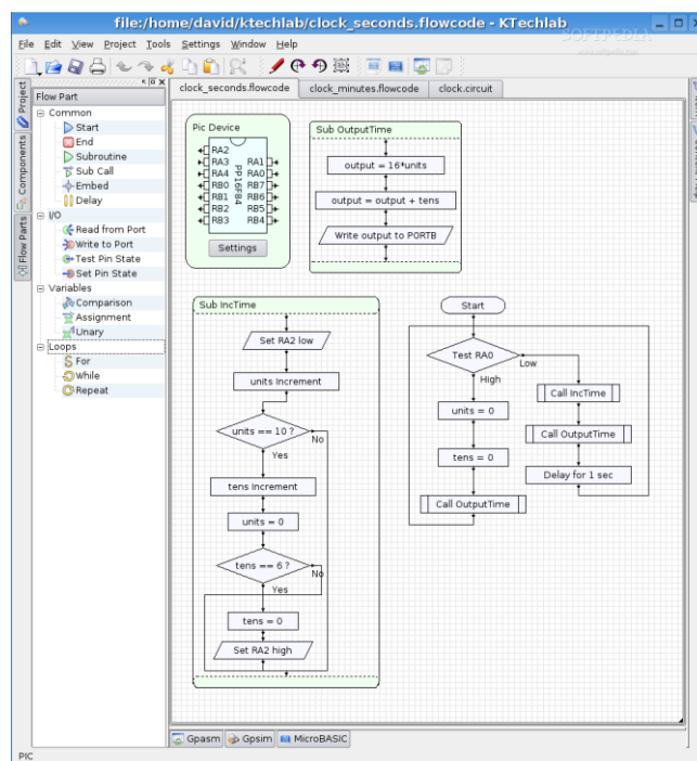
Figure 23 : Environnement / langage de développement KTechLab
