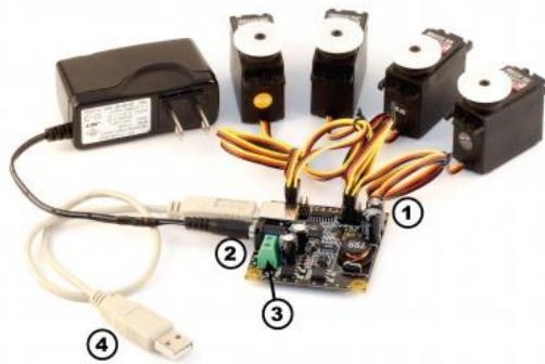
Figure 5 : carte Phidget avec plusieurs servomoteurs connectés
