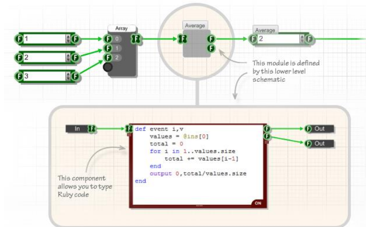
Figure 16 : Langage de programmation Flowstone (Exemple n°2)
