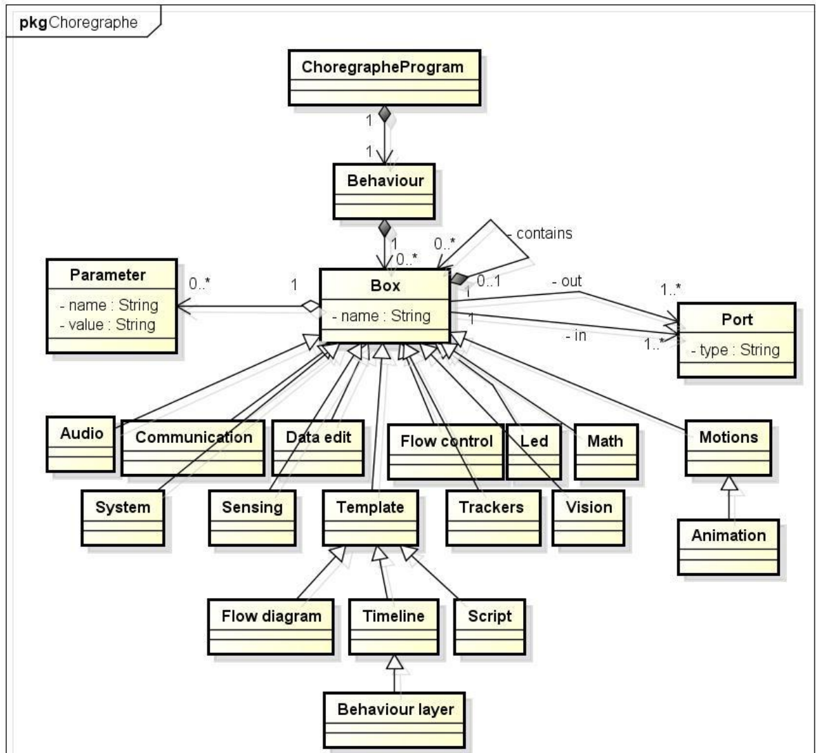
Figure 28 : Métamodèle du langage Choregraphe
