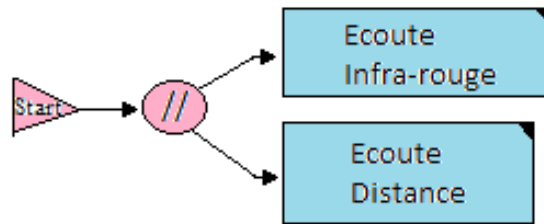
Figure 30 : Cas d'étude n°1 Exemple visuel (partie 1/3)
