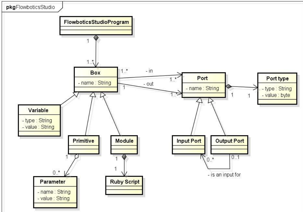
Figure 27 : Métamodèle du langage Flowstone de Flowbotics studio
