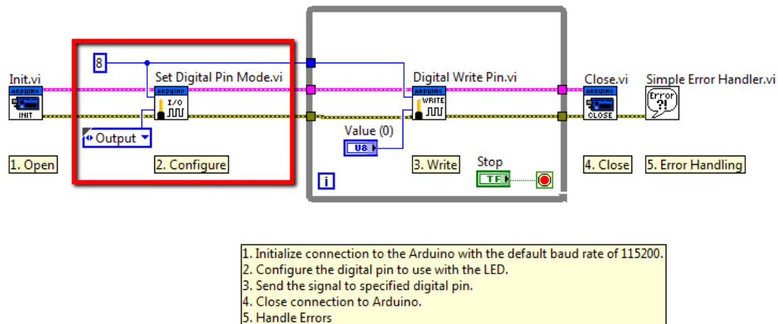
Figure 19 : Langage « G » dans LabView
