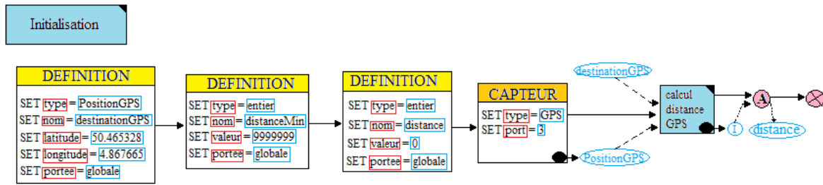
Figure 35 : Cas d'étude n°2 Exemple visuel (partie 2/4)
