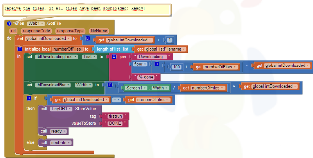
Figure 20 : Environnement / langage de développement App Inventor (exemple n°1)
