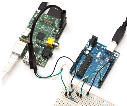
Figure 2 : Exemple de projet avec Raspberry Pi, Arduino et une breadboard
