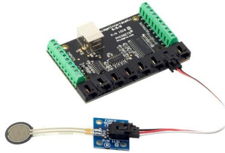
Figure 4 : Phidget capteur de force connecté à une carte Interface Kit (Bridge)
