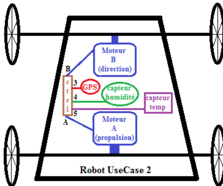
Figure 33 : Schéma du prototype de l'étude de cas n°2
