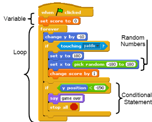
Figure 12 : langage de développement Scratch
