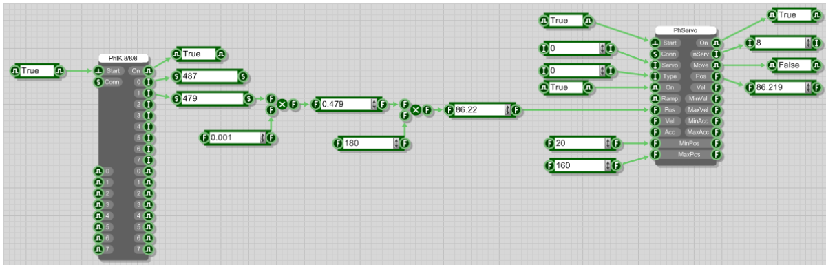
Figure 15 : Langage de programmation Flowstone (Exemple n°1)
