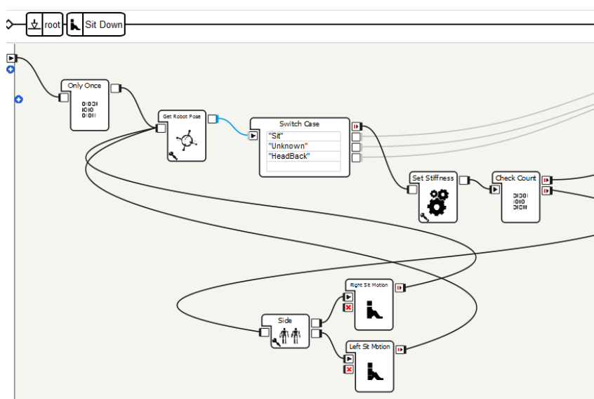
Figure 18 : Environnement / langage de développement Choregraphe (exemple n°2)
