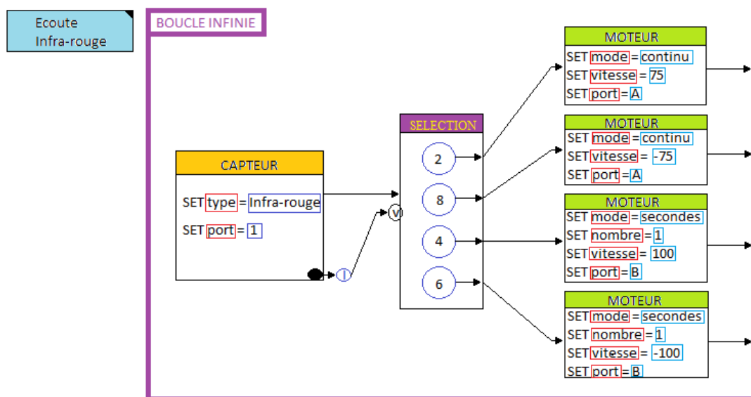
Figure 31 : Cas d'étude n°1 Exemple visuel (partie 2/3)
