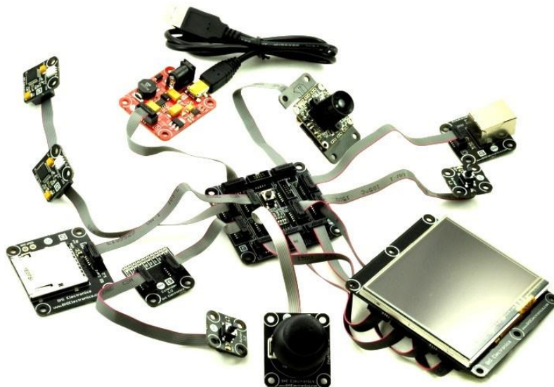
Figure 10 : Composants .Net Gadgeteer connectés à une carte GHI Fez Spider board
