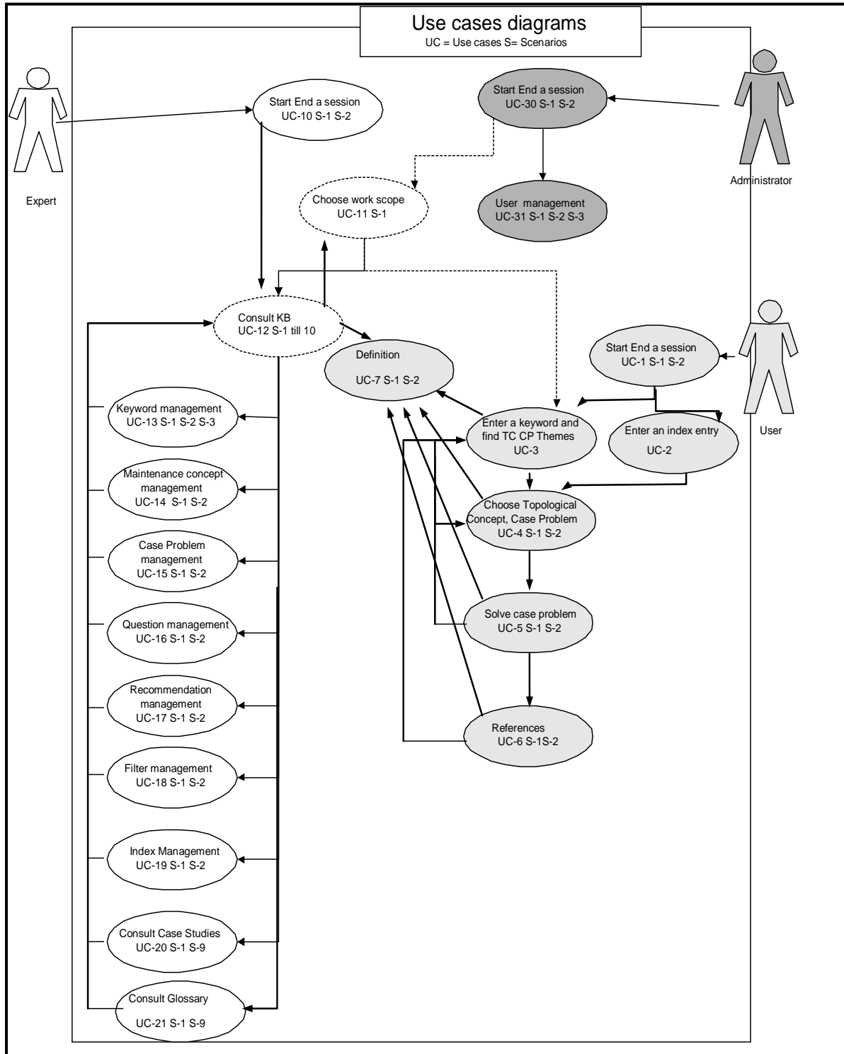
Figure 1 : Diagramme des cas d'utilisation.
