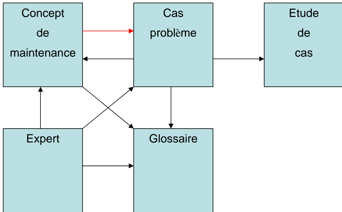
Figure 4.3 : Liens entre les différents types de fichiers de la base de connaissance
