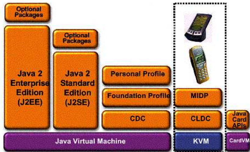
FIG. 5.4 – L'architecture de la J2ME
