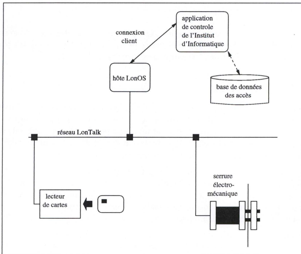
FIG. 6.1 – Une partie de l'application.
