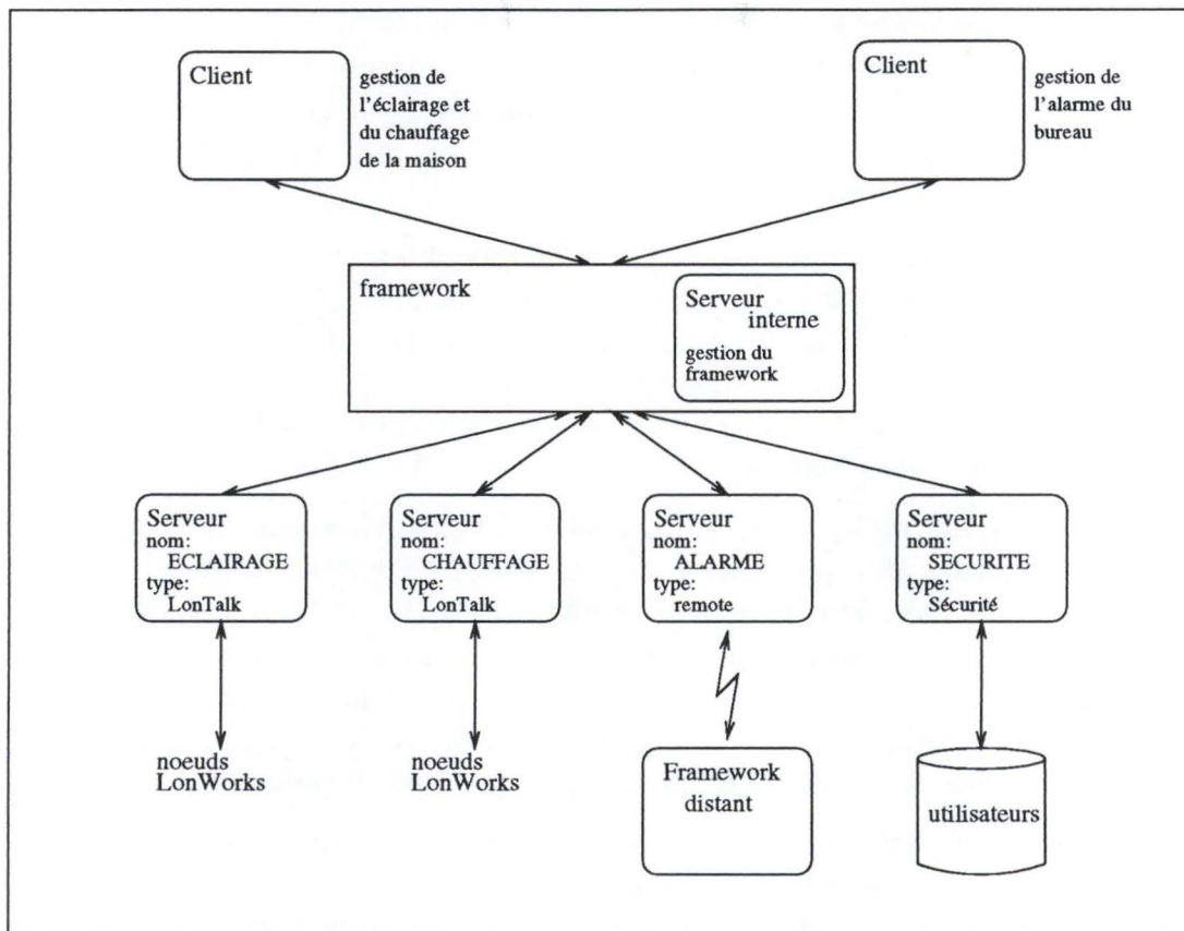
FIG. 4.2 – Un exemple de configuration typique
