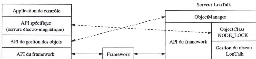
FIG. 6.2 – Intégration des différents développements relatifs au matériel.
