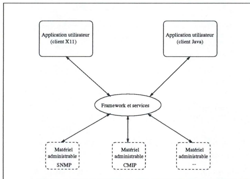
FIG. 1.9 – Schéma général de la suite logicielle OPENMASTER.
