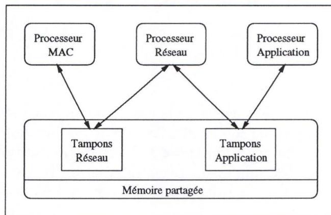
FIG. 1.5 – Communication entre les processeurs d'un Neuron Chip.
