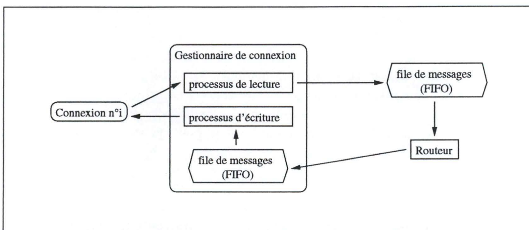
FIG. 4.6 – Détail d'un gestionnaire de connexion.
