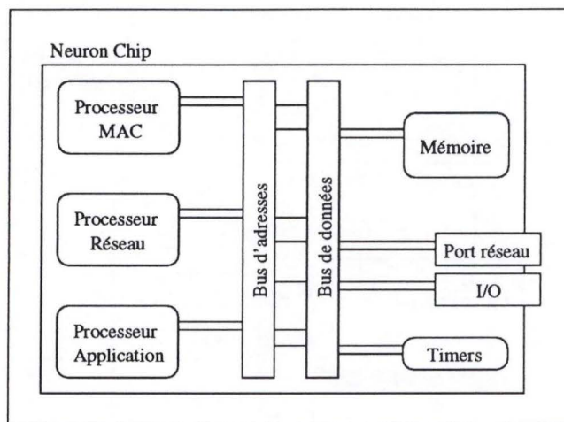
FIG. 1.4 – Synoptique d'un Neuron Chip.
