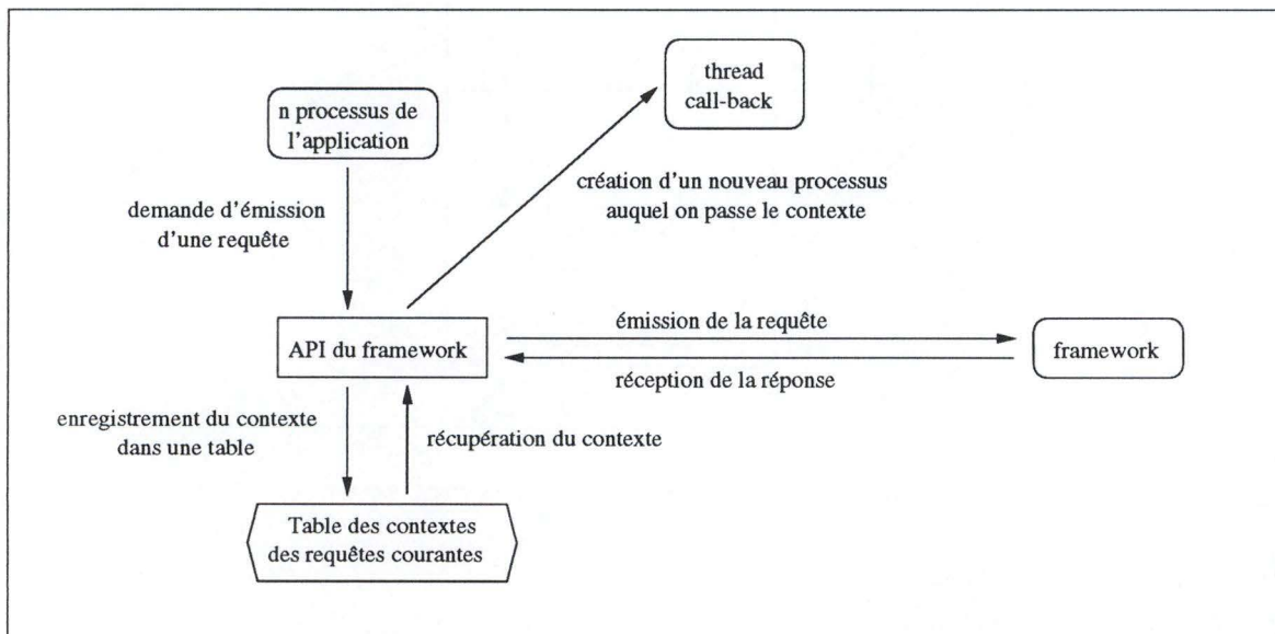
FIG. 5.4 – Première solution asynchrone.
