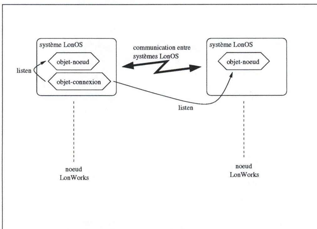
FIG. 3.12 – Connexions virtuelles.
