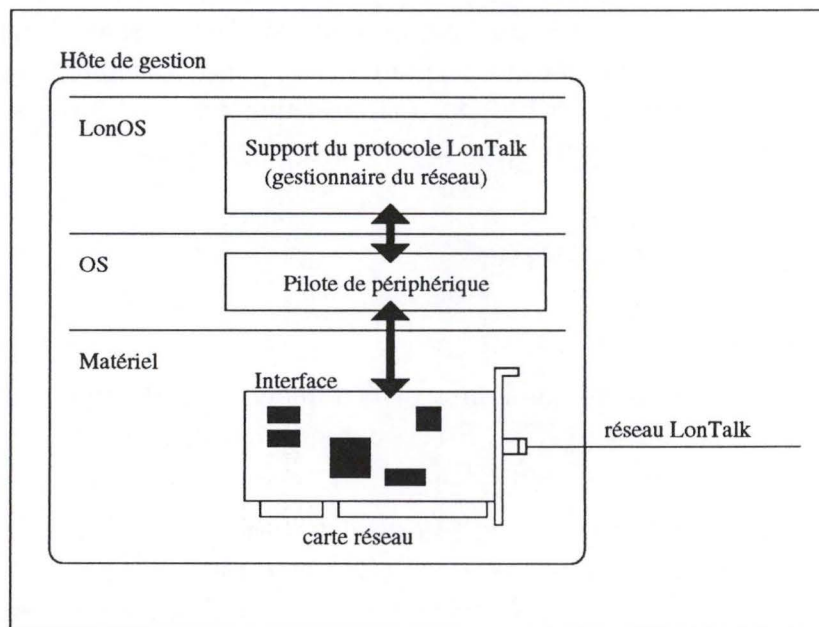
FIG. 2.1 – Hôte de gestion répondant aux besoins minimums.
