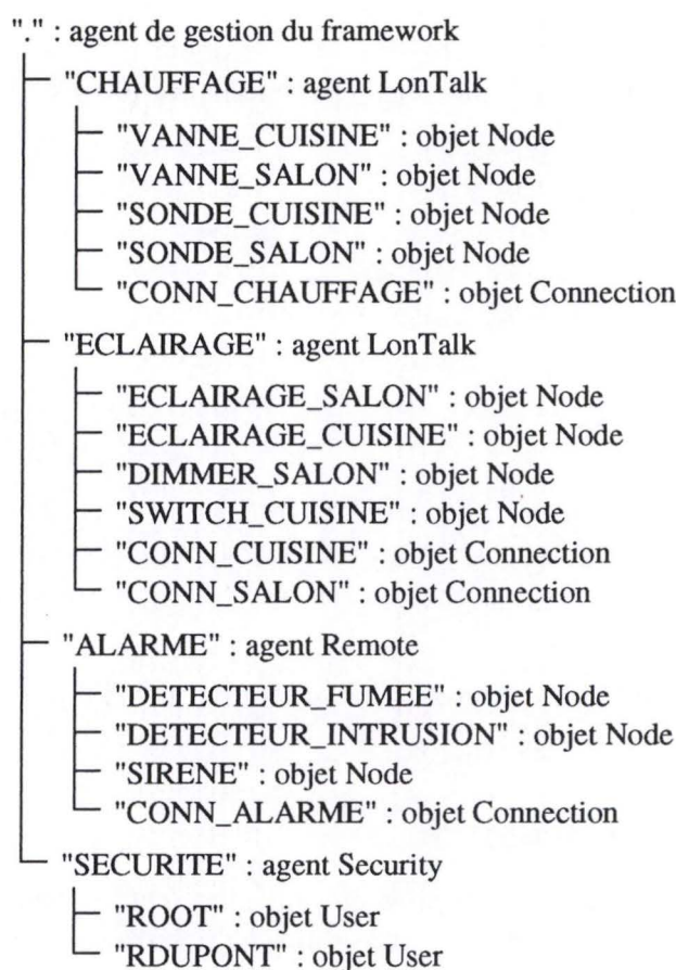
FIG. 4.8 – Arborescence des serveurs et objets enregistrés.
