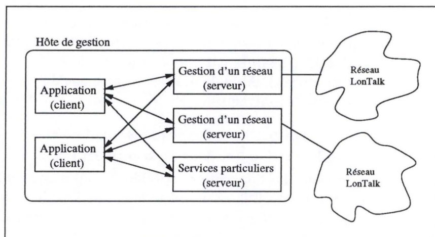
FIG. 2.2 – Multi-clients et multiples serveurs.
