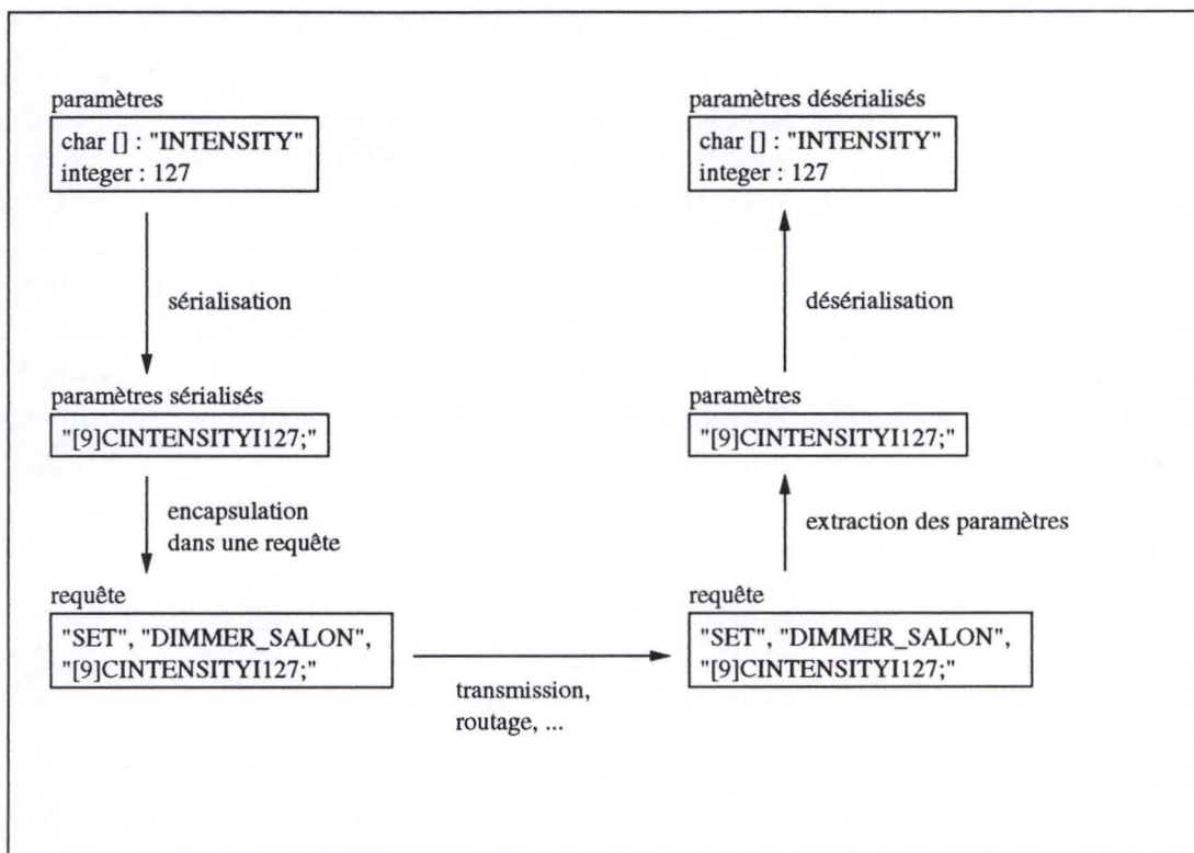
FIG. 4.4 – Serialisation et désérialisation de paramètres.
