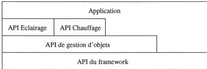
FIG. 5.1 – Exemple d'empilement des couches.
