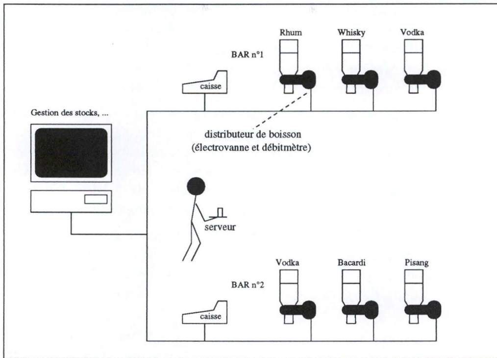
FIG. 1.2 – Contrôle de discothèques
