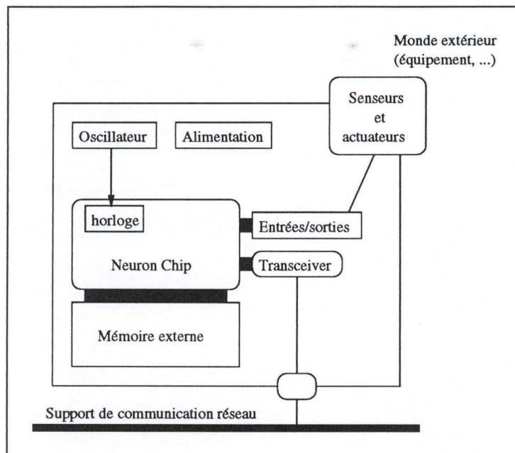
FIG. 1.3 – Schéma d'un noeud typique.
