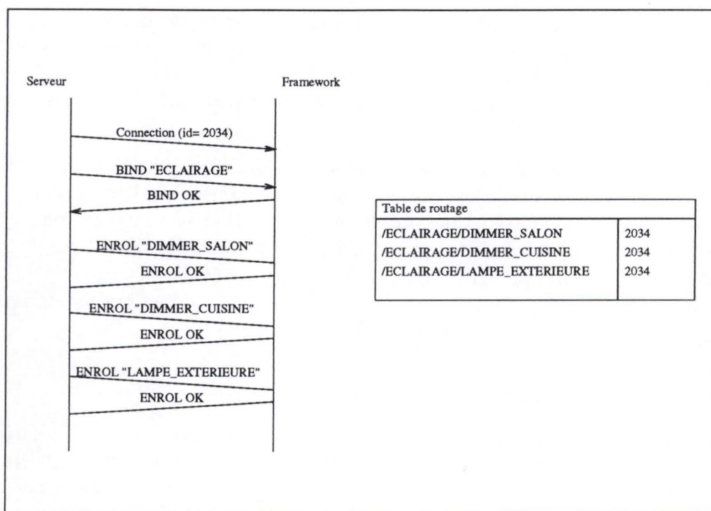
FIG. 4.3 – Exemple de démarrage d'un serveur: "bind et enrols"
