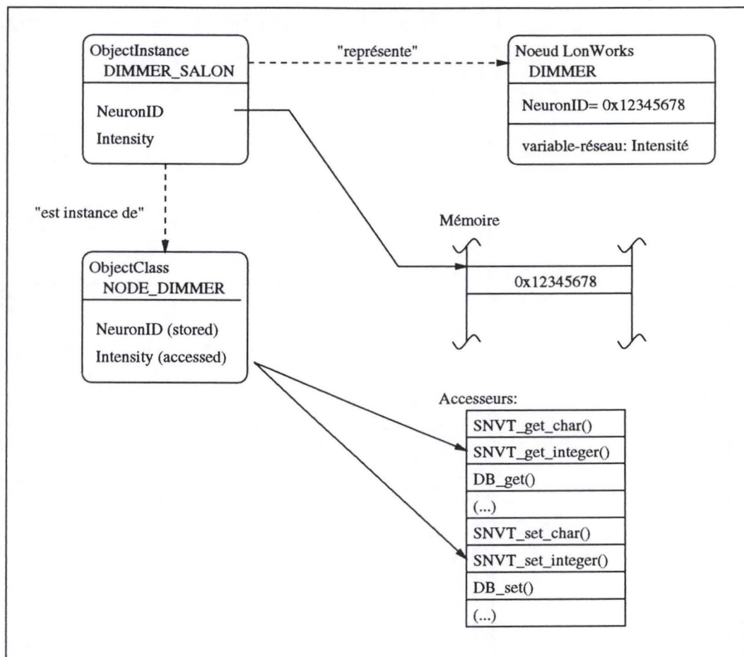
FIG. 3.7 – Variables-réseau dans la représentation d'un noeud LonWorks.
