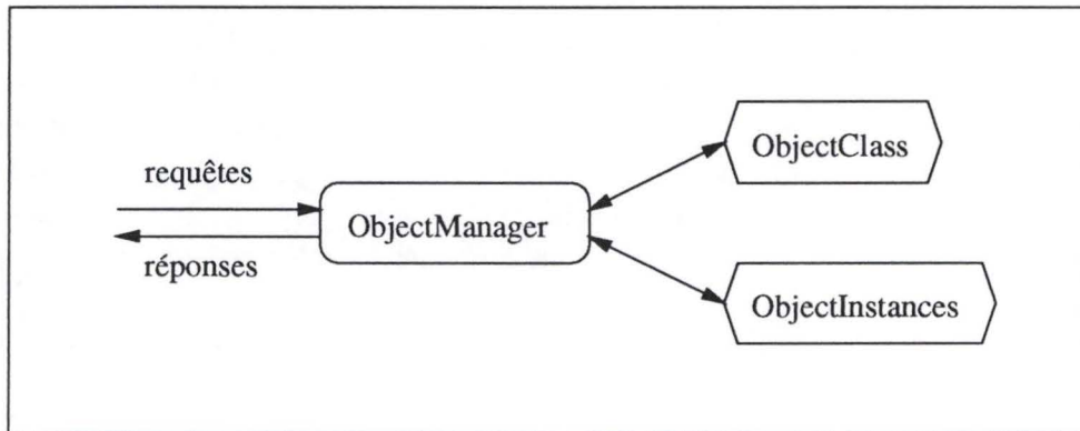
FIG. 3.13 – L' ObjectManager .
