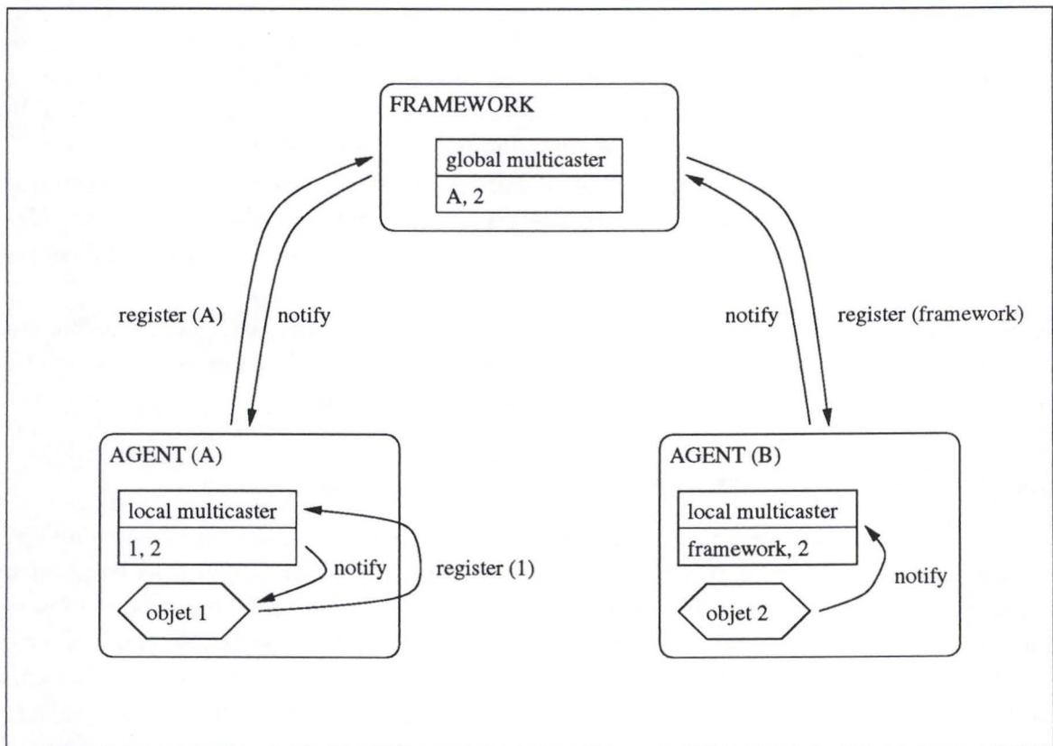
FIG. 3.11 – Communication entre objets distants.
