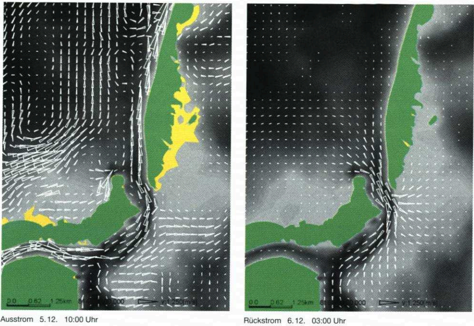
Abb. 13: Typische Strömungssituationen am 5./6. 12. 1997
