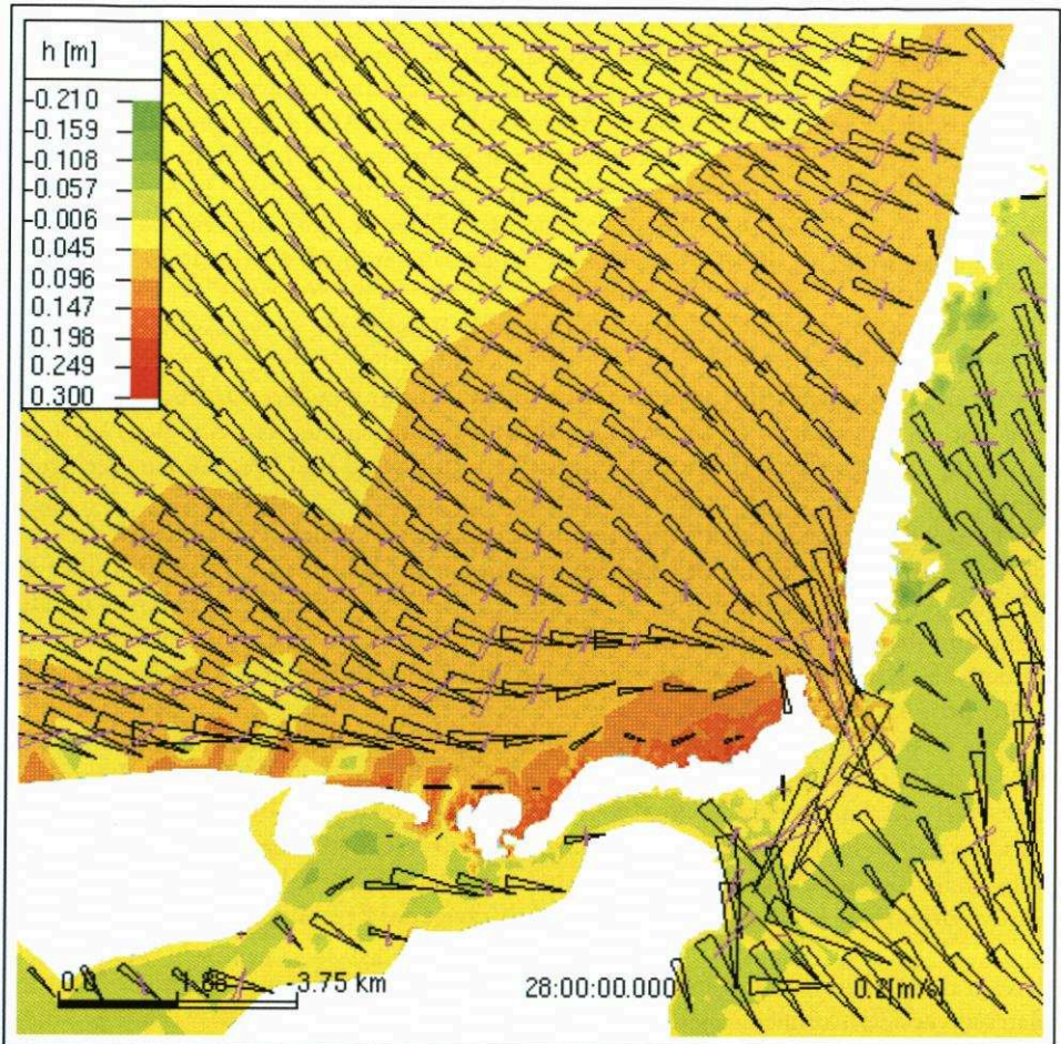
Abb. 10: Dreidimensionales Strömungsfeld in der Gellenbucht
