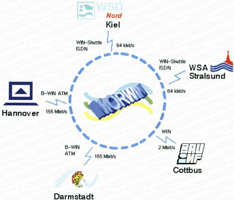
Abb. 8: MorWin-Projektpartner im Internet
