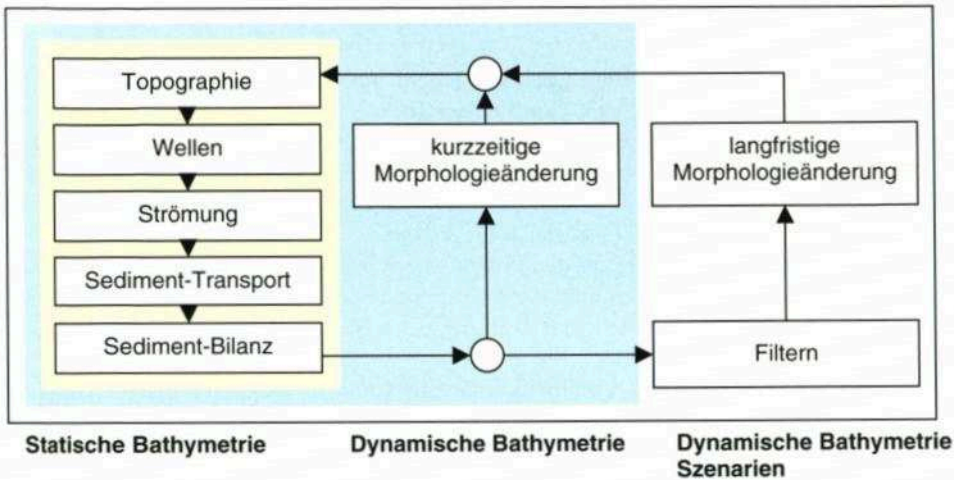
Abb. 7: Prinzip morphodynamischer Simulationen
