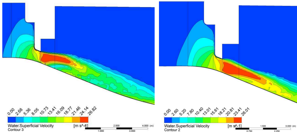
Abbildung 7: Geschwindigkeiten in der Mittelachse linkses Schütz im Fall \text{BHQ}_1 , Variante 3.01 (links) und Variante 3.02 (rechts)
