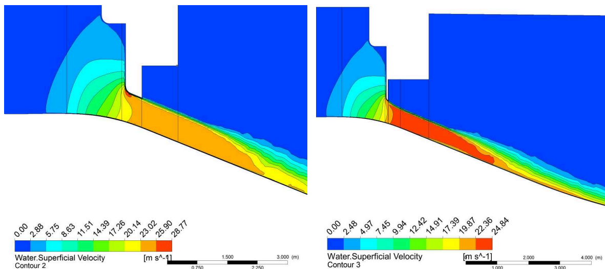
Abbildung 8: Geschwindigkeiten in der Mittelachse linkses Schütz im Fall \text{BHQ}_1 , Variante 3.03 (links) und Variante 3.04 (rechts)
