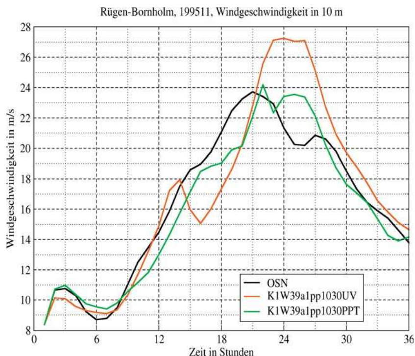
Abb. 9: Zeitreihe der Windgeschwindigkeit am Wassergitterpunkt zwischen Rügen und Bornholm. Simulation mit dem COSMO-CLM, ohne Spectral Nudging (OSN – schwarze Linie), maximales Spectral Nudging des Horizontalwindes (rote Linie), maximales Spectral Nudging des Luftdrucks und der Temperatur (grüne Linie)
