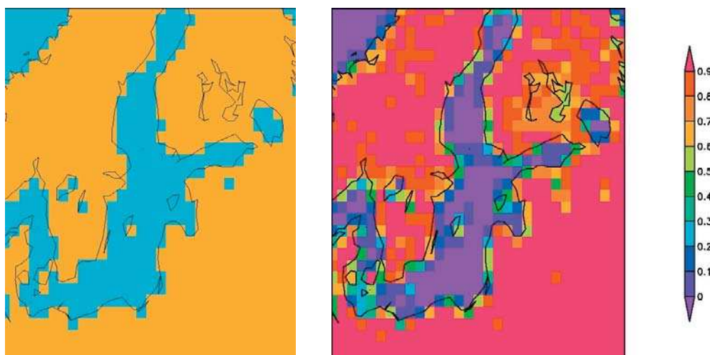
Abb. 1: Land-See-Maske (links) und fraktioneller Landanteil (rechts) des COSMO-CLM in der 0,44°-Version im Ostseeraum
