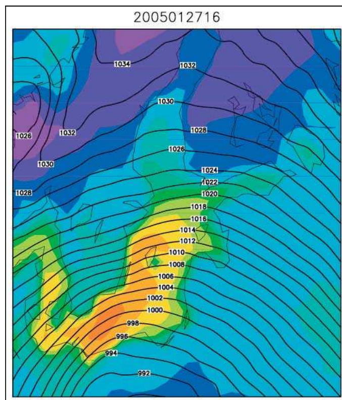
Abb. 11: COSMO-CLM-Simulation einer Sturmflutsituation an der deutschen Ostseeküste. Antriebsdatensatz: Extremer Member der EPS-Simulation zur Sturmflut am 27.1.2005
