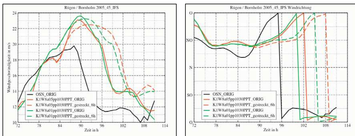
Abb. 12: Windgeschwindigkeit und -richtung aus der COSMO-CLM-Simulation einer Sturmflut-situation an der deutschen Ostseeküste. Antriebsdatensatz: Extremes Mitglied der EPS-Simulation zur Sturmflut am 27.1.2005. Schwarze Linie: Simulation ohne Spectral Nudging; rote Linie: Spectral Nudging mit Luftdruck und Temperatur mit Wellenzahl 8, Gewichtung 0,5; grüne Linie: Spectral Nudging mit Luftdruck und Temperatur mit Wellenzahl 8, Gewichtung 0,1; gestrichelt (rot und grün): Antriebsdaten aus dem EPS um 6 Stunden gestreckt in das COSMO-CLM eingelesen
