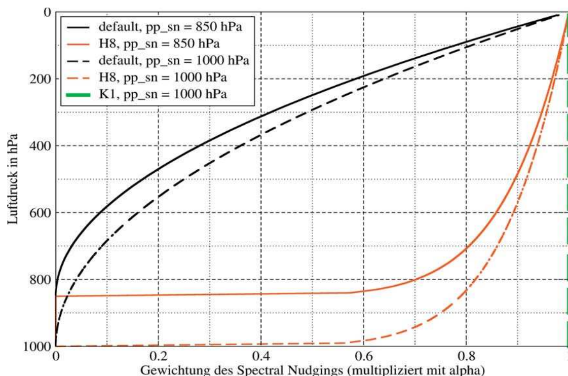
Abb. 2: Höhenabhängige Gewichtung des Spectral Nudgings im COSMO-CLM. Die schwarze Kurve zeigt den im Standard-Modell-Quellcode vorgegebenen Verlauf. Die roten Linien stehen für einen versuchsmäßig veränderten Verlauf (H8), die grüne Linie zeigt die Gewichtung 1 an (Versuchskonfiguration K1, mit K1 für Konstant Eins). Die Unterscheidung in die durchgezogene und die gestrichelte-Linie stellt sich wie folgt dar: durchgezogene Linie: Spectral Nudging ist wirksam oberhalb von 850 hPa (ca. 1,5 km Höhe), gestrichelte Linie: Spectral Nudging ist wirksam bis zum Boden
