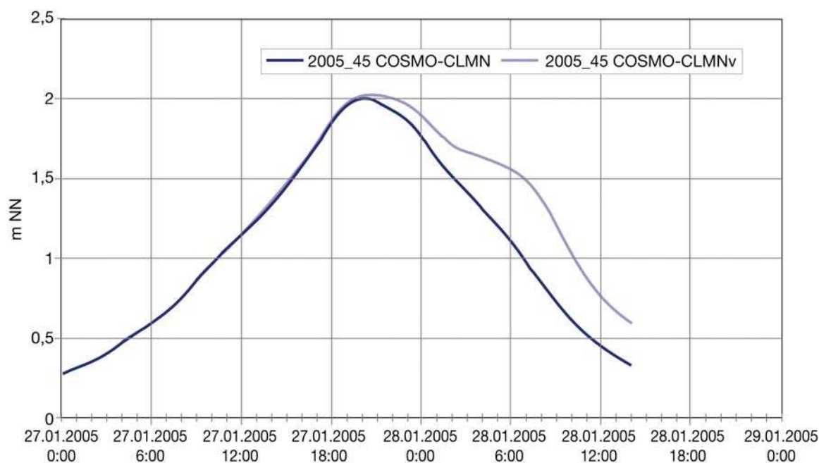
Abb. 13: Zeitlicher Verlauf des simulierten Wasserstands am Pegel Wismar. Blaue Linie: Wasserstandsmodell angetrieben mit COSMO-CLM unmodifiziert; rote Linie: Wasserstandsmodell angetrieben mit COSMO-CLM mit seinerseits verlangsamten Antrieb (analog zu den grünen Linien aus Abb. 12). Wasserstandsrechnung und Erstellung der Abbildung: BORK (2008)
