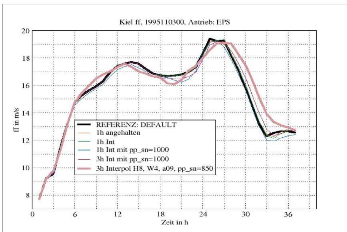
Abb. 6: Zeitreihe der simulierten Windgeschwindigkeit (ff) am Gitterpunkt „Kieler Bucht“ des COSMO-CLM. Antriebsdaten: Extremer EPS-Member für Sturmflut am 3.11.1995. Dicke schwarze Linie: zeitlicher Verlauf für den Fall der Verwendung von unveränderten Antriebsdaten, zudem COSMO-CLM-Lauf mit Standardeinstellung des Spectral Nudging; rote Linie: COSMO-CLM-Lauf mit Standardeinstellung des Spectral Nudging, Antriebsdaten für eine Stunde konstant gehalten, danach um eine Stunde versetzt in das COSMO-CLM eingelesen; grüne Linie: COSMO-CLM-Lauf mit Standardeinstellung des Spectral Nudgings, Antriebsdaten zeitlich gestreckt (um eine Stunde) linear interpoliert in das COSMO-CLM eingelesen; blaue Linie: COSMO-CLM-Lauf mit Standardeinstellung des Spectral Nudgings, jedoch mit Wirksamkeit bis in das bodennahe 1000 hPa Luftdruckniveau ( pp\_sn=1000 ), Antriebsdaten zeitlich gestreckt (um eine Stunde) linear interpoliert in das COSMO-CLM eingelesen; violette Linie: COSMO-CLM-Lauf mit Standardeinstellung des Spectral Nudgings, jedoch mit Wirksamkeit bis in das bodennahe 1000 hPa Luftdruckniveau ( pp\_sn=1000 ), Antriebsdaten zeitlich gestreckt (um drei Stunden) linear interpoliert in das COSMO-CLM eingelesen; dicke braune Linie: COSMO-CLM-Lauf mit strengem Spectral Nudging, mit H8 als Höhenabhängigkeit des Nudgings gemäß Abb. 2, W4 verweist auf die Übernahme der 4 größten Wellenzahlen, a09 auf eine Gewichtung von 0,9, pp\_sn=850 auf eine Beschränkung des Spectral Nudgings auf die Modellniveaus oberhalb des 850 hPa Druckniveaus (ca. 1,5 km), Antriebsdaten zeitlich gestreckt (um drei Stunden) linear interpoliert in das COSMO-CLM eingelesen
