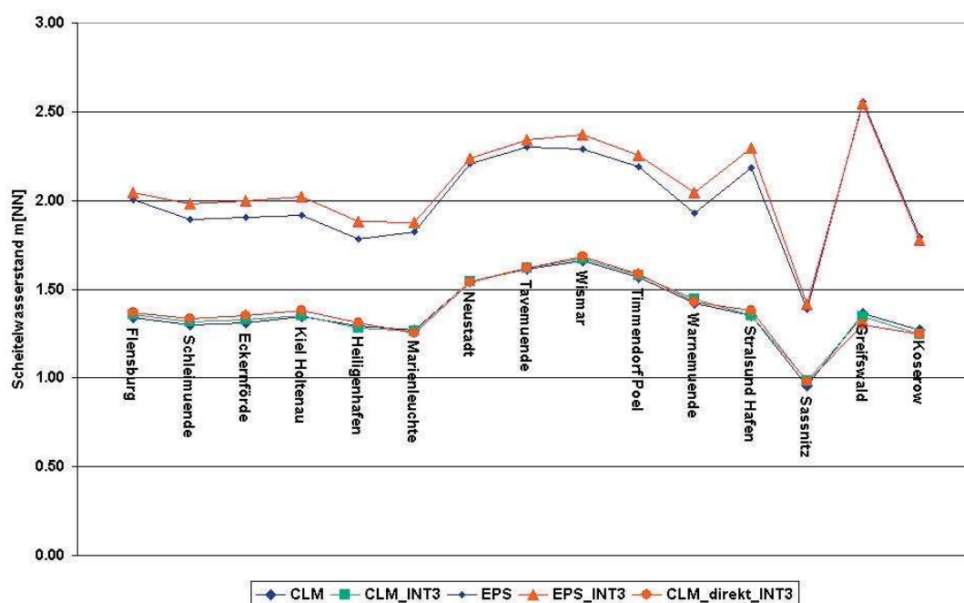
Abb. 5: Simulierte Scheitelwasserstände an der deutschen Ostseeküste. Simuliert mit dem Ostseemodell des BSH, das mit verschiedenen meteorologischen Daten („Antriebsdaten“) angetrieben wurde. Ausgangslage: Extremes EPS-Member zum 3.11.1995. Die Legende bedeutet Folgendes: CLM: Atmosphärendaten aus COSMO-CLM; CLM_INT3: Atmosphärendaten aus COSMO-CLM, jedoch seinerseits mit um drei Stunden verlangsamt abgelaufener Antriebsdaten angetrieben; EPS: Atmosphärendaten aus EPS; EPS_INT3: Atmosphärendaten aus EPS, diese aber um drei Stunden gestreckt ins Ostseemodell des BSH eingelesen; CLM_direkt_INT3: Atmosphärendaten aus dem COSMO-CLM, diese aber um drei Stunden gestreckt in das Ostseemodell des BSH eingelesen. Simulationsdaten der BSH-Simulation und Abbildung: BORK (2007)
