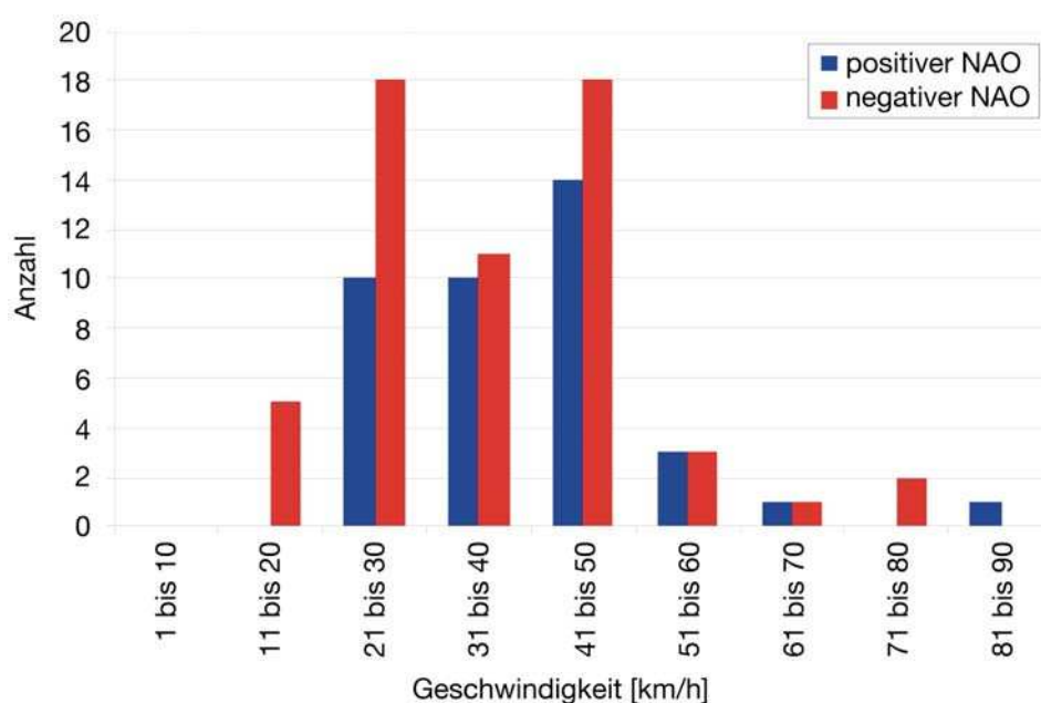
Abb. 3: Häufigkeitsverteilung Zuggeschwindigkeiten sturmfluterzeugender Sturmtiefs bei positivem bzw. negativem NAO-Index (1953 bis 1997)
