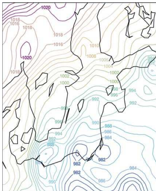
Abb. 8: Bodennahes Luftdruckfeld im untersten Modelllevel des COSMO-CLM bei maximalem Spectral Nudging des Horizontalwindes
