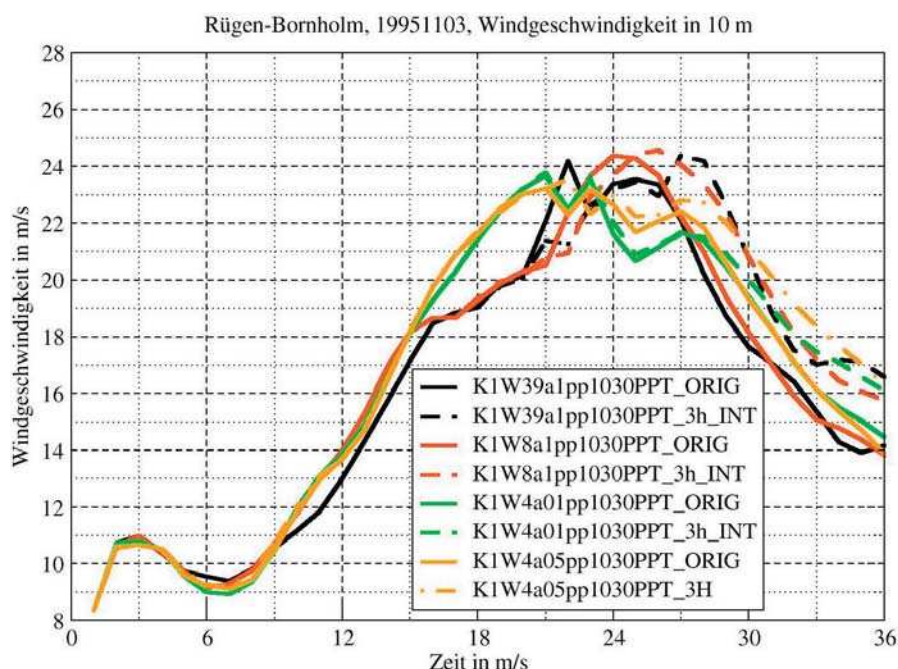
Abb. 10: Zeitreihe der Windgeschwindigkeit am Wassergitterpunkt zwischen Rügen und Bornholm. Simulation mit dem COSMO-CLM, jeweils mit Spectral Nudging des Luftdrucks und der Temperatur. In der Legende bedeuten die Kürzel Folgendes: K1: „Konstant Eins“ (Spectral Nudging nicht höhenabhängig, insbesondere keine abnehmende Gewichtung in Richtung Erdboden); W39 bzw. W8 oder W4: Anzahl der Wellenzahlen, die per Nudging aus dem Antriebsdatensatz übernommen werden (W4: nur
