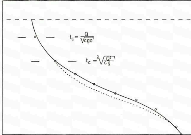
Abb. 2. Vergleich von halbanalytischer Salzzunge (durchgezogene Linie) mit experimentellen Daten. Punktiert: Keulegans Salzzunge, kritische Strömung an der Ästuarmündung Kreise: Keulegans Salzzunge, an halbanalytische Kurve angepaßt Gestrichelt: Wasseroberfläche
