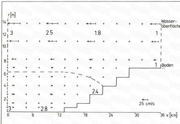
Abb. 3. Strömungsgeschwindigkeiten (Pfeile) und Salzgehalt (Zahlen) in einem durchmischten Ästuar, stationärer Zustand. Die gestrichelte Linie trennt die Gebiete stromauf und stromab gerichteter Geschwindigkeiten.
