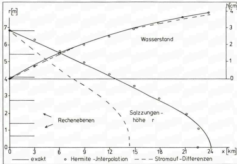
Abb. 1. Stationäre Salzzungenprofile und Wasserstände — halbanalytische Lösung, \circ\circ\circ Transport mittels Hermite-Interpolation, --- Transport mittels stromauf gerichteter Differenzen.
