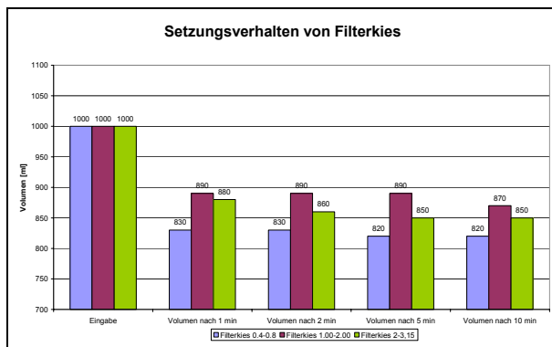
Bild 12: Setzungsverhalten und Setzungsmaß in Filterkiesen in Funktion der Zeit
