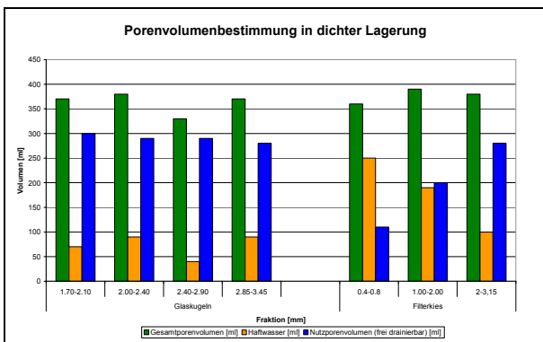
Bild 9: Ergebnisse der Porenraumbestimmung sowie der Anteile an nicht frei drainierbaren Wasseranteilen im Filterkies und in Glaskugeln mit dichter Lagerung
