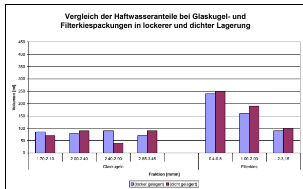
Bild 11: Ergebnisse der Bestimmung der Haftwasser- bzw. Kapillarwasseranteile in Filterkiesen und Glaskugeln in lockerer und dichter Lagerung
