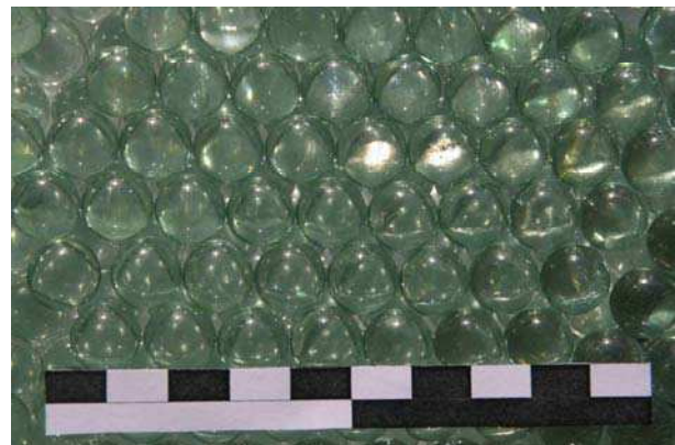
Bild 5: Haufwerk von Glaskugeln 6 \text{ mm} in dichter Lagerung. Foto: Fa. Ochs, Nürnberg
