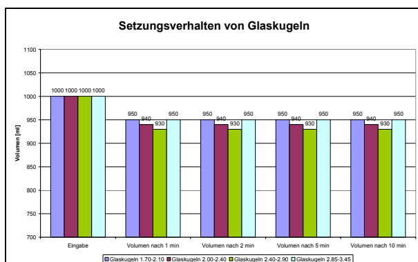
Bild 13: Setzungsverhalten und Setzungsmaß in Glaskugeln in Funktion der Zeit
