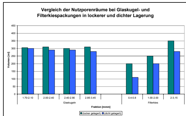
Bild 10: Ergebnisse der Nutzporenraumbestimmung an Filterkiesen und Glaskugeln in lockerer und dichter Lagerung
