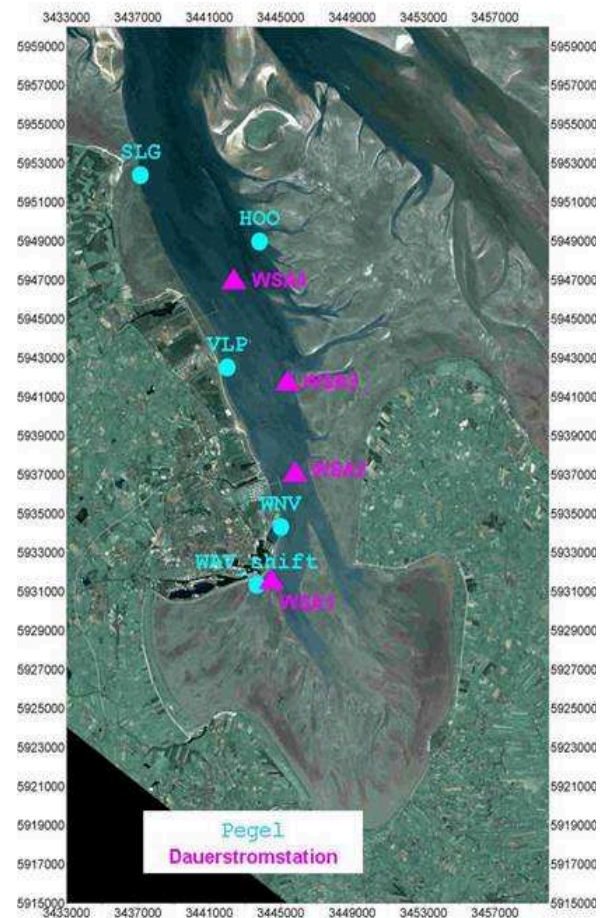
Bild 3. Standorte der Pegel und Dauerstromstationen (Foto: DLR)
