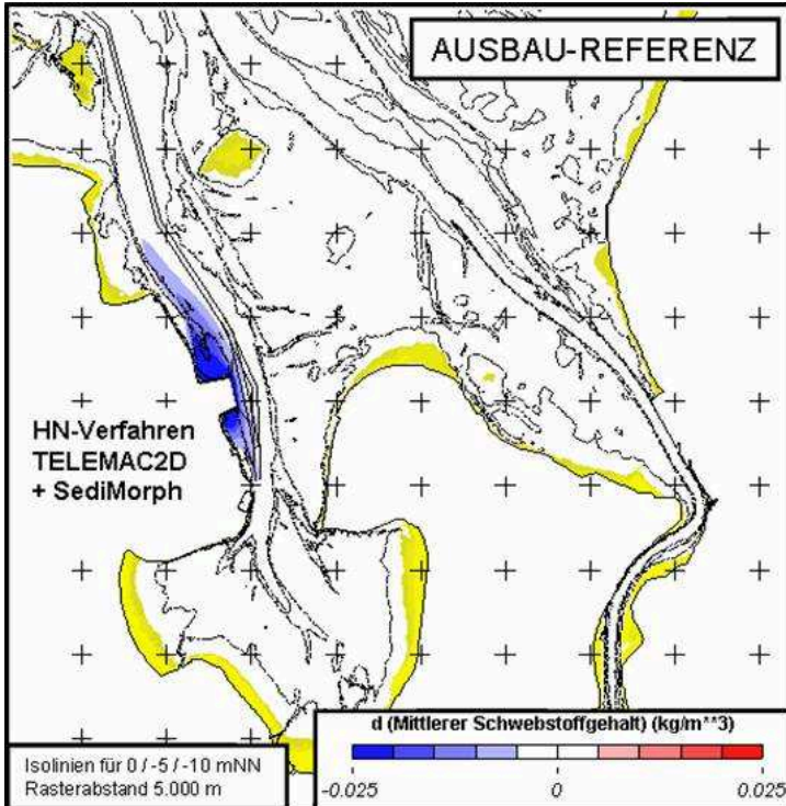
Bild 11. Ausbaubedingte Änderungen des mittleren Schwebstoffgehaltes
