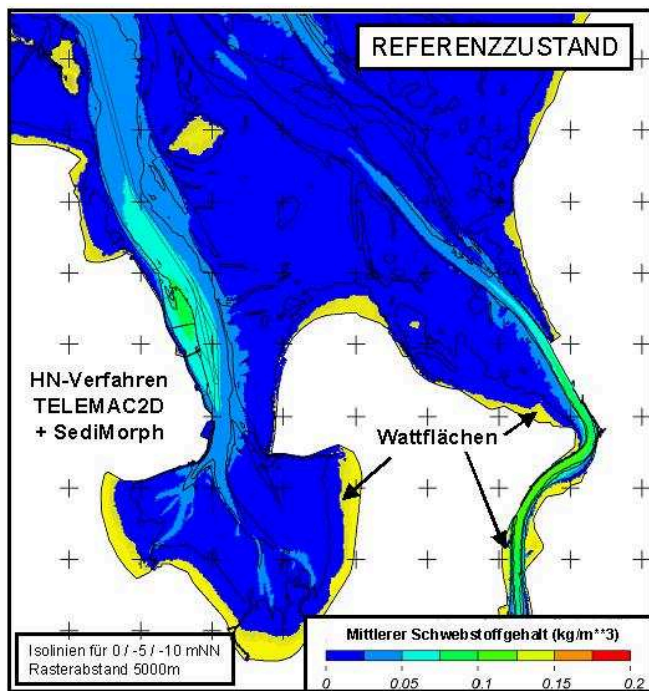
Bild 7: Gerechneter mittlerer Schwebstoffgehalt im Analysezeitraum für den Referenzzustand
