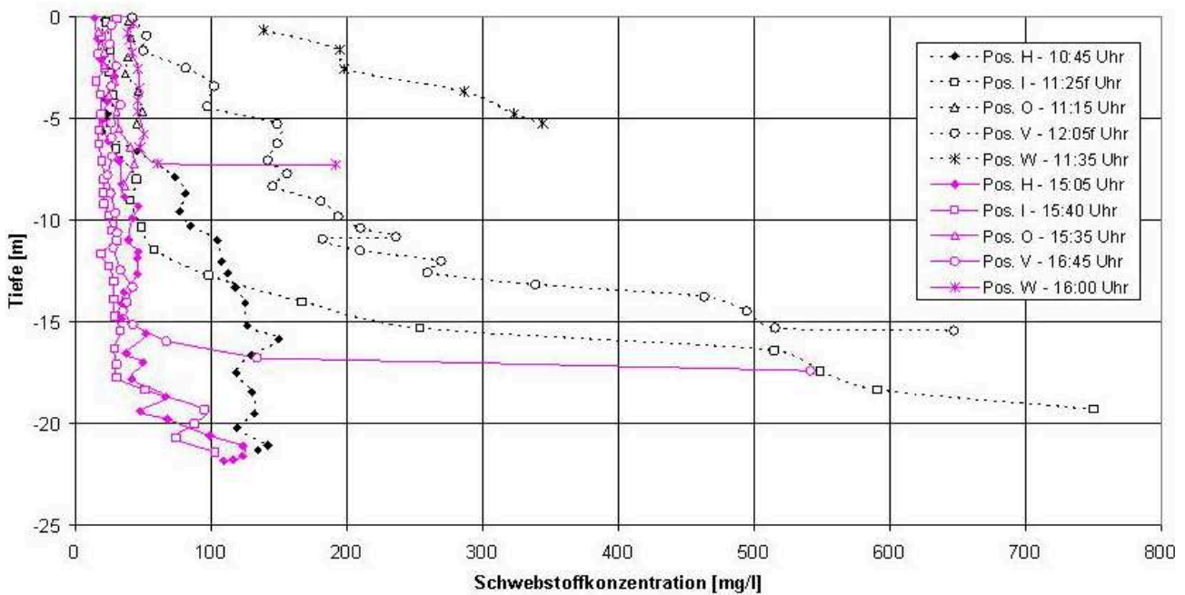
Bild 6: Gemessene Schwebstoffkonzentrationen in der Innenjade bei Flutstrom (gestrichelte Linien) und Flutstromkenterung der Springtide vom 21.03.2003 (Ingenieurbüro Visscher, Burgwedel, 2003)
