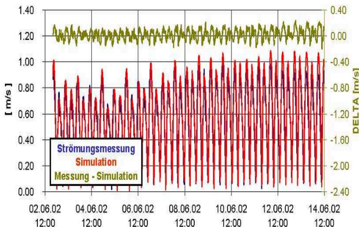
Bild 5: Vergleich der gemessenen und berechneten Strömungsgeschwindigkeiten für die Dauerstrommessstation 4 (WSA 4)
