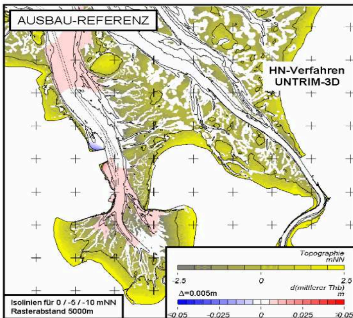
Bild 8. Ausbaubedingte Änderungen des Tidehubs
