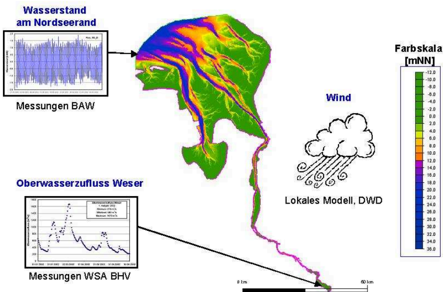
Bild 2: Schematische Übersicht des Modellgebietes sowie der in der Modellsteuerung berücksichtigten Randwerte
