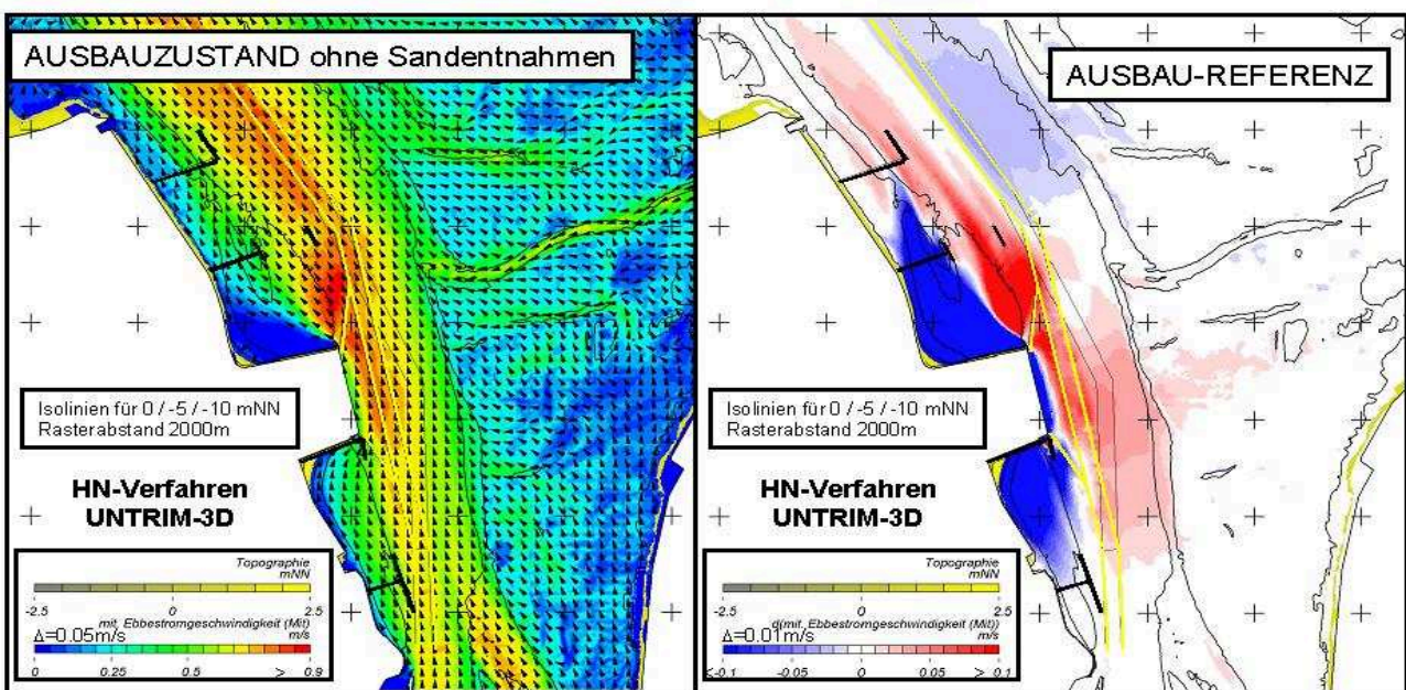
Bild 9. Mittlere Ebbestromgeschwindigkeiten (li.) und ausbaubedingte Änderungen der mittleren Ebbestromgeschwindigkeiten (re.)
