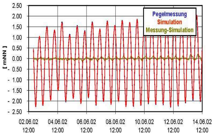
Bild 4: Vergleich der gemessenen und berechneten Wasserstandszeitreihen für den Pegel Wilhelmshaven Neuer Vorhafen
