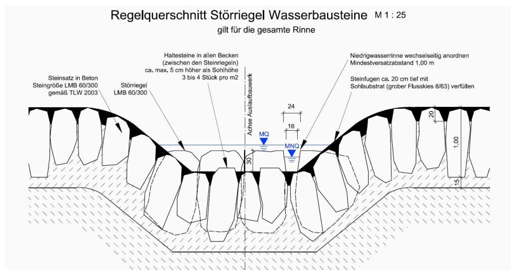
Abbildung 1: HRB Neuwürschnitz, Regelquerschnitt Störriegel (ARGE HPI ARCADIS)
