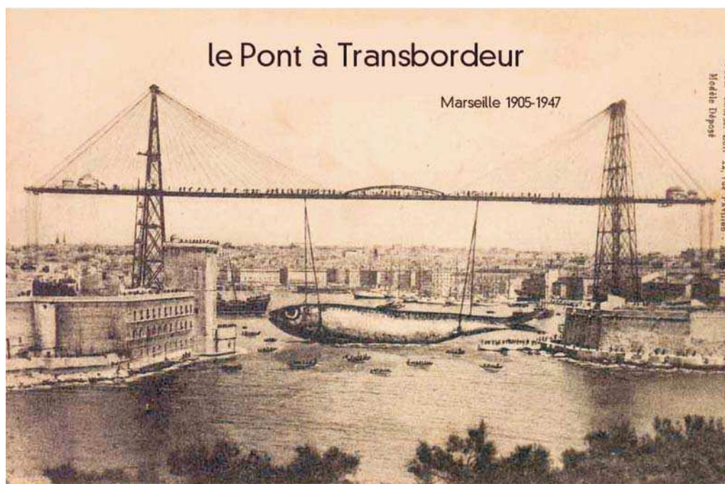
Abb. 9: Schwebefähre für große Lasten, Beispiel „Sardinentransport“ im Hafen von Marseille (Internet)
