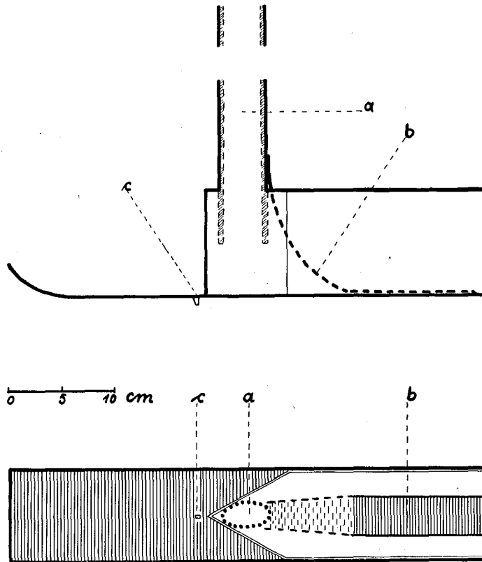
Abb. 13. Drillkufe. Oben: Seitenansicht (schemat.); unten: Grundriß a = Saatrohr, b = Schleiffeder, c = Drilldorn.
