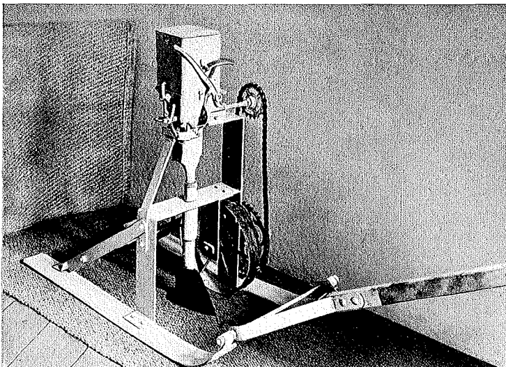
Abb. 9. Watt-Drillschlitten mit mechanischer Samenförderung. Bildarchiv Westküste B — a 768, 771, 770 Aufnahmen E. Wohlenberg
