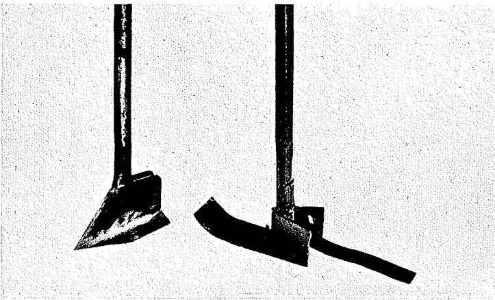
Abb. 8. Die auswechsel- baren Saatbett- bereiter. Links: Drillschar für Sandwatten, Rechts: Drillkufe für Schlickwatten.
