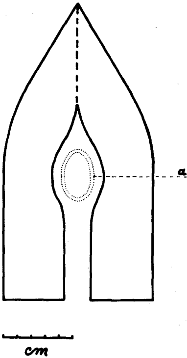
Abb. 10. Drillschar, Grundriß a=Saatrohr
