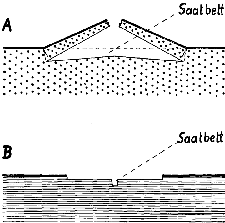
Abb. 14. Die Form der Saatbetten. Das von der Drillschar im Sandwatt (A) und von der Drillkufe im Schlickwatt (B) bereitete Saatbett.
