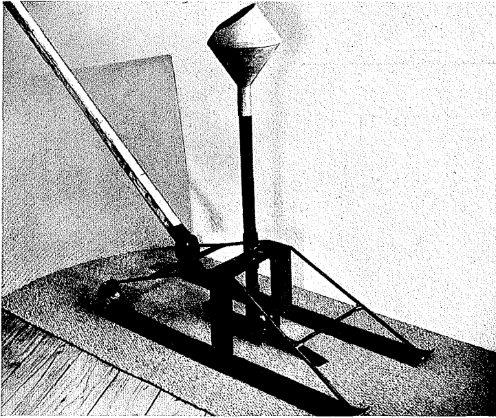
Abb. 7. Watt-Drillschlitten mit Drillkufe und Saattrichter.
