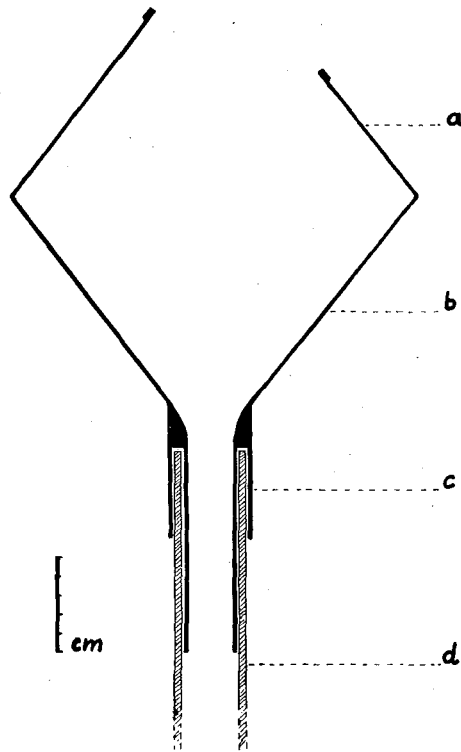
Abb. 12. Saattrichter für den Watt-Drillschlitten (Längsschnitt) a=Windschutzkragen b=Trichter c=Aufsatzkragen (Regenschutz) d=Saatrohr.
