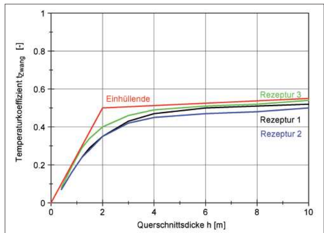
Bild 6-2: Temperaturkoeffizienten t_{Zwang}
