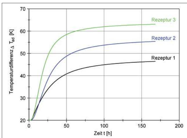
Bild 6-1: Adiabatische Temperaturerhöhung
