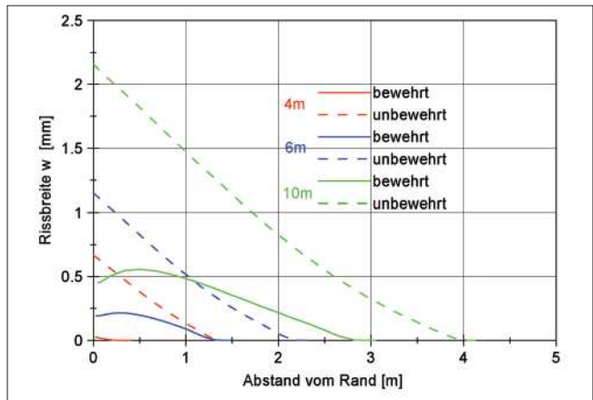
Bild 4-26: Maximale Rissbreiten
