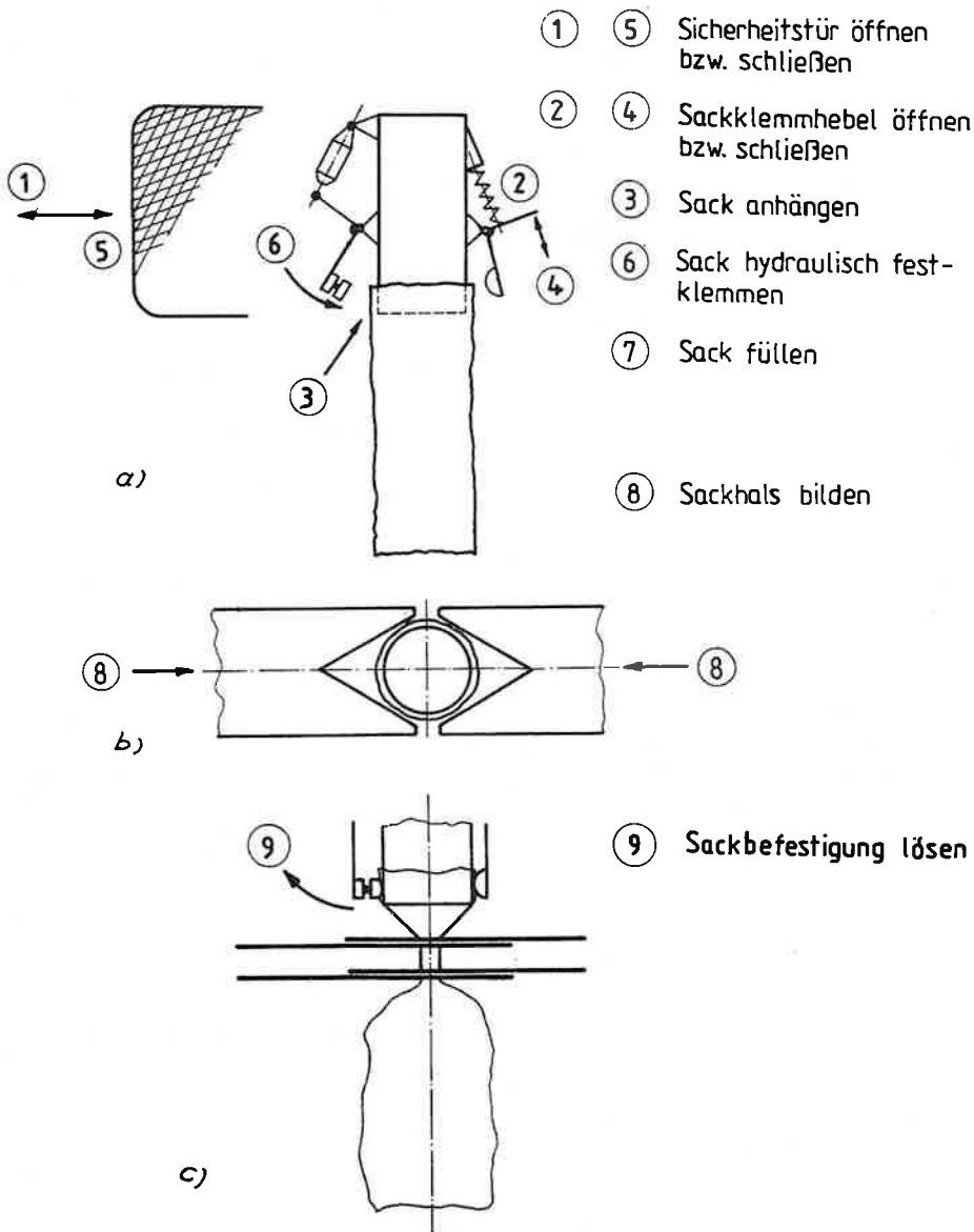
Bild 10 a....f Schematische Darstellung des Sackfüll- und -verschließprozesses
