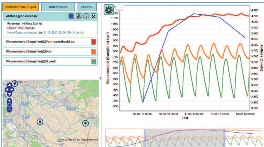
Abbildung 5: Sensor Web Client Zeitreihenanzeige – Extremhochwasserereignis in Geesthacht an der Elbe – Parameter Wasserstand und Abfluss.
