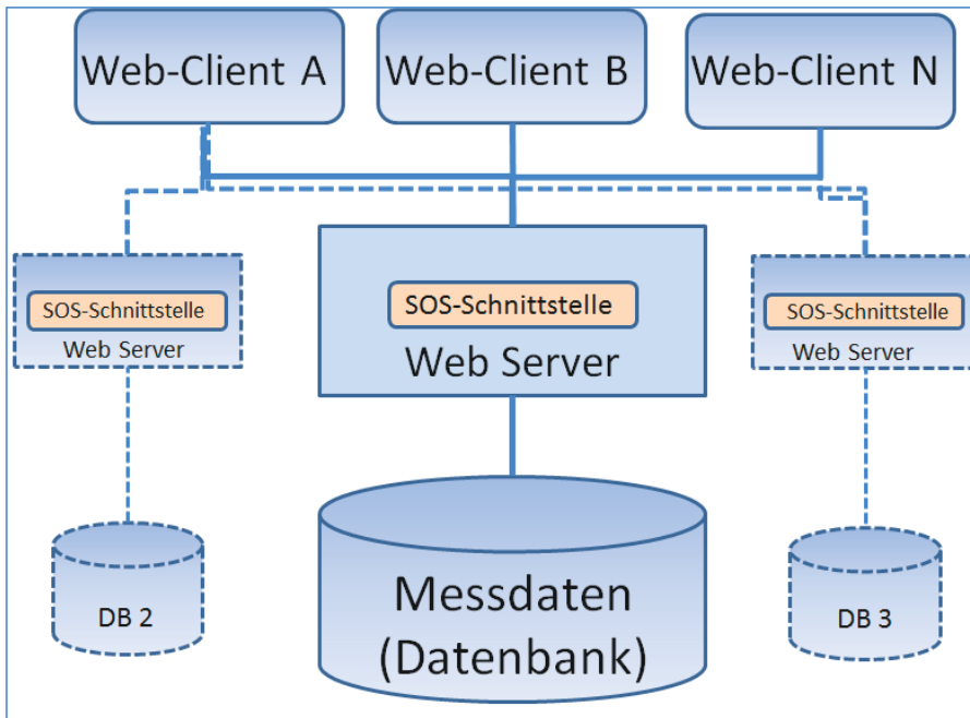
Abbildung 3: Typische SOS-Konfiguration.
