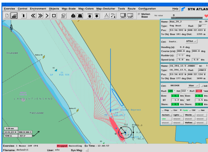
Abb. 8: nautische Simulation eines Wendemanövers
