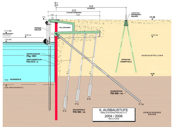
Abb. 9: Querschnitt Containerterminal CT 4
