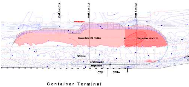
Abb. 7: erforderliche Baggerflächen
