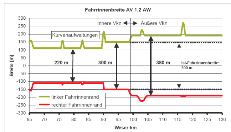
Abb. 4: Fahrinnenbreiten der angepassten Außenweser
