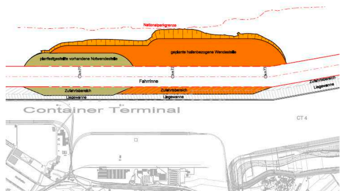
Abb. 6: alte und neue Wendestelle
