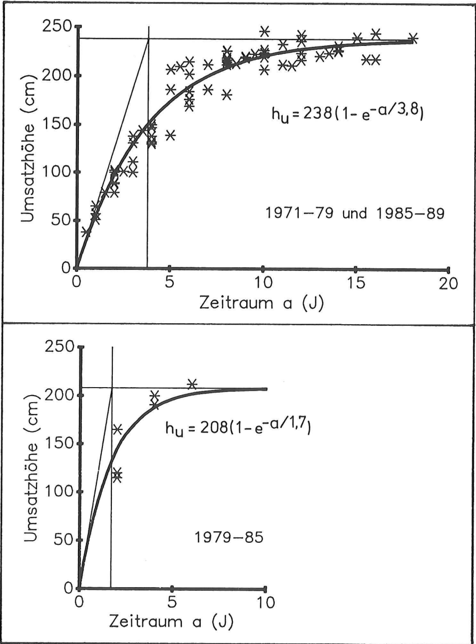
Abb. 20: Umsatzhöhen h_u über den Vergleichszeitraum a für die Perioden 1971-79/85-89 (oben) und 1979-85 (unten)
