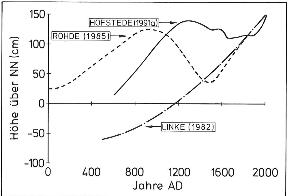
Abb. 2: Vergleich einiger rezenter MThw-Kurven für die innere Deutsche Bucht
