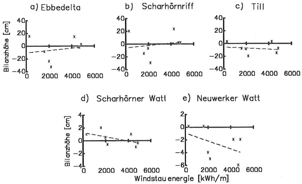
Abb. 12: Bilanzhöhen in Teilen des Küstenvorfeldes zwischen Außenelbe und Knechtsand und Windstauenergie
