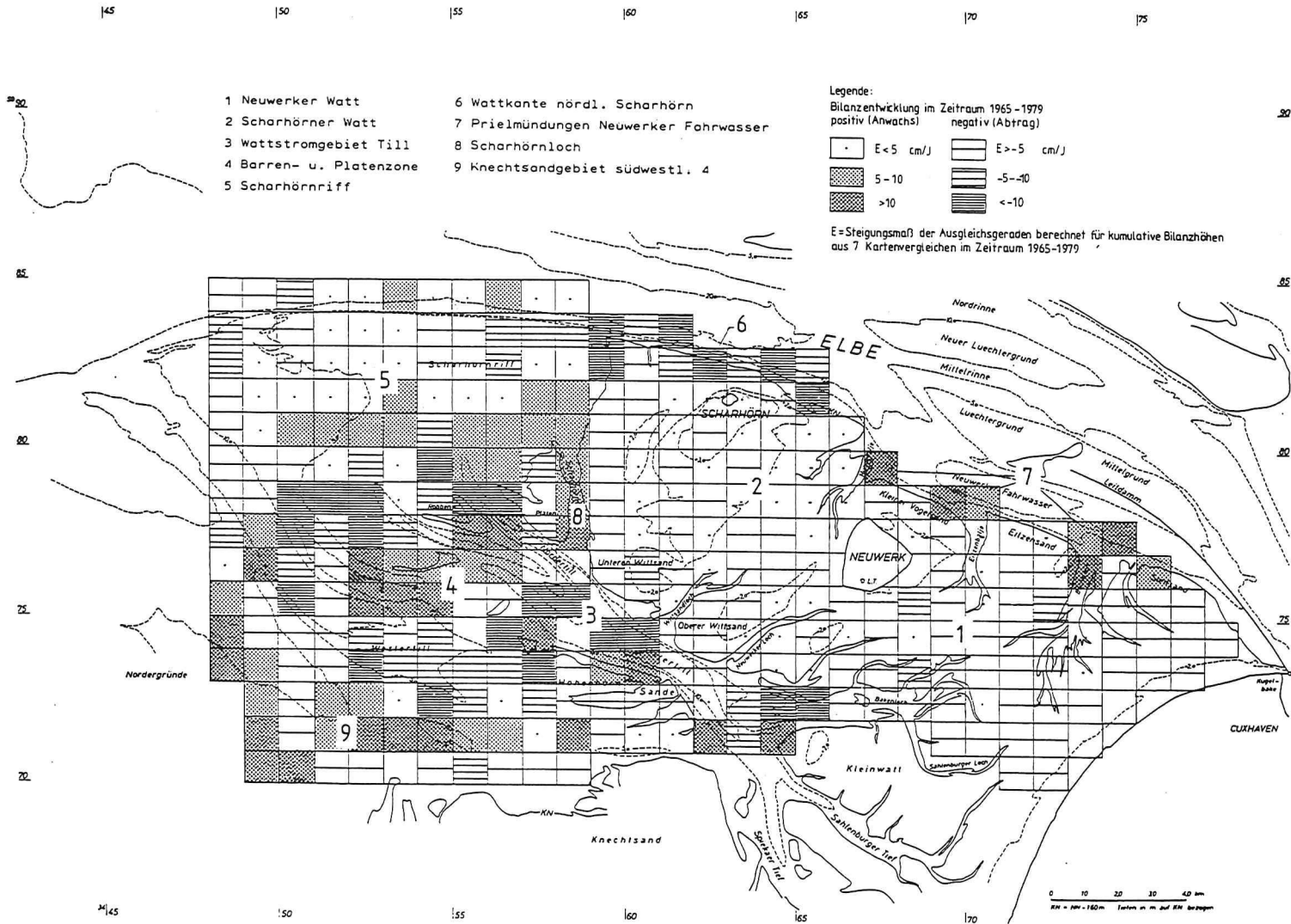
Abb. 5: Entwicklung der Bilanzhöhen zwischen 1965-1979 im Küstenvorfeld zwischen Außenelbe und Knechtsand
