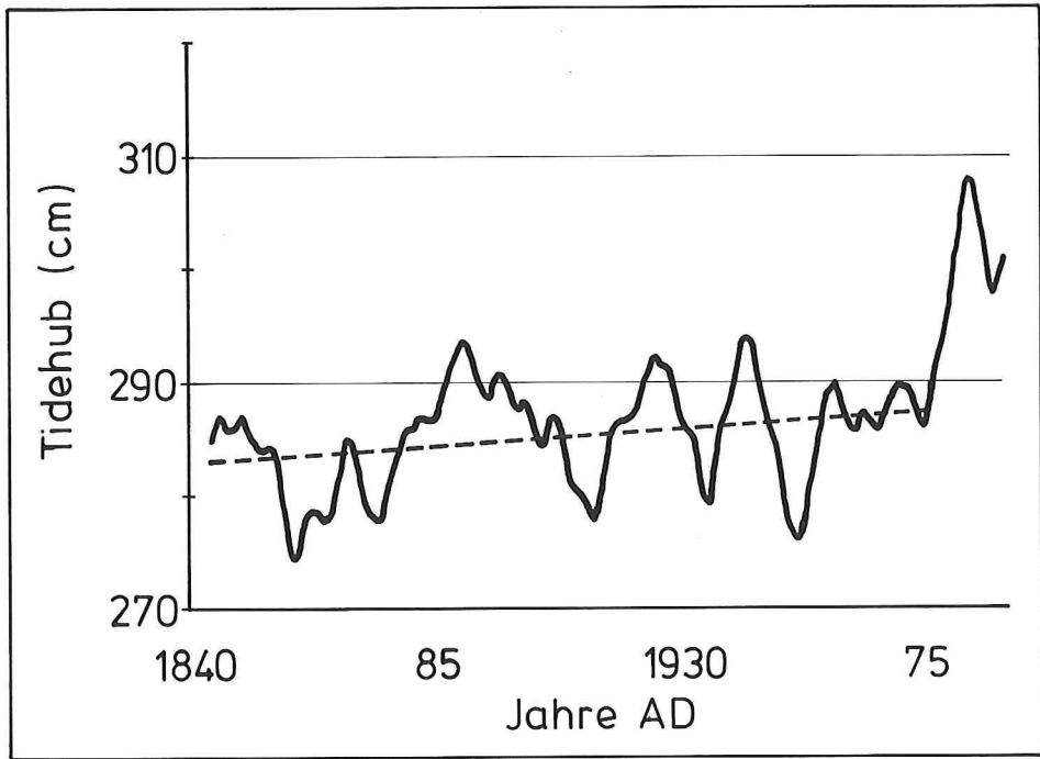
Abb. 3: MThb-Entwicklung am Pegel Steubenhöft, Cuxhaven seit 1844 (dreijährige übergreifende Mittel)
