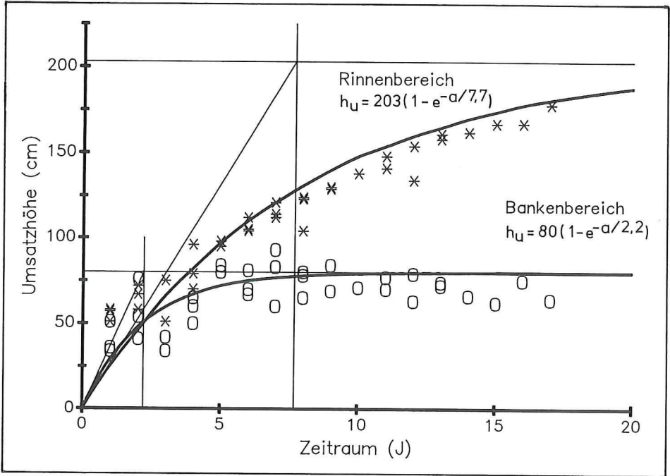
Abb. 15: Umsatzhöhen h_U über den Vergleichszeitraum a für die Teilgebiete Rinnenbereich (*) und Bankenbereich (o)
