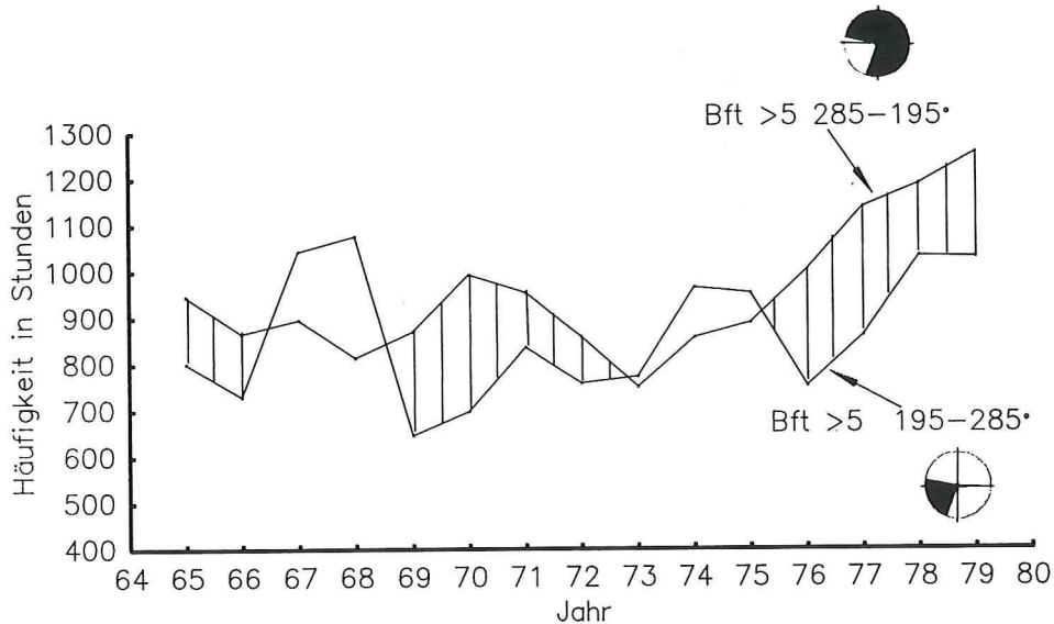
Abb. 10: Verteilung der summierten Stundenhäufigkeiten für die Windrichtungen 285–195° und 195–285° (Station Scharhörn)
