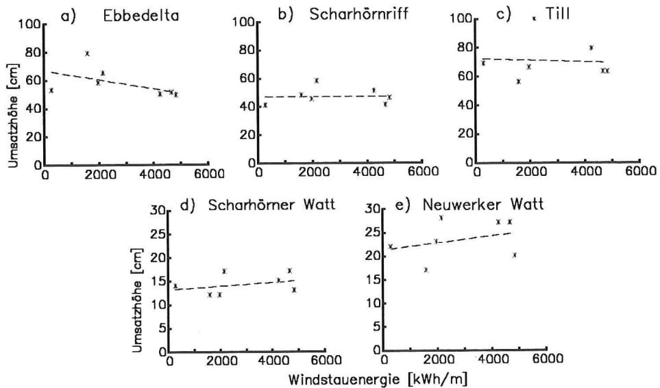
Abb. 13: Umsatzhöhe in Teilen des Küstenvorfeldes zwischen Außenelbe und Knechtsand und Windstauenergie
