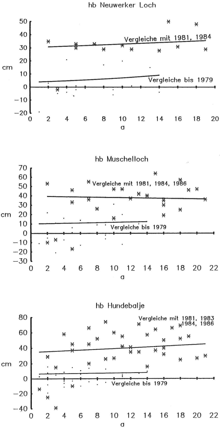
Abb. 4: Bilanzhöhen der Kartenvergleiche bis 1979 bzw. bis 1986 für verschiedene Prielgebiete
