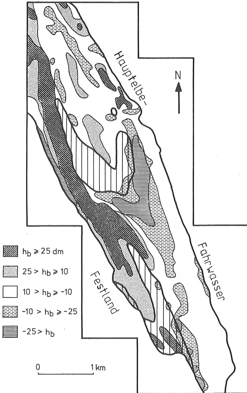
Abb. 17: Flächenmäßige Bilanzierung (Vergleich 1970–87) des Elbe-Randbereiches Brammerbank/Kraut-sander Watt
