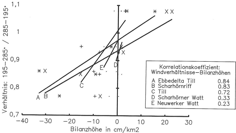
Abb. 11: Zusammenhang zwischen Windverhältnissen und Bilanzhöhen für Teilgebiete des Küstenvorfeldes zwischen Außenelbe und Knechtsand
