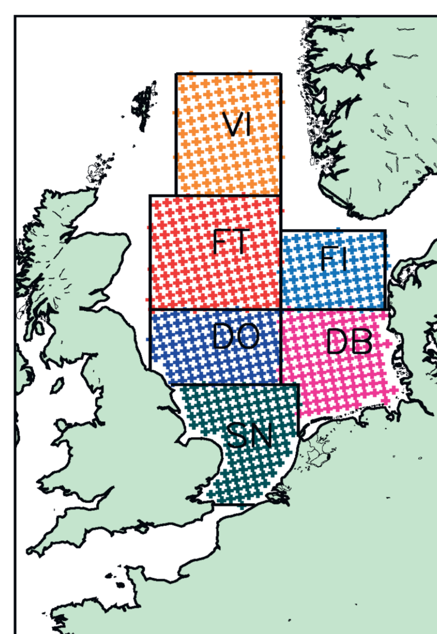
Abb. 1: Teilgebiete der Nordsee Viking (VI), Forties (FT), Fisher (FI), Dogger (DO), Deutsche Bucht (DB) und Südwestliche Nordsee (SN) mit REMO-Gitterpunkten über See.
