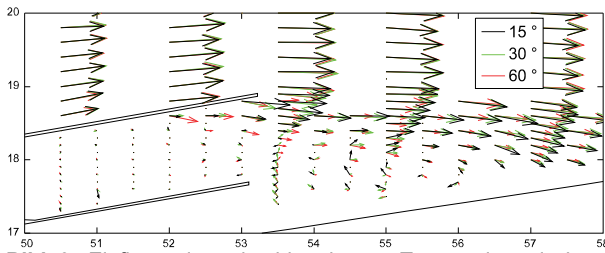
Bild 6: Einfluss einer durchbrochenen Trennmole zwischen Vorhafen und Fluss
