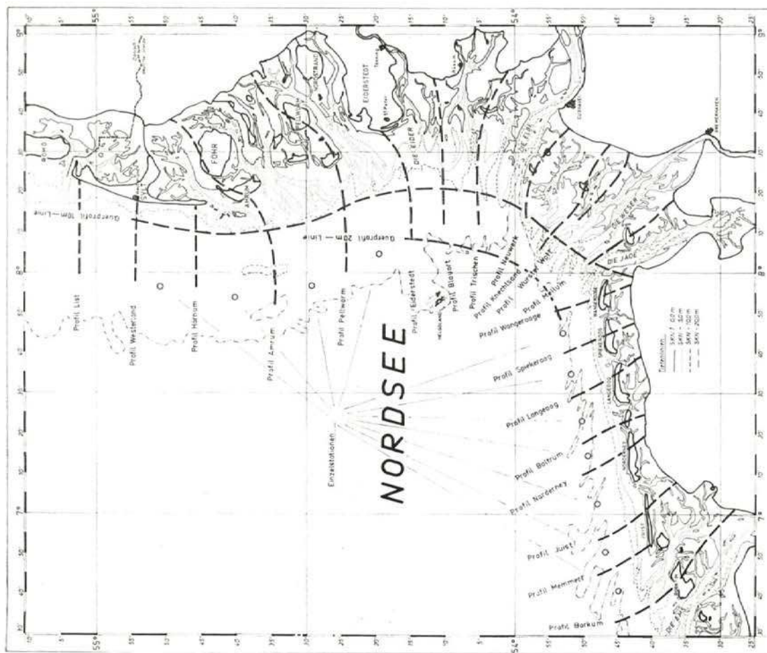
Abb. 2. Küstenforschungsprogramm, Vorschlag für Strömungsmeßprofile
