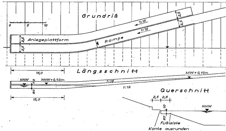
Abb. 6: Bootsschleppe — für Ruderboote (Vierer) — Einsetzstelle im Unterwasser
