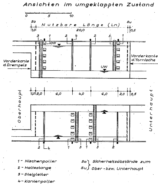
Abb. 1: Bootsschleuse Regelaurüstung der Kammerwände
