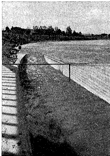
Abb. 5: Bootsgasse an der Lahn (Offene U-Gasse)
