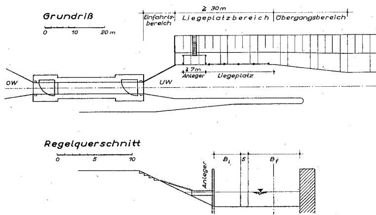
Abb. 2: Bootsschleuse — Vorhafen im Unterwasser
