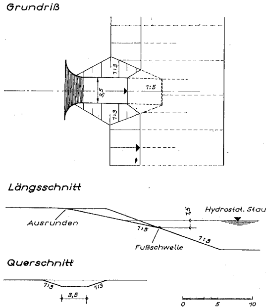
Abb. 8: Einsetzstelle für kleine Motorboote — Querrampe —
