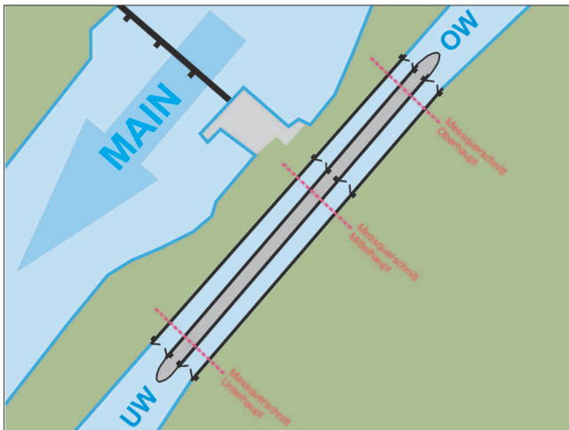
Bild 4: Schleusenquerschnitt mit Grundwassermessstellen Figure 4: Cross section of the lock with groundwater observation wells
