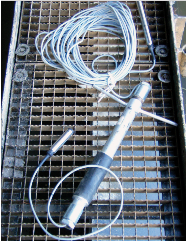
Bild 8 Messsystem bestehend aus Datenlogger und Packer (links) und eingebautes Messsystem (rechts) Figure 8: Measuring system consisting of data logger and packer (left) and installed measuring system (right)
