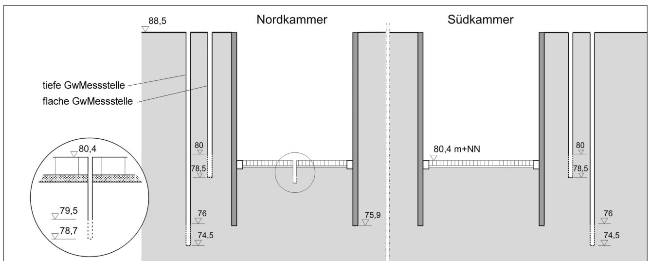
Bild 5: Lageplan Grundwassermessstellen Figure 5: Site map of groundwater observation wells
