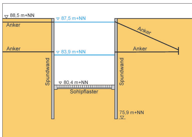
Bild 2: Querschnitt der Schleusenkammer Figure 2: Cross section of the lock chamber
