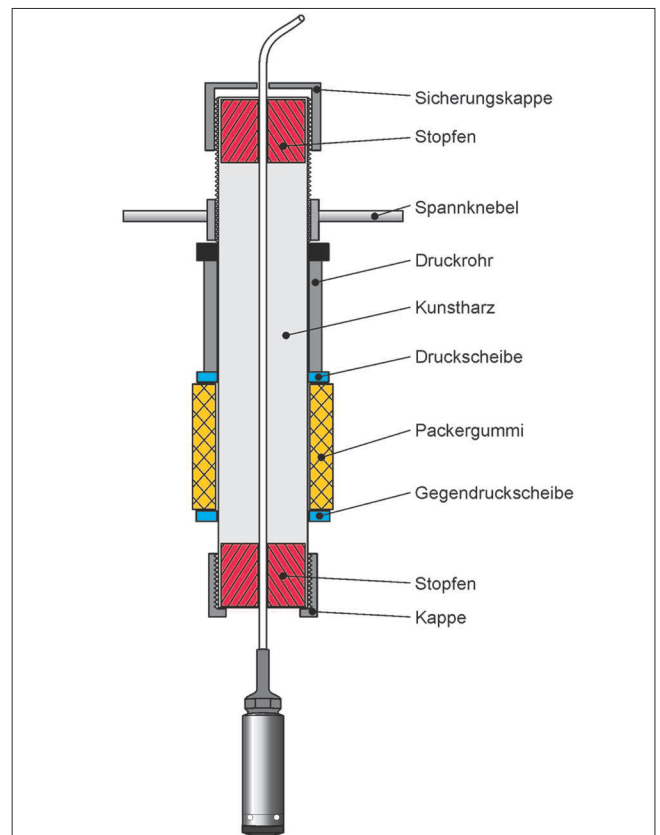
Bild 7: Messsystem mit Druckaufnehmer für den Einbau in die Grundwassermessstelle Figure 7: Measuring system with pressure transmitter for the installation in the piezometer
