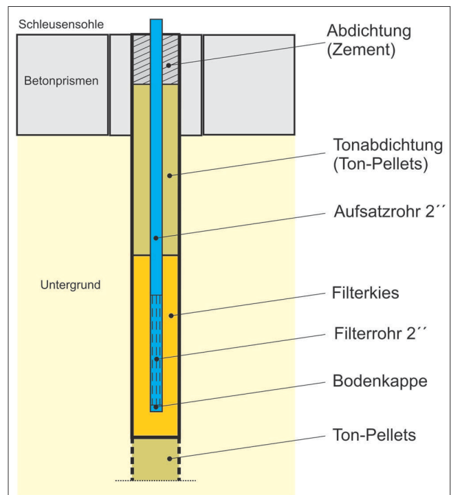
Bild 6: Ausbau der Grundwassermessstellen in der Schleusensole
