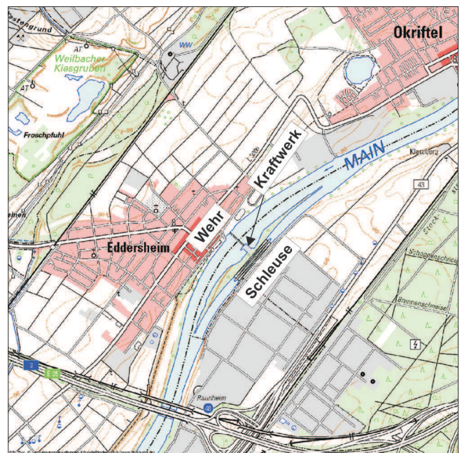
Bild 1: Lageplan Schleuse und Wehr Eddersheim Figure 1: Site map of Eddersheim lock and weir
