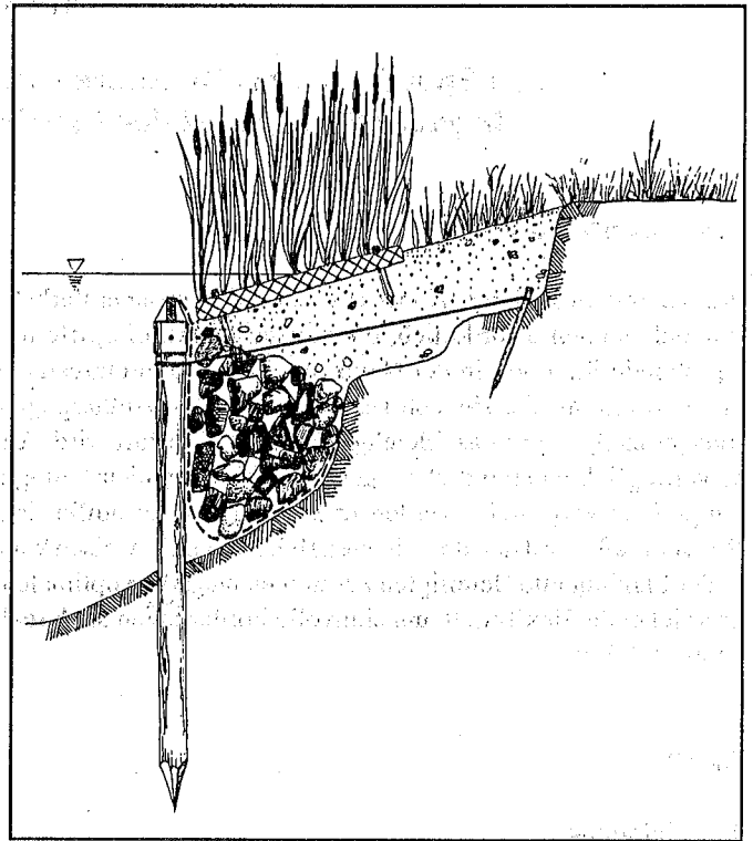
Abb. 1: Ufersicherung am steilen Abbruchufer
