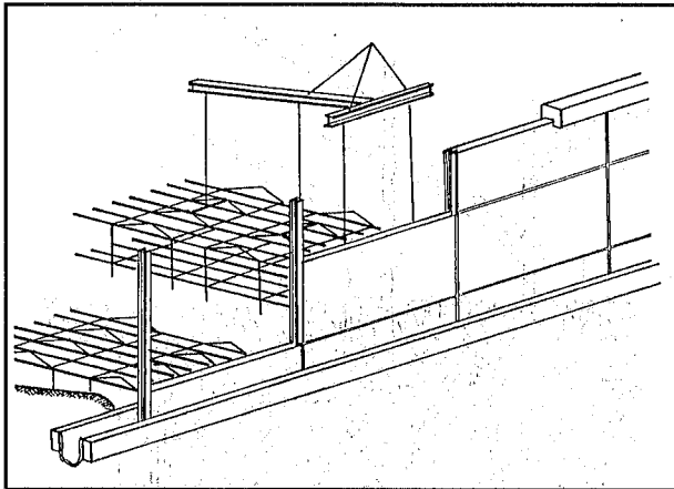
Abb. 5: Bewehrte Erde - Schemazeichnung für Unterwasserkonstruktion [9] Einsetzen von Wandpaneel und Bewehrungskorb an einer Krantraverse
