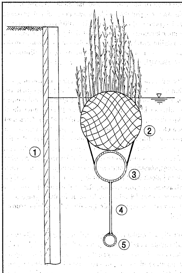
Abb. 4: Vegetationselement für vertikale Uferbefestigungen
