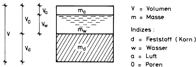
Bild 5: Gedankenmodell eines Bodenvolumens
