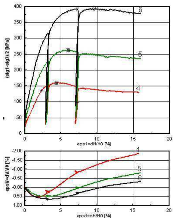
Bild 20: Versuchsergebnisse aus einem dräniertes Triaxialversuch, (oben) Spannungs-Verformungs-Verlauf, (unten) Volumen-Dehnungs-Verlauf
