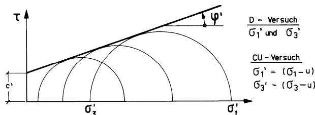
Bild 18: Konsolidierter, dräniertes (D-Versuch) bzw. konsolidierter, undrännertes (CU-Versuch) Versuch aus (Kempfert et al. 1998)
