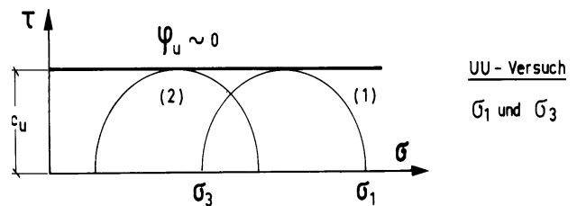
Bild 19: Unkonsolidiertes, undrännertes (UU-Versuch) Versuch aus (Kempfert et al. 1998)
