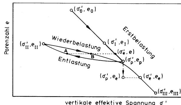
Bild 28: Druck-Porenzahl-Diagramm mit Erstbelastungs-, Entlastungs- und Wiederbelastungsästen aus (Scherzinger 1991)
