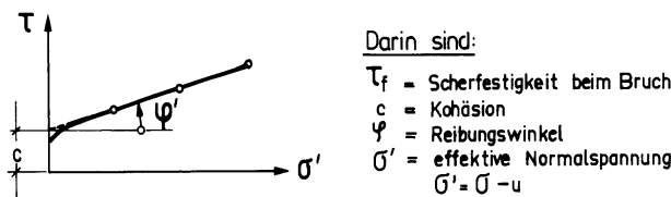
Bild 11: Coulombsche Bruchbedingung
