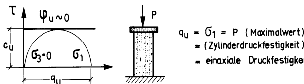
Bild 21: Zusammenhänge beim Einaxialversuch
