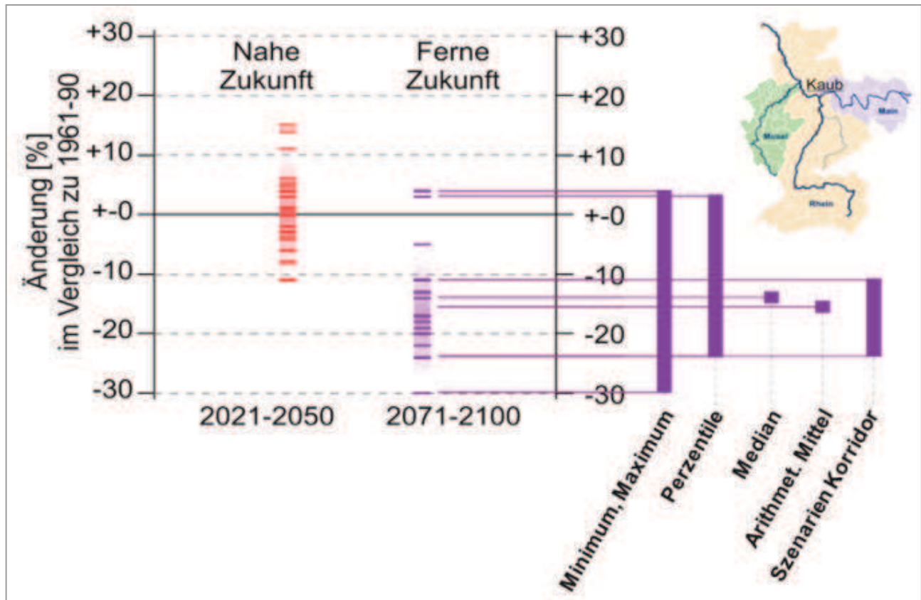
Abbildung 4: Beispiel-Diagramm zur Darstellung einer Bandbreite und Schema zur Beschreibung eines Ensembles inklusive des Szenarienkorridentors (Nilson et al. 2014)
