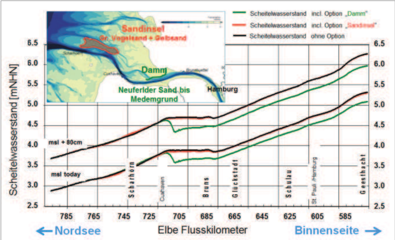
Abbildung 6: Effekte auf Sturmflutscheitelwasserstände durch die Optionen „Damm“ und „Sandinsel“ im Mündungsbereich des Elbe-Ästuars. Vergleich für den Referenzzustand „heute“ und für ein Szenario mit + 80 cm mittlerem Meeresspiegelanstieg (SEIFFERT et al. 2014)
