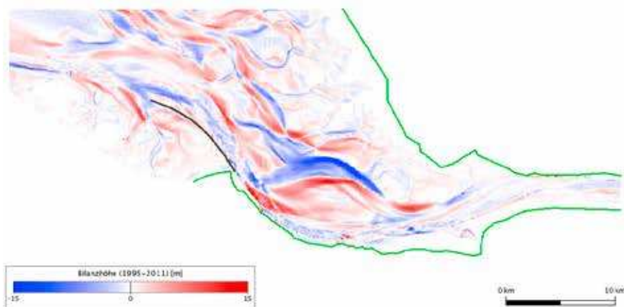
Abb. 16: Differenztopographie 2011-1995
