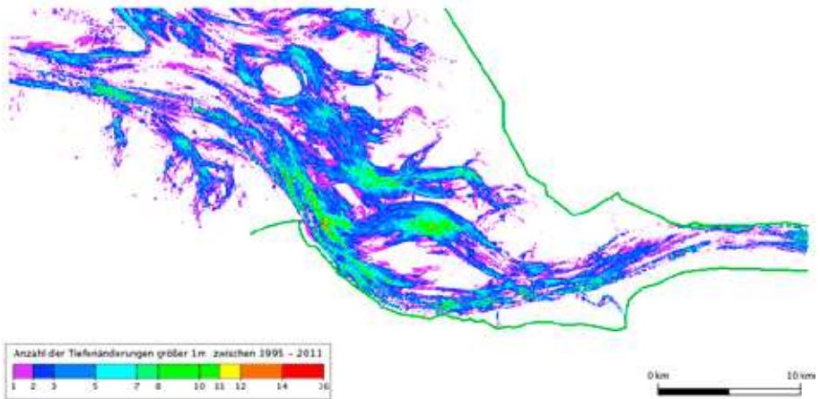
Abb. 19: Anzahl der Tiefenänderungen, die größer 1 m/a betragen, für den Zeitraum 1995-2011
