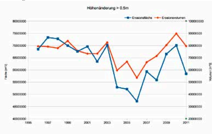
Abb. 21: Erosionsentwicklung Mündungsbereich der Elbe
