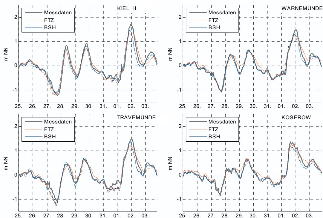
Abb. 10: Wasserstand an vier deutschen Pegeln für beide Modelle unter Verwendung des Windschubansatzes nach SMITH und BANKE 1975 im Vergleich mit Messungen für den Sturm 2006
