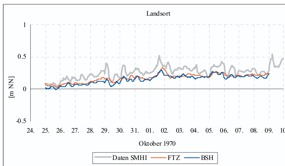
Abb. 18: Modellwasserstände und Pegelraten der Vorlaufsimulation Oktober/November 1970, angetrieben durch Era40-Windfelder, mit mittleren Flusseinträgen
