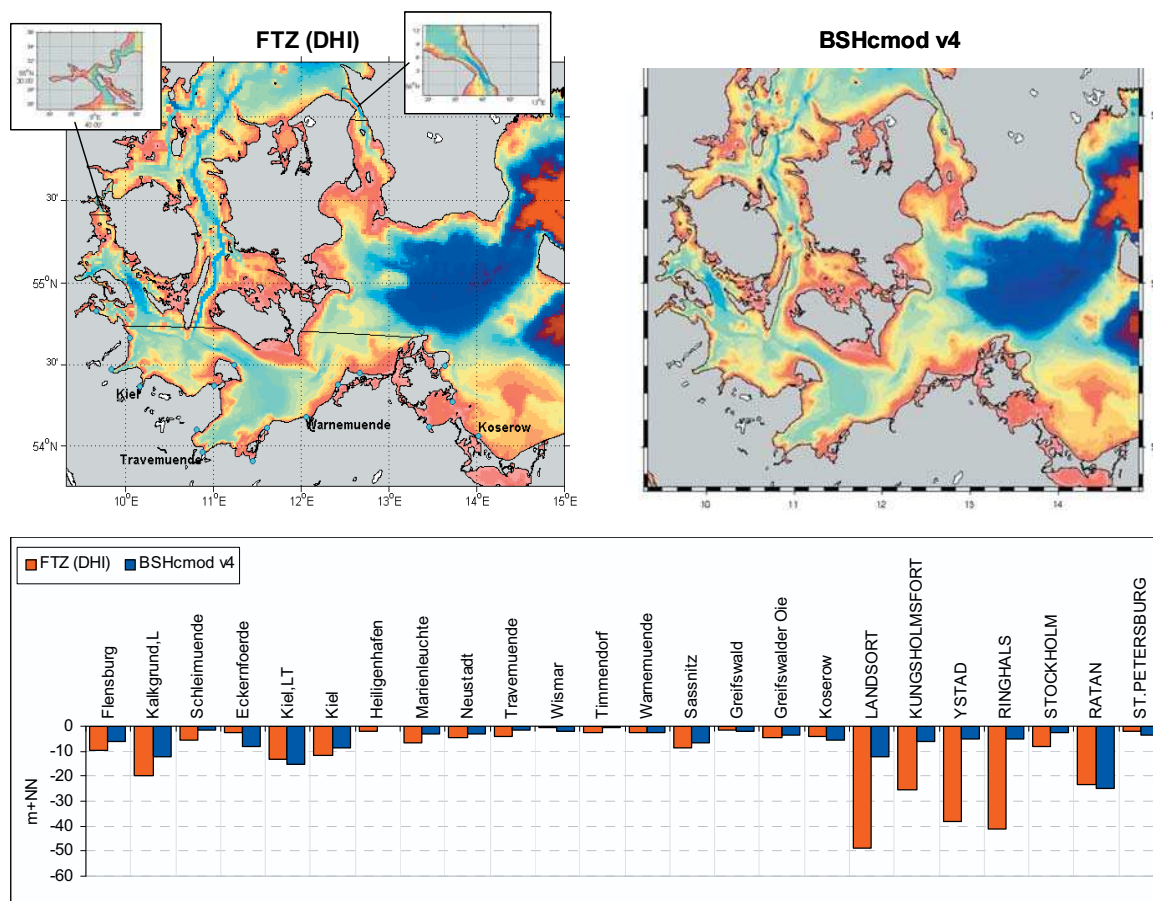
Abb. 2: Topographie der beiden Modelle in der westlichen Ostsee bei gleicher Farbskala und Modell-tiefen an 17 deutschen, sechs schwedischen und einem russischen Pegelort
