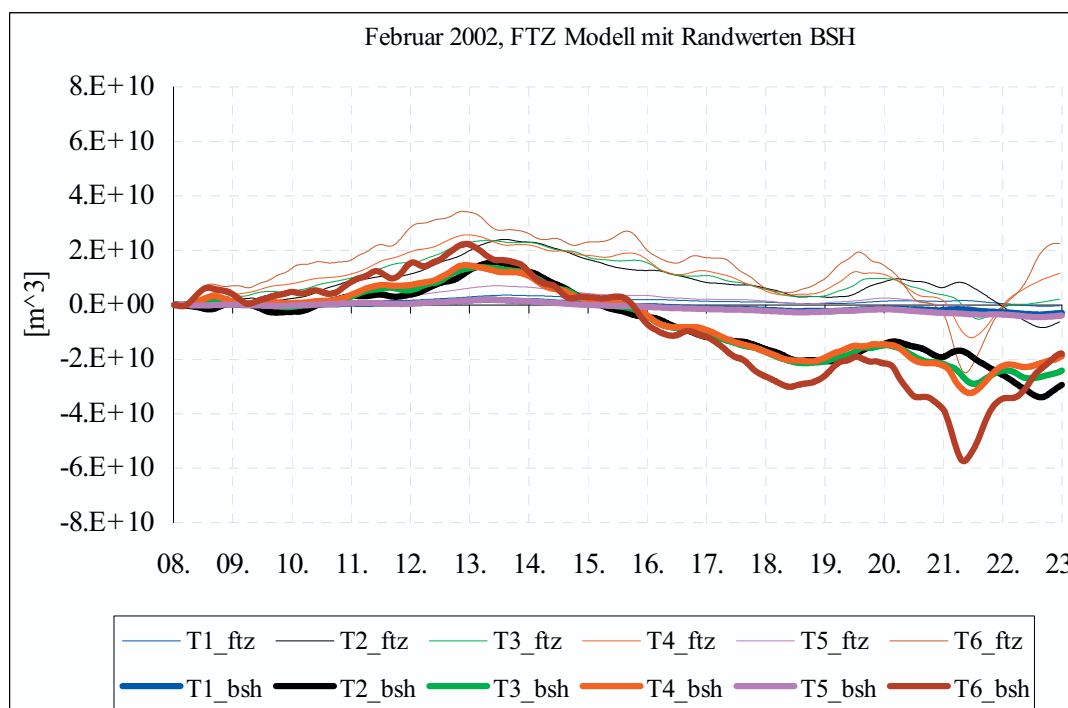
Abb. 17: Kumulative Transporte durch die Schnitte aus Abb. 15
