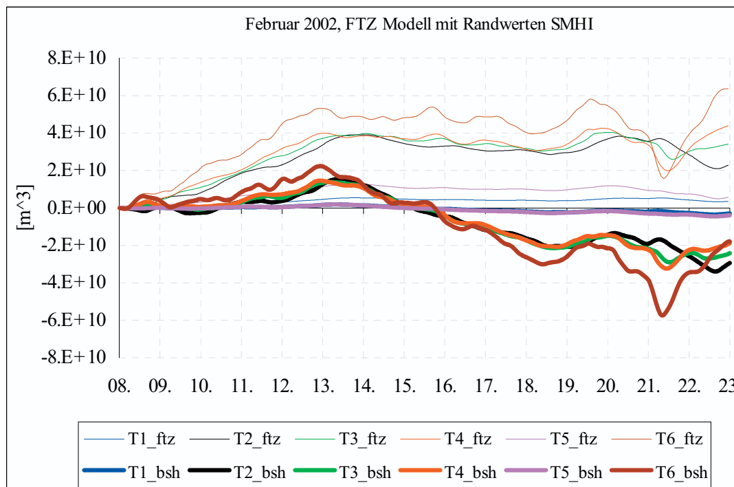
Abb. 16: Kumulative Transporte durch die Schnitte aus Abb. 15.
