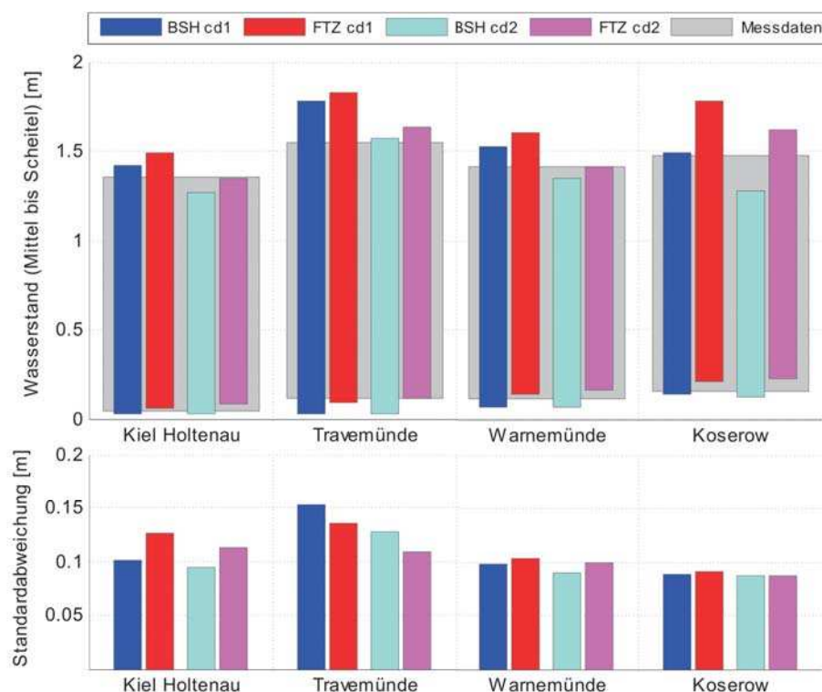
Abb. 8: Statistische Verifikation der Modelle für den Zeitraum 13.–23. Februar 2002, unter Verwendung zweier unterschiedlicher Windschubansätze
