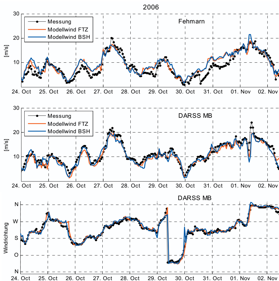
Abb. 9: Vergleich der Windgeschwindigkeiten und Richtungen interpoliert auf beide Modellgitter mit Messdaten für den Sturm November 2006
