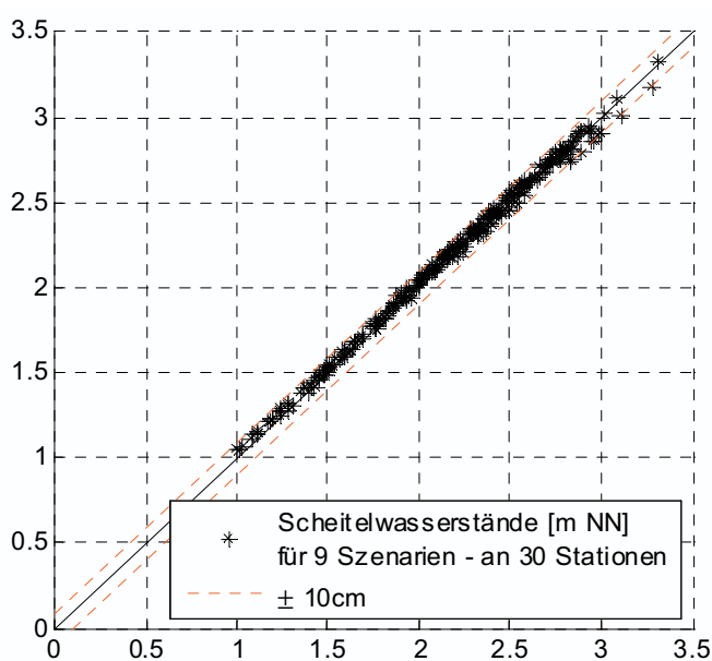
Abb. 21: Vergleich von Scheitelwasserständen an der deutschen Ostseeküste berechnet mit dem FTZ-Modell unter Verwendung unterschiedlicher Randwerte
