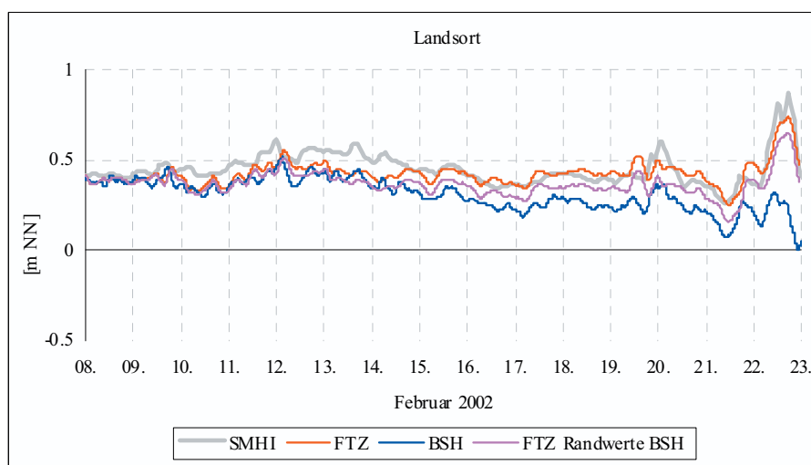
Abb. 14: Modellwasserstände und Pegeldaten in Landsort Februar 2002
