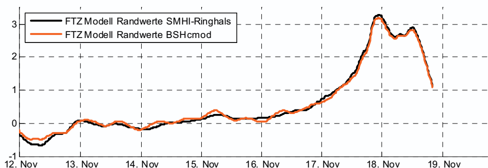
Abb. 20: Wasserstände des FTZ-Modells in Flensburg
