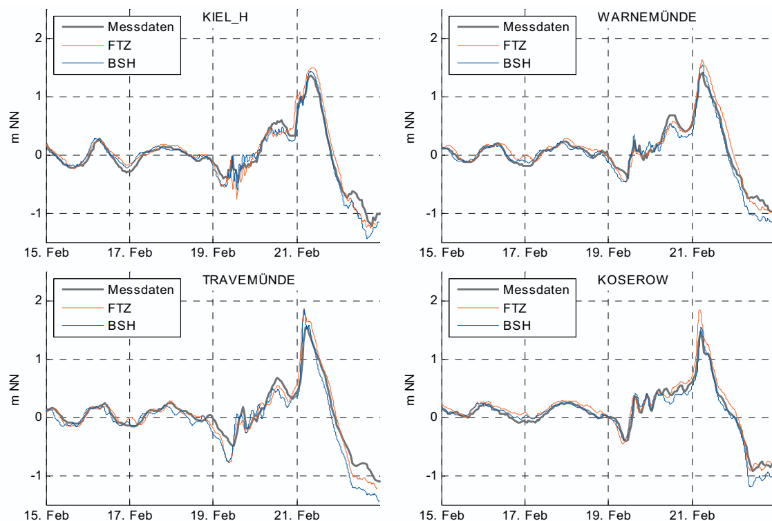
Abb. 7: Wasserstand an vier deutschen Pegeln für beide Modelle unter Verwendung des modifizierten Windschubansatzes nach SMITH und BANKE 1975 im Vergleich mit Messungen für den Sturm 2002
