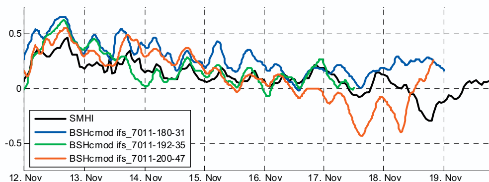
Abb. 19: Pegelraten und Modellwasserstände des BSH für 3 EPS-Stürme in Ringhals (Bezeichnungen in BORK u. MÜLLER-NAVARRA [2009]: 1970_31b0c2, 1970_35b0cw und 1970_47b0d1)
