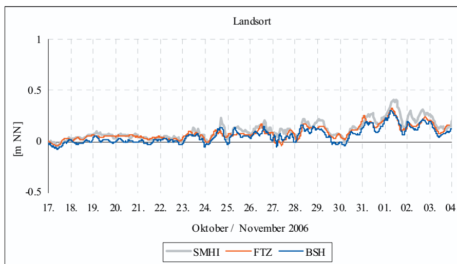
Abb. 13: Modellwasserstände und Pegeldaten in Landsort Oktober/November 2006
