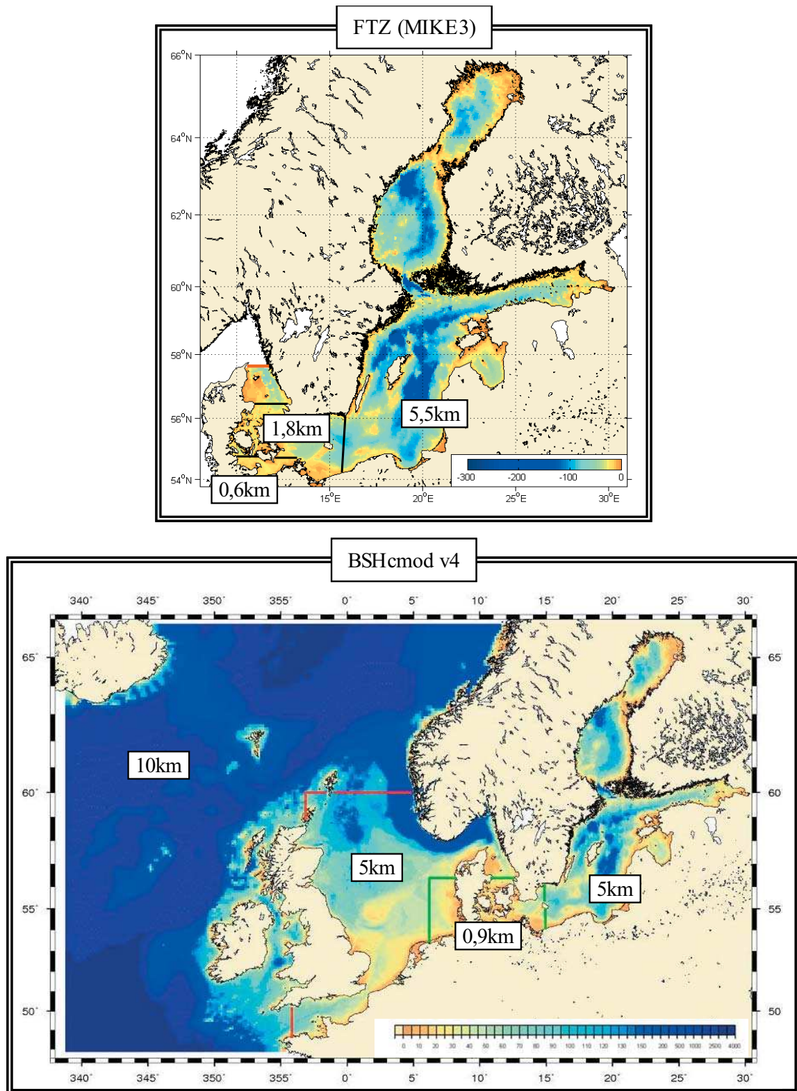
Abb. 1: Modellgebiete, Topographien und horizontale Auflösung der beiden Modelle bei ähnlicher Farbskala. Oben: das am FTZ eingesetzte Modell auf Basis der MIKE3 Software des DHI; unten: das am BSH entwickelte und operationell betriebene Modell BSHcmod v4
