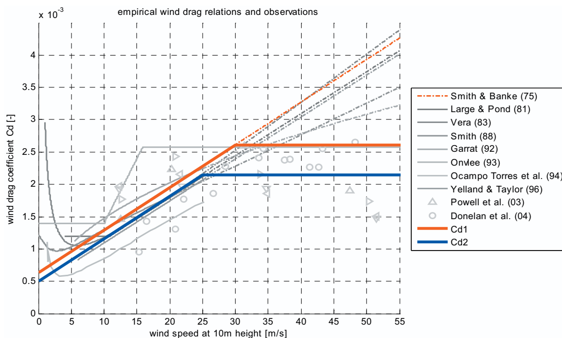
Abb. 3: Empirisch bestimmte Windschubkoeffizienten und neuere Sturmtiefmessdaten
