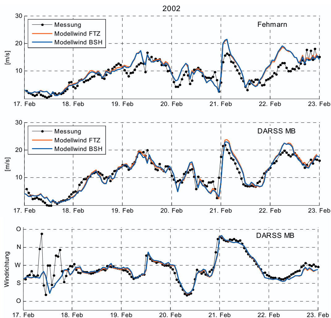
Abb. 6: Vergleich der Windgeschwindigkeiten und Richtungen interpoliert auf beide Modellgitter mit Messdaten für den Sturm Februar 2002
