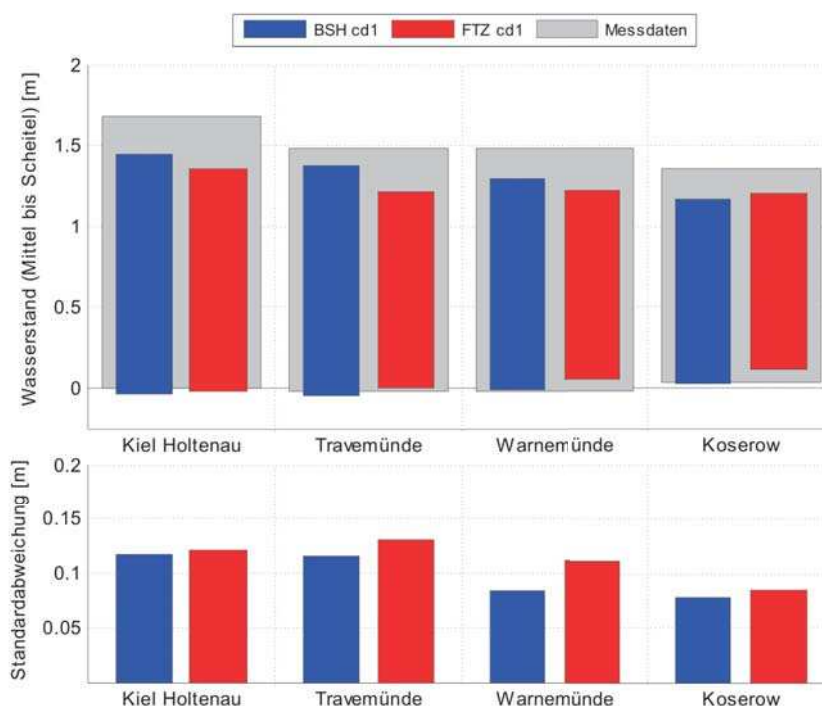
Abb. 11: Statistische Verifikation der Modelle für den Zeitraum 19. Oktober bis 4. November 2006
