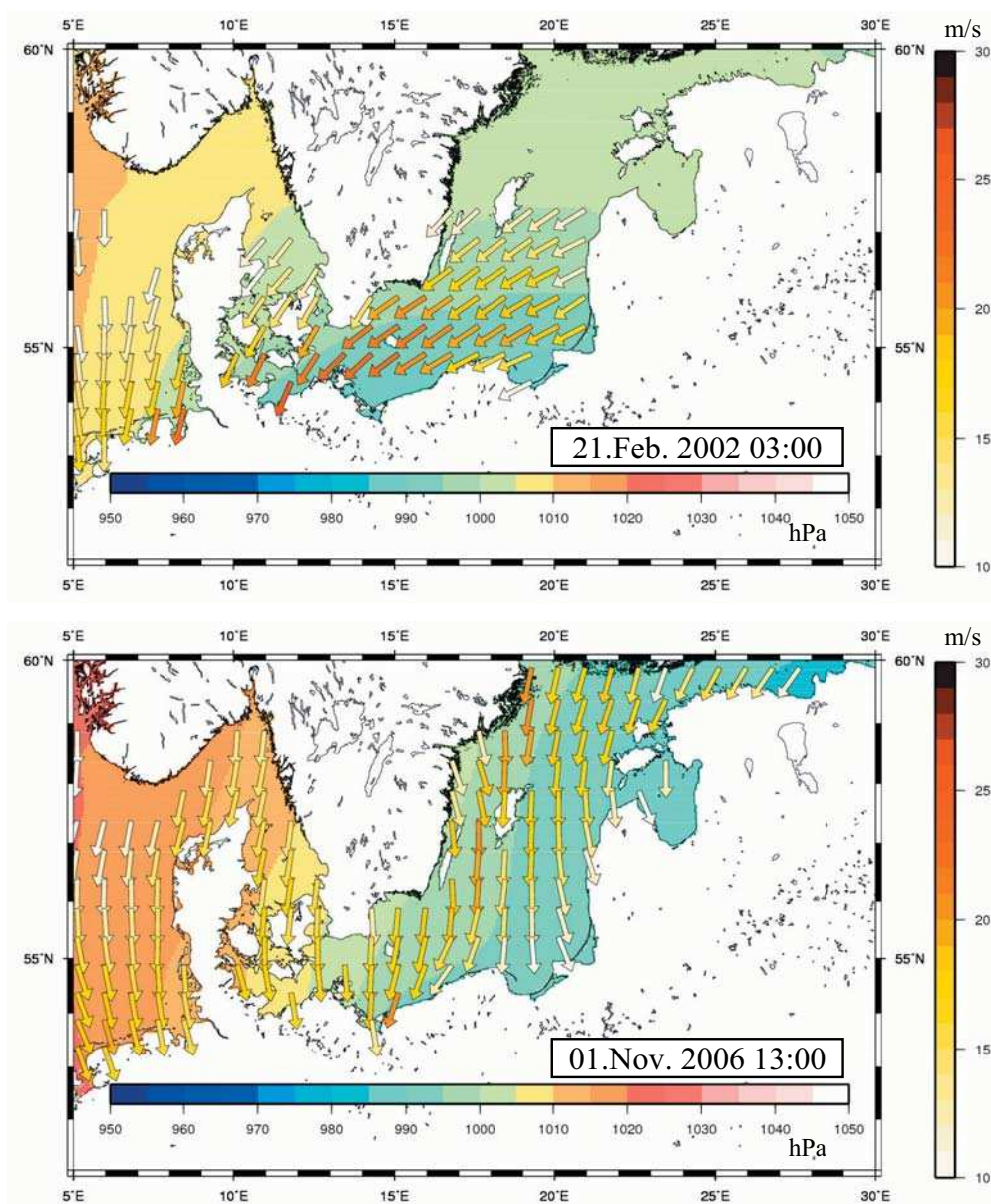
Abb. 5: Windverteilung über der südlichen Ostsee am 21. 2. 2002 um 3 Uhr UTC und am 1. 11. 2006 um 13 Uhr UTC (Windgeschwindigkeiten >10 m/s in jedem 10 Wasserpunkt, im Hintergrund der Bodendruck in hPa)
