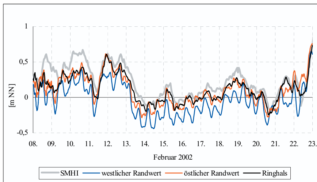
Abb. 12: Pegeldaten Ringhals (SMHI, grau) und Modellergebnisse des BSHcmod in Ringhals (schwarz), sowie Modellergebnisse des BSHcmod am offenen Rand des FTZ-Modells (blau und rot)
