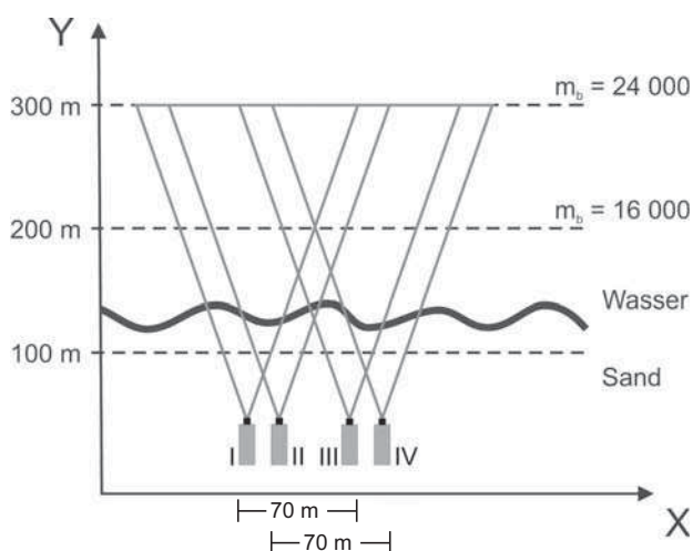
Abb. 7: Aufnahmekonfiguration im Grundriss
