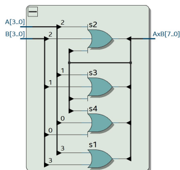
Figura 5. Circuit AM1 part aproximada.
