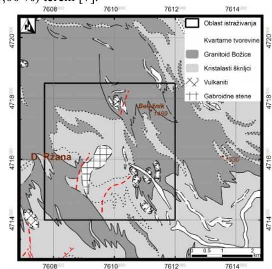
Slika 2 - Geološka karta
