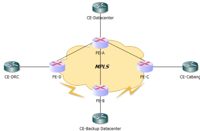
Gambar 4. Desain Konfigurasi Routing OSPF
