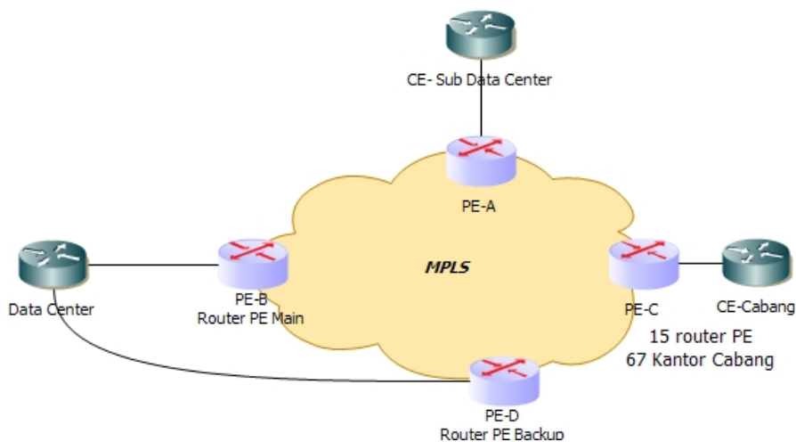
Gambar 3. Konfigurasi Jaringan
