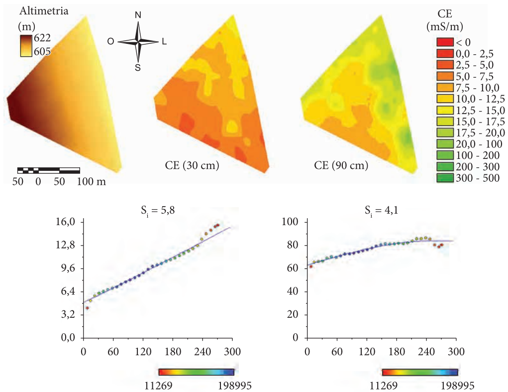
Figura 2. Mapas de altimetria, CEa_{30\ cm} e CEa_{90\ cm} do talhão 49, interpolados por krigagem, para fins da análise dos respectivos variogramas e dos índices de oportunidade ( S_i ) resultantes.
