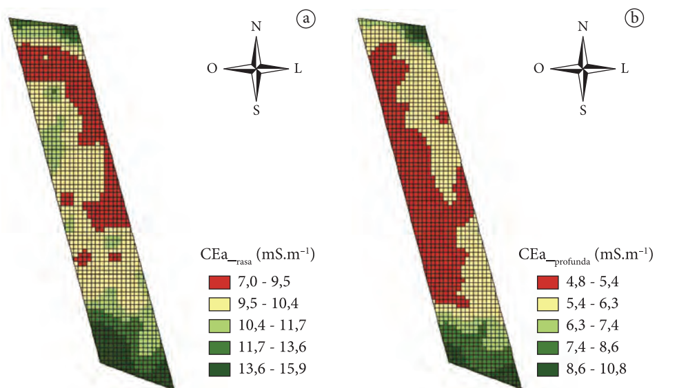
Figura 1. Mapas de superfície da condutividade elétrica aparente do solo (CEa) obtida através do Veris EC 3100 na área experimental de 57,6 ha na Fazenda Pamplona, GO. a) CEa rasa (0-30 cm); b) CEa profunda (0-90 cm).
