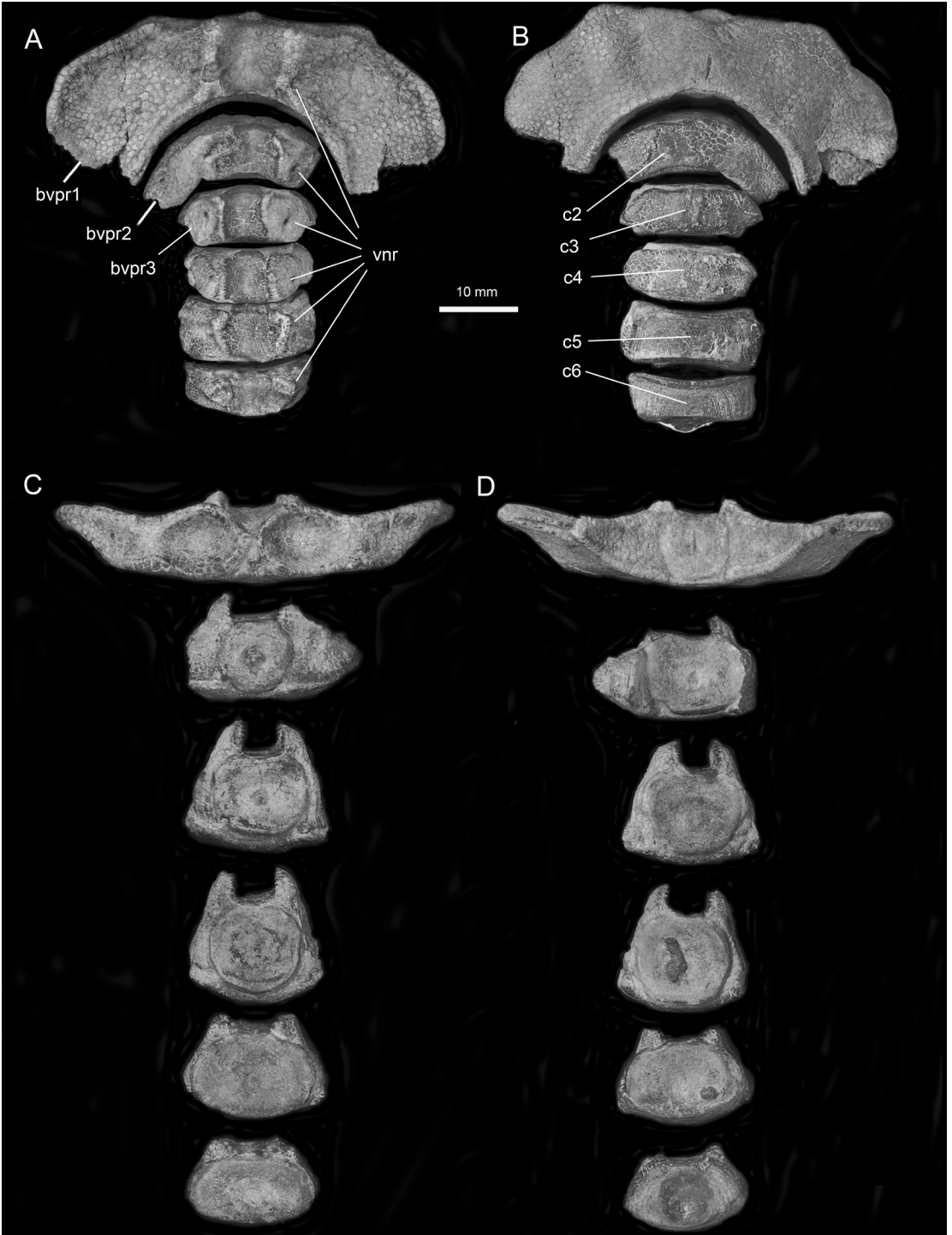
FIG. 2. Cretasquatina americana , gen. nov., sp. nov. Holotype, ALMNH 2792-C, six associated vertebrae forming the anterior vertebral complex: A , dorsal view; B , ventral view; C , anterior views of centra 1–6; D , posterior views of centra 1–6.
