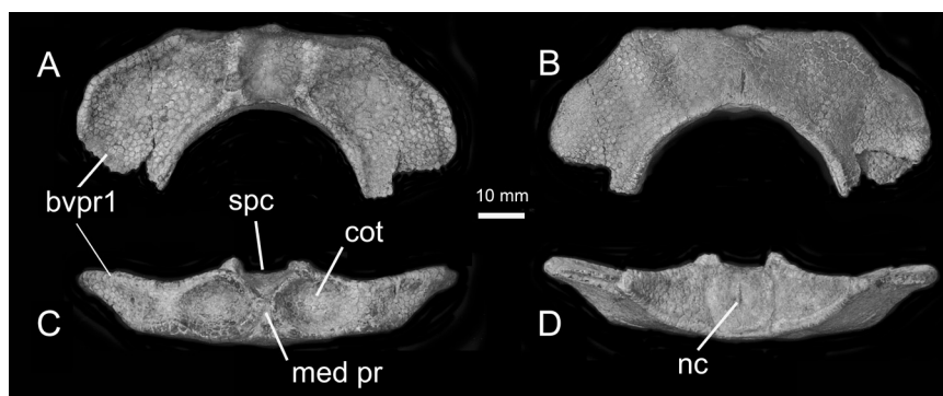
FIG. 3. Cretasquatina americana . Holotype, ALMNH 2792-C, first vertebra: A , dorsal view; B , ventral view; C , anterior view; D , posterior view. Note large size of individual tesserae.
