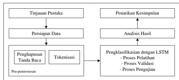
Gambar 1. Metodologi Penelitian
