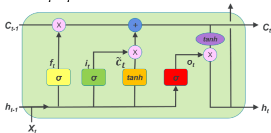
Gambar 2. Arsitektur LSTM
