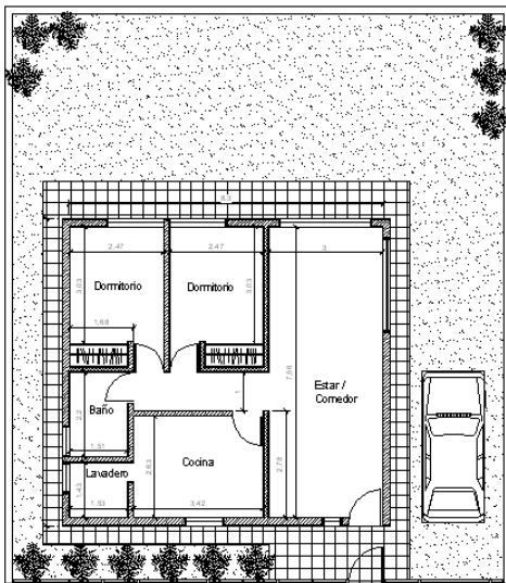
Figura 1: Planta de vivienda tipo “Hogares Casas”
