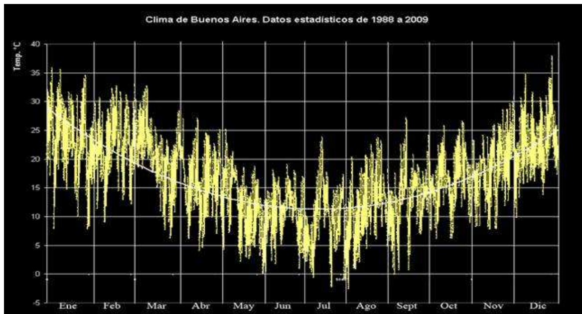
Figura 4: archivo de clima utilizado para la simulación de la vivienda
