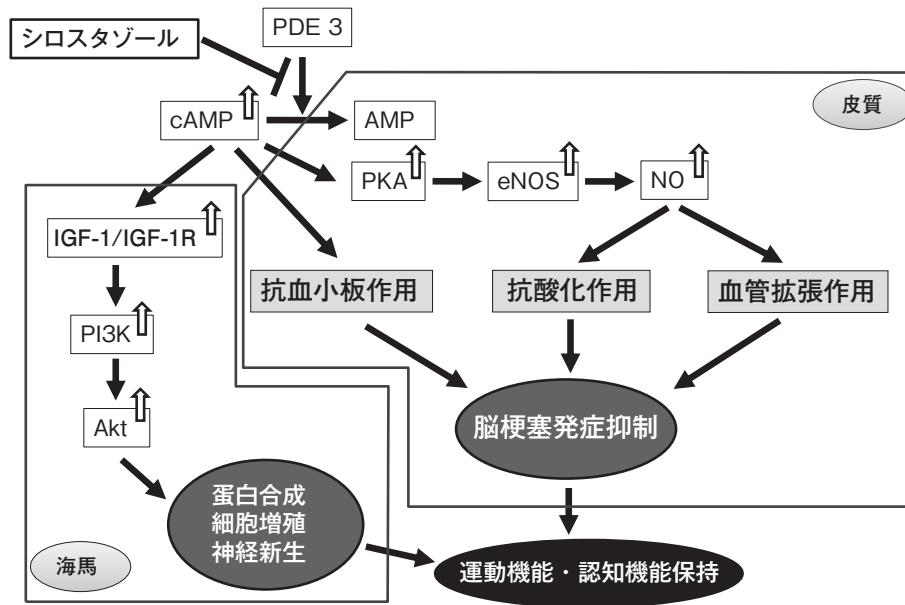
図 シロスタゾールはホスホジエステラーゼ3 (PDE3) を阻害し、細胞内の環状アデノシンーリン酸 (cAMP) 濃度を上昇させ、血管内皮における一酸化窒素合成酵素 (eNOS) 活性を増強し、血管拡張作用や抗酸化作用を発揮する。また、cAMP は IGF/IGF-1R に作用し、プロテインキナーゼA (PKA)、ホスファチジルイノシトール3キナーゼ (PI3K) を介するシグナル伝達経路を活性化させ、蛋白合成や細胞増殖作用を有する。これらの作用により、脳梗塞発症抑制が得られ、運動機能・認知機能が保持されていたと考えられる。 略語：PDE3：ホスホジエステラーゼ3、cAMP：環状アデノシンーリン酸、AMP：アデノシンーリン酸、PKA：プロテインキナーゼA、eNOS：内皮型一酸化窒素合成酵素、NO：一酸化窒素、IGF-1：インスリン様成長因子-1、IGF-1R：インスリン様成長因子-1受容体、PI3K：ホスファチジルイノシトール3キナーゼ
