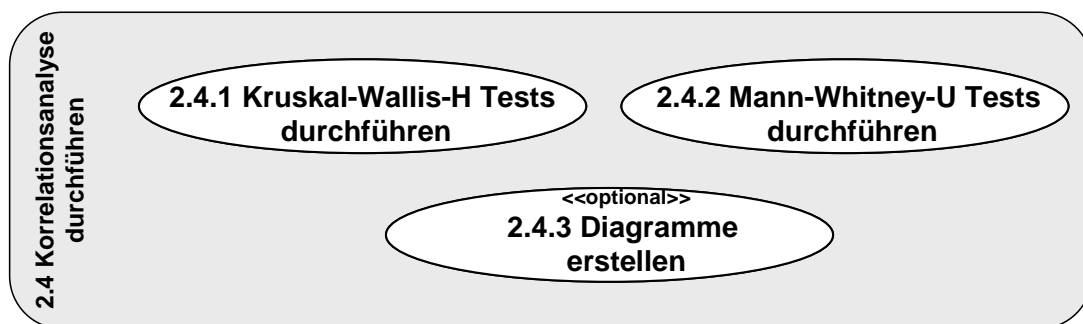
Abbildung 19: Teilschritte zur Durchführung der Korrelationsanalyse
