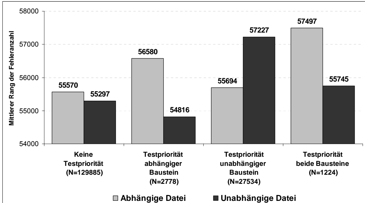
Abbildung 23: Mittlere Ränge (Fehleranzahl) der Abhängigkeiten, eingeteilt nach Testpriorität für Fördergeldverwaltungssoftware Version 18.09.2008
