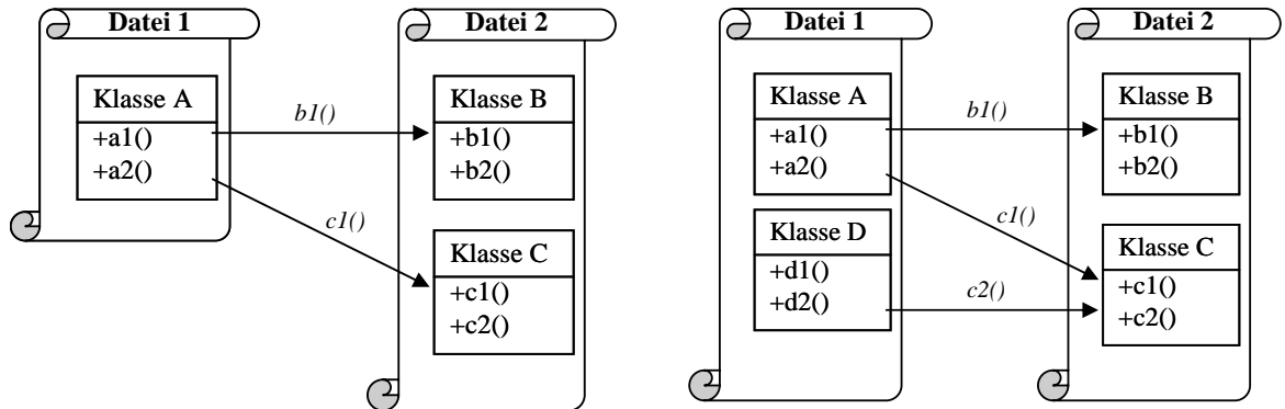
c.) Eine Abhängigkeit mit Aufrufeigenschaften zwischen Datei 1 und Datei 2
