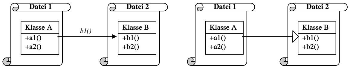
a.) Eine Abhängigkeit mit Aufrufeigenschaften zwischen Datei 1 und Datei 2
