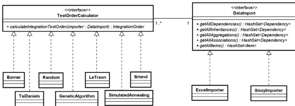
Abbildung 29: Hauptklassen und Schnittstellen von TOC
