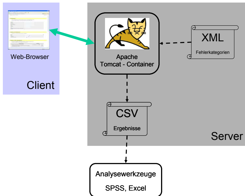
Abbildung 2: Architektur der Onlineumfrage
