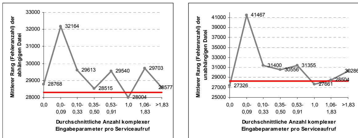
Abbildung 18: Beispiel einer unregelmäßigen Korrelation in Eclipse 2.0
