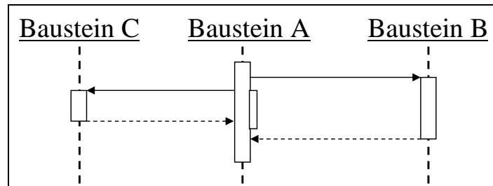
Abbildung 13: Beispiel einer asynchronen Kommunikation
