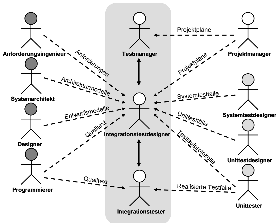
Abbildung 9: Rollen des Integrationstestprozesses und ihre Abhängigkeiten
