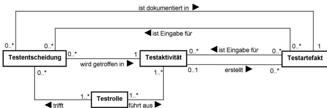
Abbildung 5: Zusammenhänge zwischen Rollen, Artefakten, Aktivitäten, Entscheidungen
