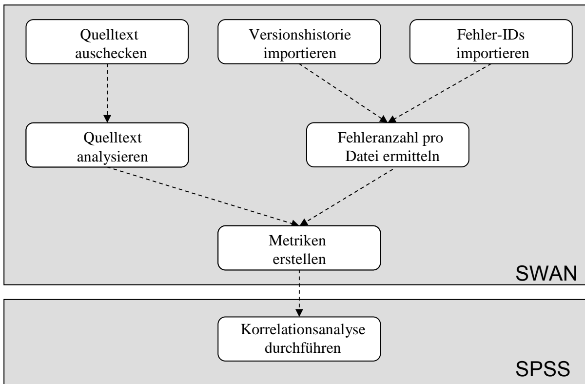
Abbildung 27: Werkzeugunterstützte Teilschritte der Testfokauswahl
