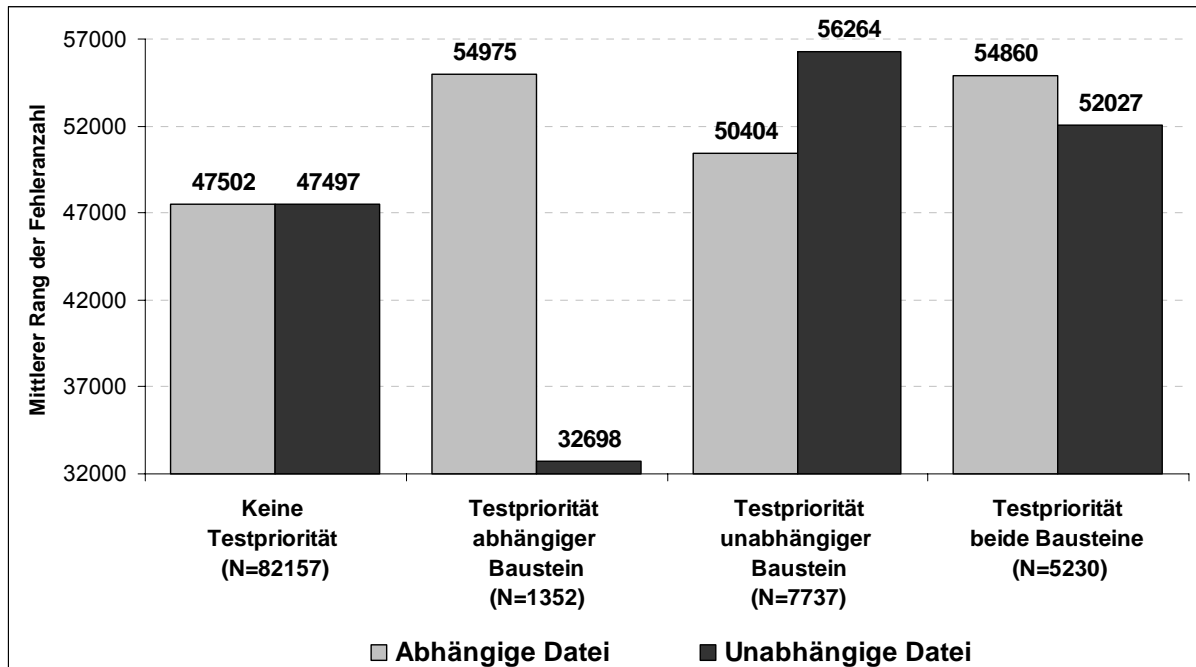
Abbildung 21: Mittlere Ränge (Fehleranzahl) der Abhängigkeiten, eingeteilt nach Testpriorität für Eclipse 3.0
