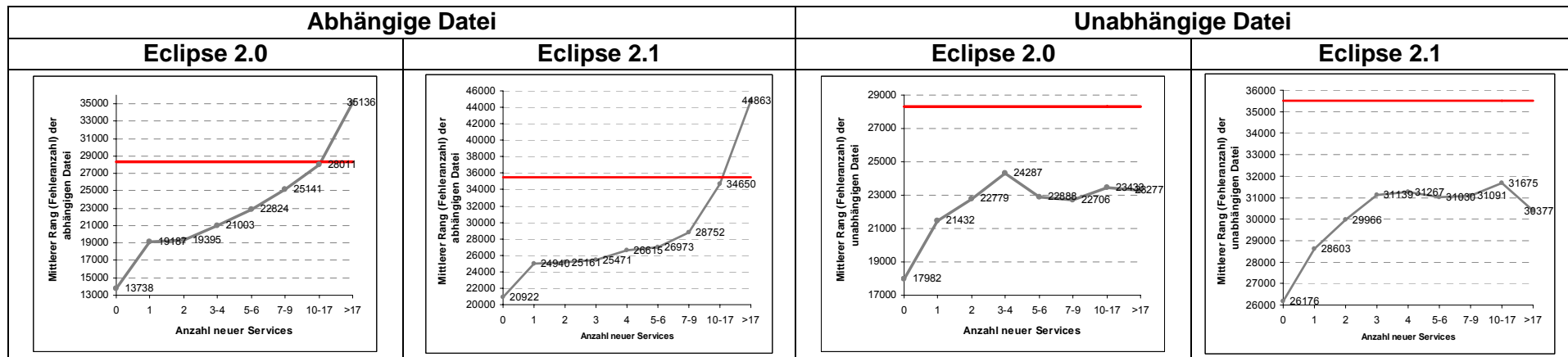
Anzahl neuer Services
