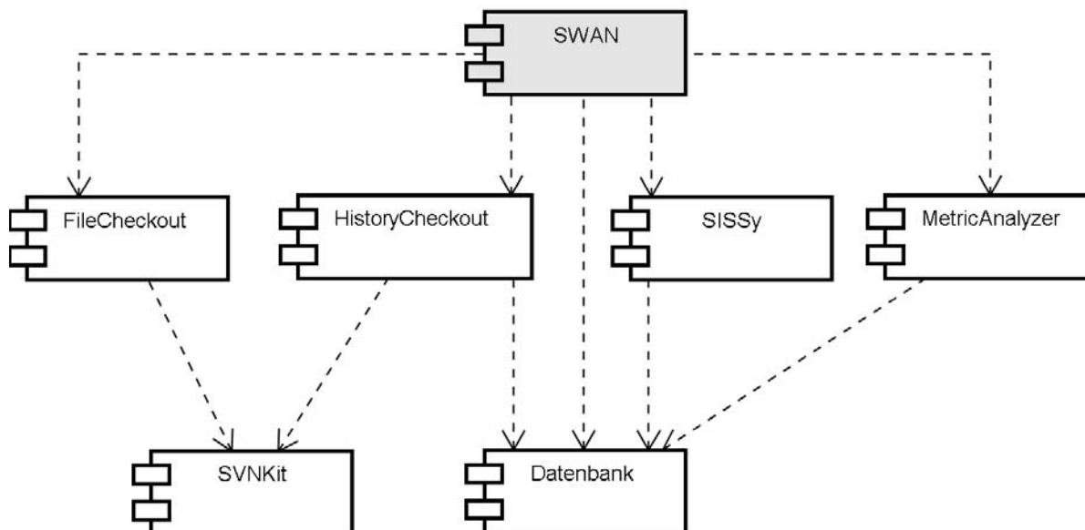
Abbildung 28: Architektur SWAN
