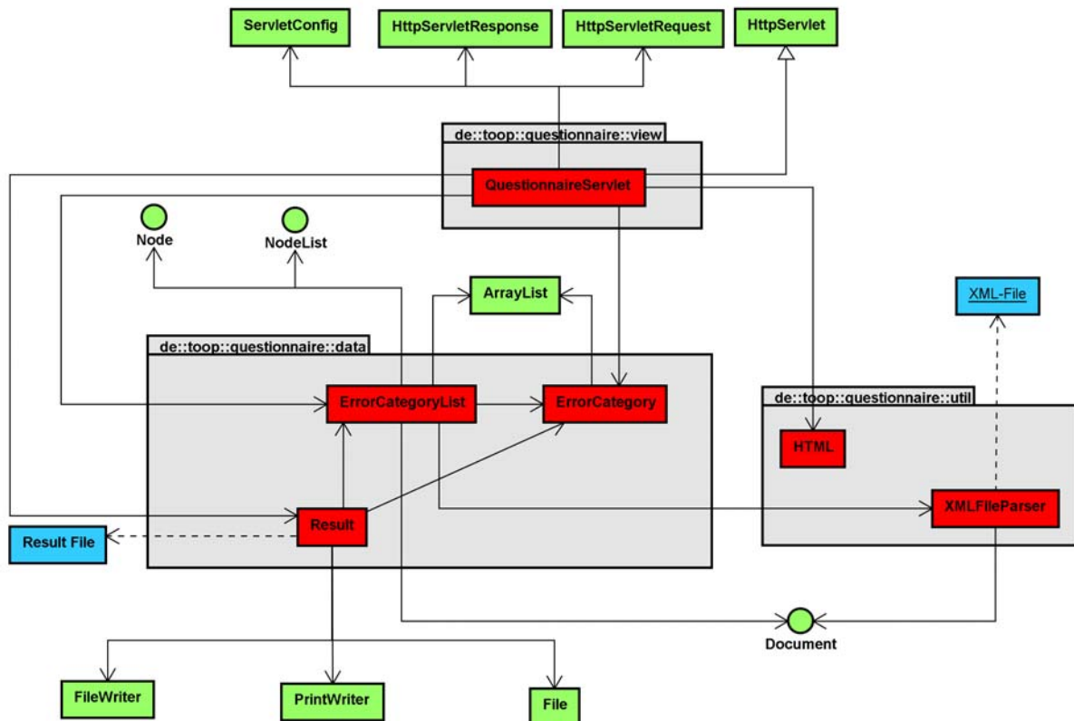
Abbildung 3: Interne Struktur des Onlinefragebogens als Klassendiagramm
