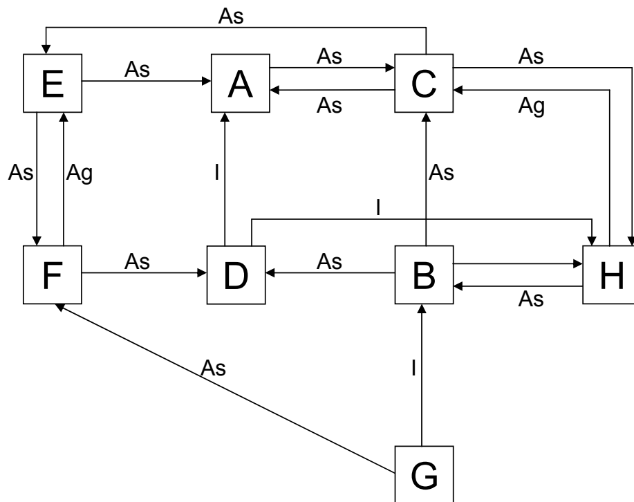
Abbildung 24: Beispielsystem dargestellt als Objektrelationsdiagramm (ORD) nach [BLW01]
