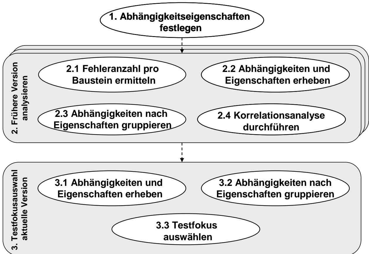
Abbildung 16: Vorgehen zur Testfokusauswahl
