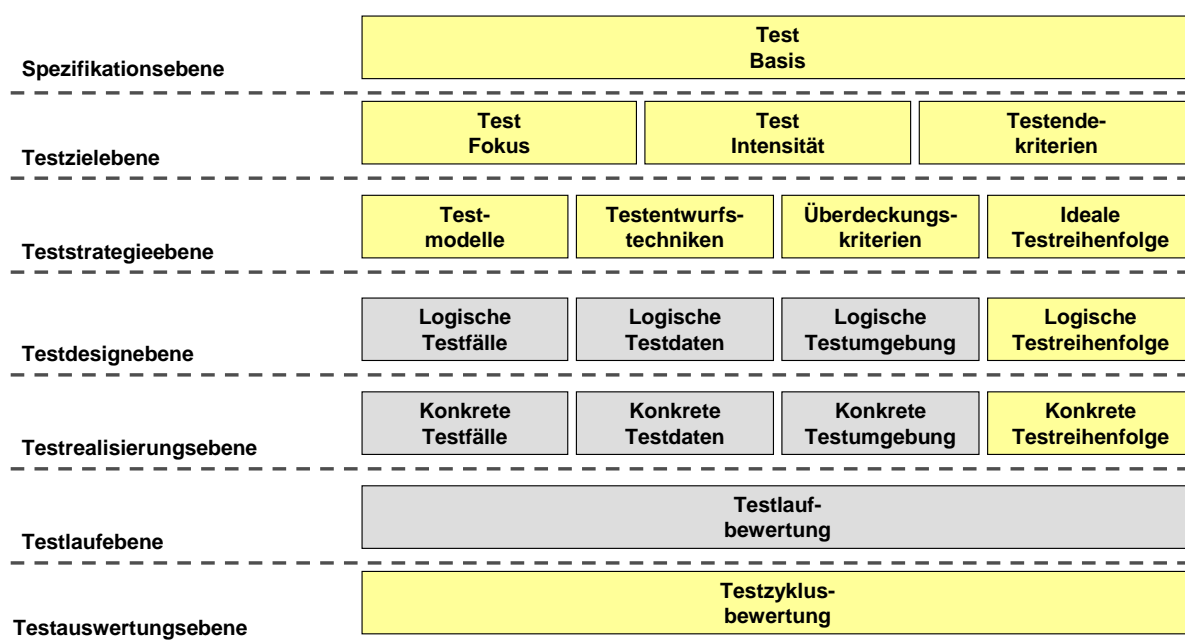
Abbildung 6: Entscheidungshierarchie des generischen Testprozesses
