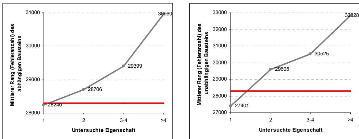
Abbildung 17: Beispiel einer regelmäßigen Korrelation in Eclipse 2.0
