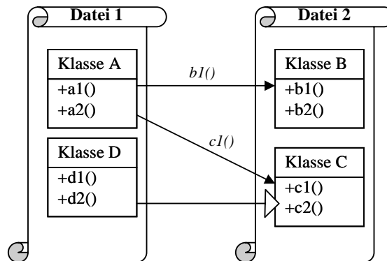
e.) Eine Abhängigkeit mit Aufruf- und Vererbungseigenschaften zwischen Datei 1 und Datei 2
