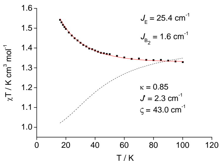
Abbildung 36: cis -Fe[CuL 2 ] 2 ClO 4 : \chi T vs. T-Diagramm experimentelle Daten (■), Simulation (—) mit Modell 2, Simulation unter Annahme eines perfekt oktaedrischen [\text{Fe}^{\text{III}}(\text{CN})_6]^{3-} (---)
