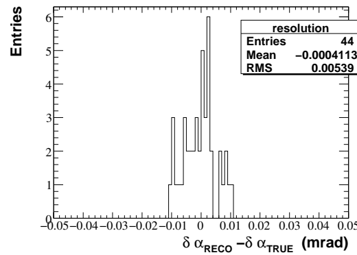
(d) Error plots \delta\alpha
