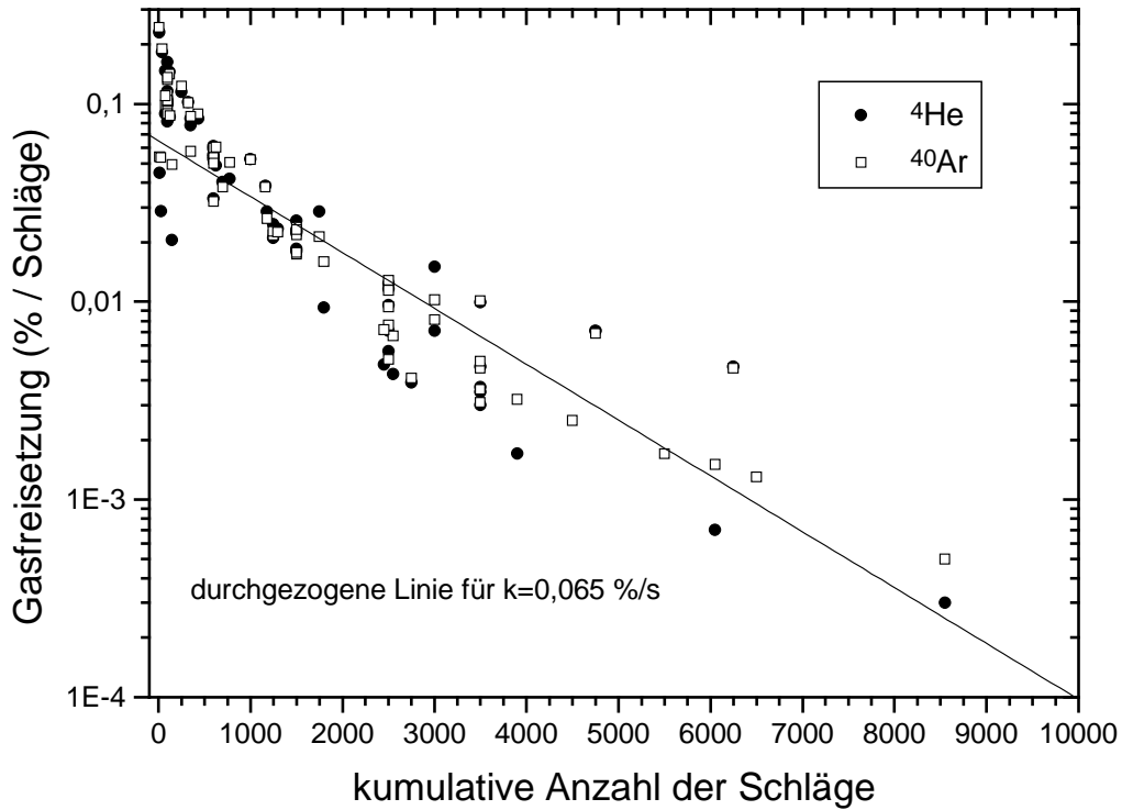
Abbildung 6.2: Normierte Gasfreisetzung von ^4\text{He} (gefüllte Kreise) und ^{40}\text{Ar} (offene Quadrate) versus kumulative Schlagzahl. Es wurde die korrigierte Schlagzahl ( s - s_{\text{EXTR}}/2 ) aufgetragen (siehe Text zur Erläuterung). Linie entspricht Modellkurve mit k=0,065\%/Schlag .
