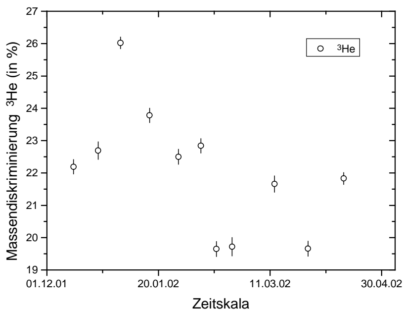
Abbildung A.10: Massendiskriminierung von 3 He nach Installation des neuen He-Eichgases aus Potsdam Ende 2001. Fehlerbalken entsprechen 1 \sigma .
