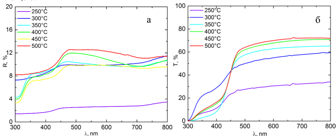
Рис. 1. Спектри відбиття (а) пропускання (б) плівок Zn_xCd_{1-x}S , отриманих при температурах підкладки T_s = (523-773) К
