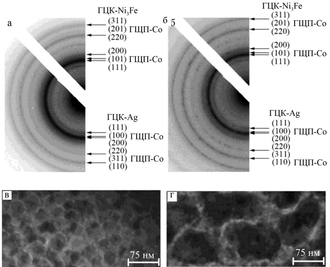
Рисунок 3.4 – Дифракційні картини (а, б) та кристалічна структура (в, г) для тришарової псевдоспін-вентельної структури \text{Ru}(5) / \text{Ag}(9) / \text{Co}(30) / \text{П} після конденсації та (а, в) та відпалювання до 750 К (б, г)
