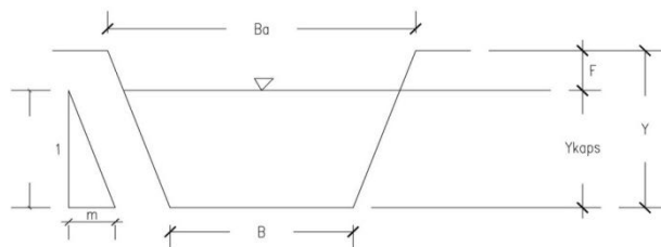
Gambar 1. Saluran berbentuk trapesium Sumber : Triatmodjo, 2008
