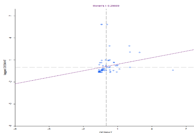
Figura 3. Diagrama I de Moran - grau de autocorrelação espacial do desmatamento em Mato Grosso do Sul. Fonte: Resultados da pesquisa.
