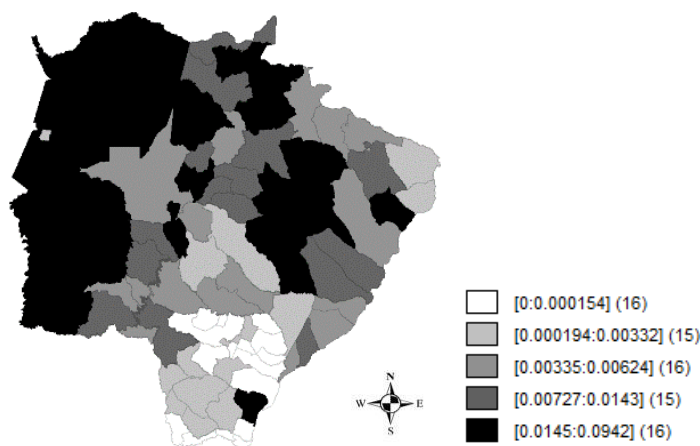
Figura 2. Superfície de desmatamento (km 2 ) por cidade em Mato Grosso do Sul em 2008. Fonte: Resultados da pesquisa.
