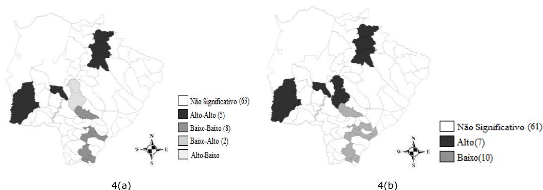
Figura 4. Mapa de cluster de I de Moran - 4(a) e mapa de cluster da estatística G de Getis-Ord - 4(b). Fonte: Resultados de pesquisa.
