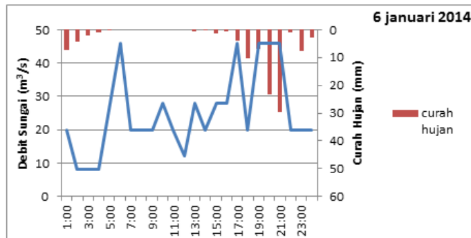
Gambar 6. Debit sungai Way Besai dan curah hujan di Suoh per jam tanggal 6 Januari 2014
